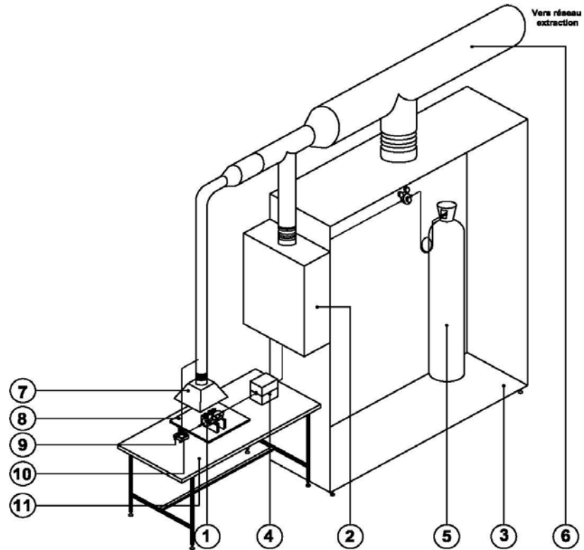
Figure 1 Schéma global du banc de mesure, vue physique des composants
