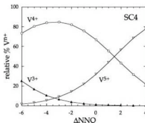
Figure D.4: Variations théoriques des proportions relatives des différents degrés d'oxydation du vanadium ( V^{n+} ) en fonction de la fugacité en oxygène pour un liquide ferrobasaltique, appelé SC4. Les conditions en fugacité en oxygène correspondant aux systèmes terrestres basaltiques varient de \Delta NNO = -3 à \Delta NNO = +1 , où \Delta NNO représente les conditions en oxygène par rapport au tampon NNO (Nickel-Nickel Oxide). La figure provient de la Ref. [206].
