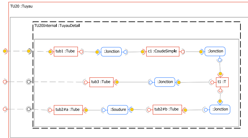
Figure 5.13 – Résultat du tronçonnage du tube tub2 .
