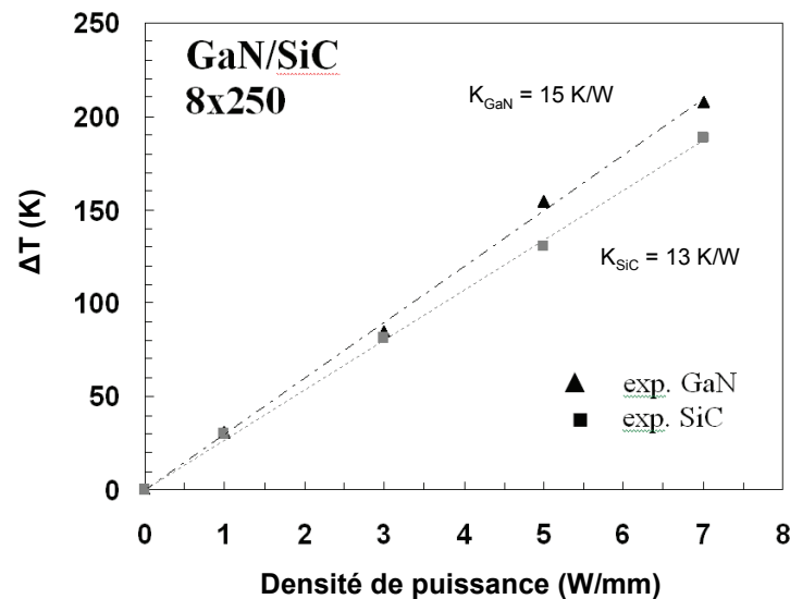
Figure 3-36 : Evolution de la température des couches de GaN et de SiC en fonction de la densité de puissance du HEMT AlGaIn/GaN 8 doigts.
