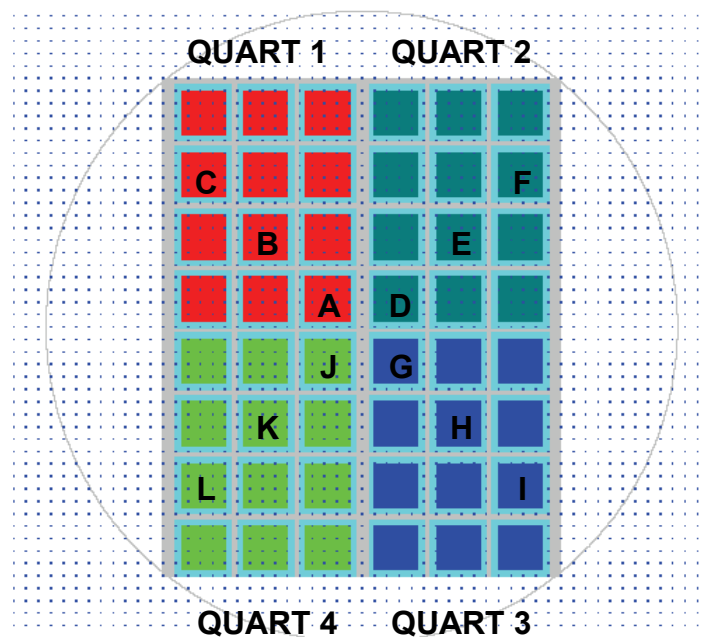
Figure 2-23 : Schéma du wafer étudié.
