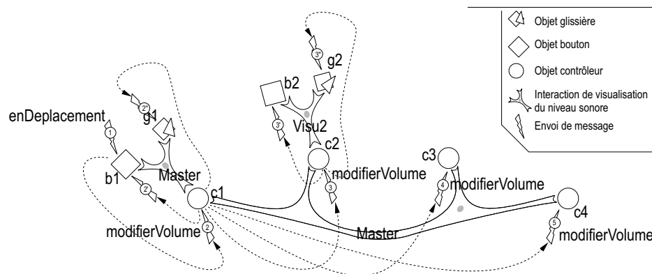
FIG. 8.6 – Graphe de propagation des comportements réactifs
