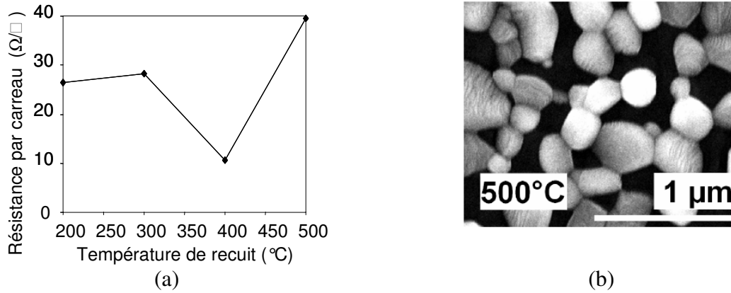
Fig. 96 : Resistance de couche (a) des échantillons Pt(20nm)/Ge(1.5 \mu\text{m} )/Si recuit à différentes températures, et observation MEB en vue de dessus de l'échantillon recuit à 500°C (b).
