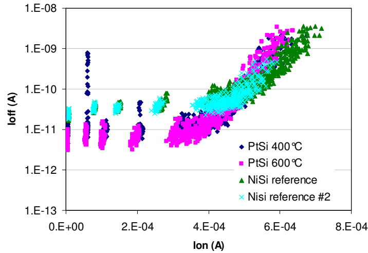
Fig. 135 : Graphique I_{off} - I_{on} des transistors NMOS pour les plaques PtSi 400°C, PtSi 600°C, et pour la référence NiSi.
