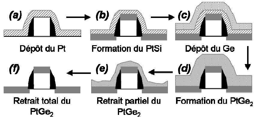
Fig. 91 : Schéma d'intégration alternatif utilisant un procédé de retrait sélectif du métal non réagi (ici le platine) par germaniuration sacrificielle
