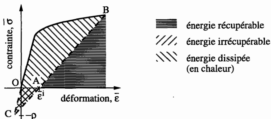
FIG. 1.5 - Bilan énergétique pour un composite endommageable avec contraintes résiduelles initiales.
