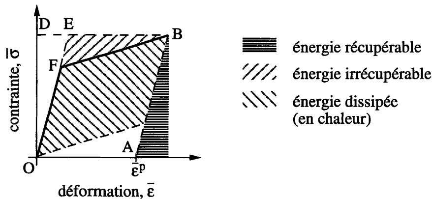
FIG. 1.3 - Bilan énergétique pour un matériau à écrouissage cinématique linéaire.
