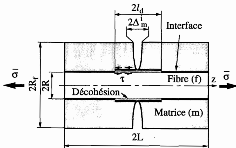
FIG. 1.6 - Cellule élémentaire d'un composite subissant de la décohérence et du frottement.
