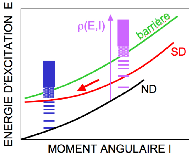
Figure 1.6: Dessin qui illustre de façon schématique comment varie en fonction du moment angulaire I (i) l'énergie d'excitation E des états superdéformés par rapport aux états normalement déformés de même spin (ii) la hauteur de la barrière de potentiel séparant le puits normalement déformé et le puits superdéformé et (iii) la densité d'états normalement déformés à l'énergie d'excitation des états superdéformés.
