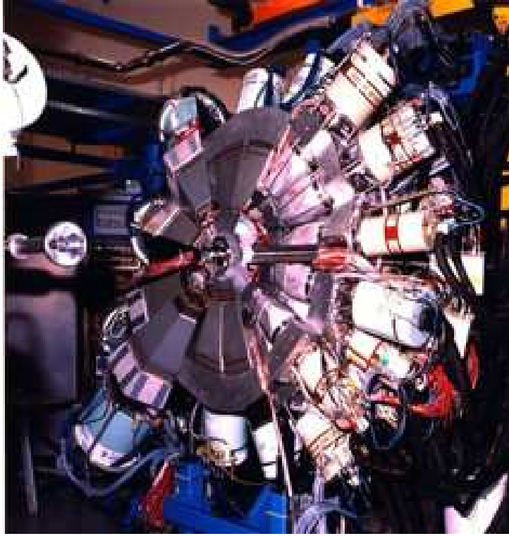
Figure 1.4: Demi-sphère du multidétecteur EUROBALL IV installé à l'IREs.
