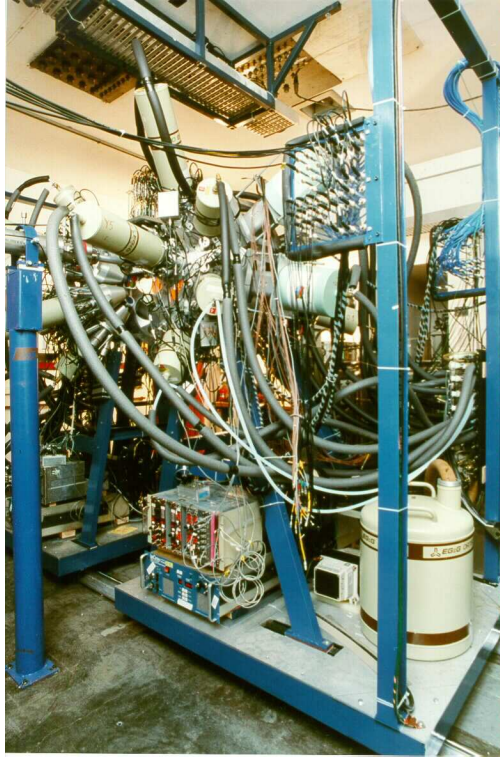
Figure 1.7: Multidétecteur Yrastball installé auprès du tandem de l'Université de Yale.
