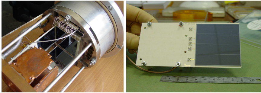
Figure 3.6: Photographie de la mécanique de soutien des détecteurs au silicium utilisés au plan focal de VASSILISSA. Sont visibles le détecteur d'implantation et deux faces du tunnel pour la détection des particules \alpha échappées ainsi que les électrons de conversion interne. A droite: Photographie d'un des 4 détecteurs d'électrons.
