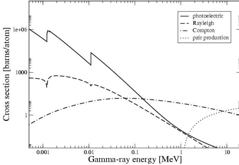
Figure 4.3: Section efficace d'interaction de photons dans du Germanium en fonction de l'énergie incidente des photons.
