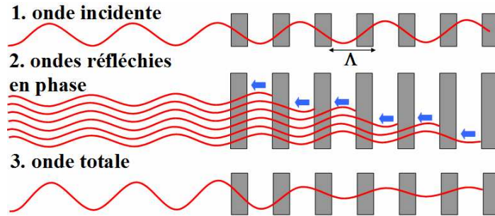
Figure III.A-3 : principe de fonctionnement d'un réseau de Bragg
