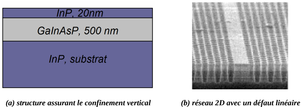
Figure I.A-1 : guide en cristal photonique [1]. Le confinement est assuré verticalement par l'épitaxie (a) et horizontalement par le cristal photonique (b)
