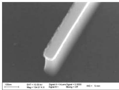
(a) extrémité d'un taper, largeur 80 nm
