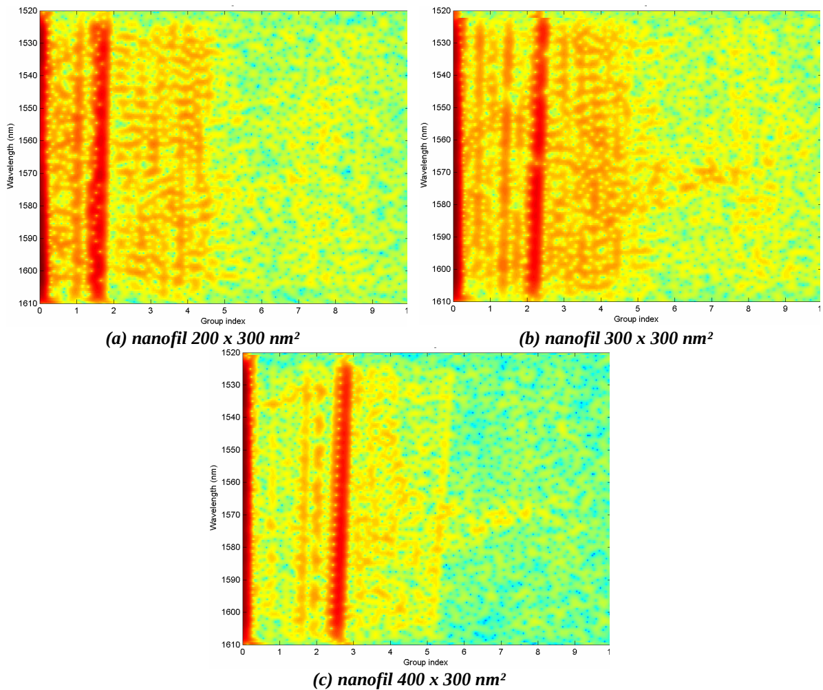
Figure II.C-7 : réflectogrammes obtenus en TM pour des nanofils d'InP dans le BCB de 300 nm de haut et de 200 (a) 300 (b) et 400 nm de larges reportés sans titane
