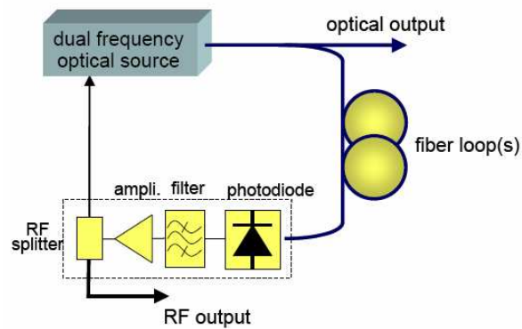
Figure III.A-1 : schéma d'un oscillateur optoélectronique [1]
