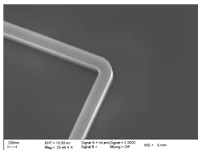
(c) coude à 90° sur un guide de 300 nm
