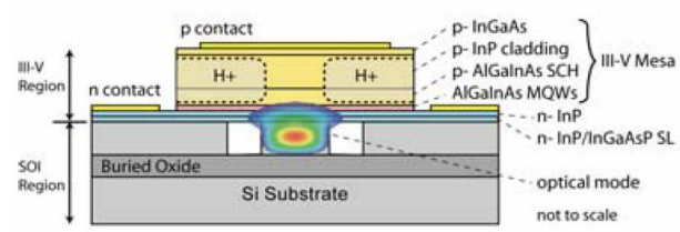
(b) laser à puits quantique AlGaInAs reporté sur un guide SOI ( 0,76 \times 2 \mu\text{m}^2 ) [15]
