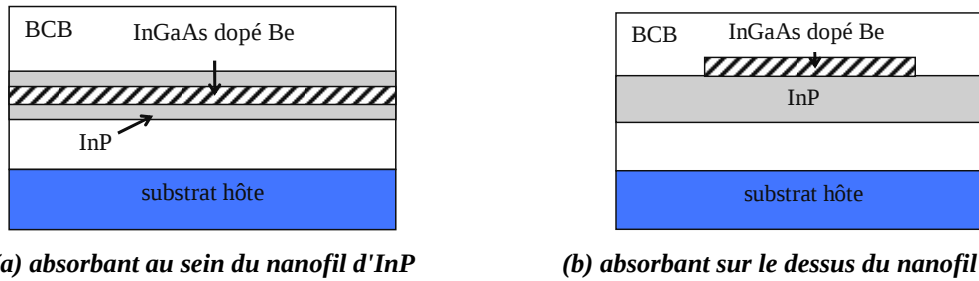
Figure IV.B-1 : schéma des structures proposées pour la réalisation d'un interrupteur optique sur nanofil d'InP dans le BCB
