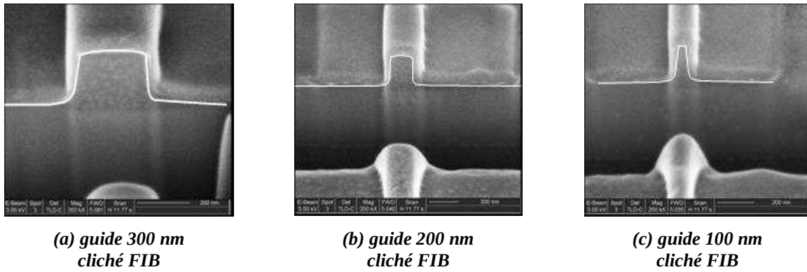
Figure I.B-12 : observation au FIB de la gravure \text{CH}_4(10\text{sccm})/\text{H}_2(80\text{sccm})/\text{Ar}(10\text{sccm}) , 250W, 35 mTorr réalisée à l'aide du nouveau bâti Plasmalab 80+
