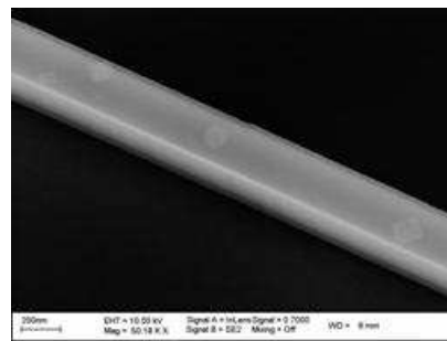
(b) guide de 300 nm
