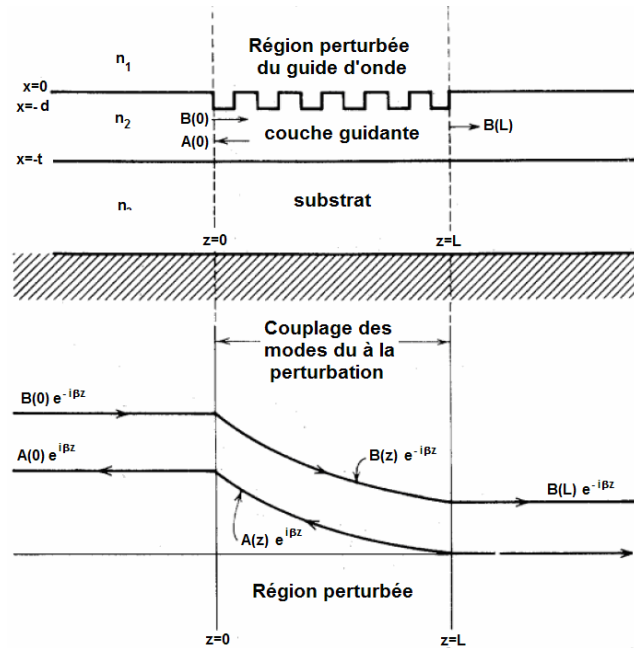
Figure B-1: section perturbée du guide d'onde considéré (haut) et évolution des enveloppes des champs incident (B) et réfléchi (A) (bas)
