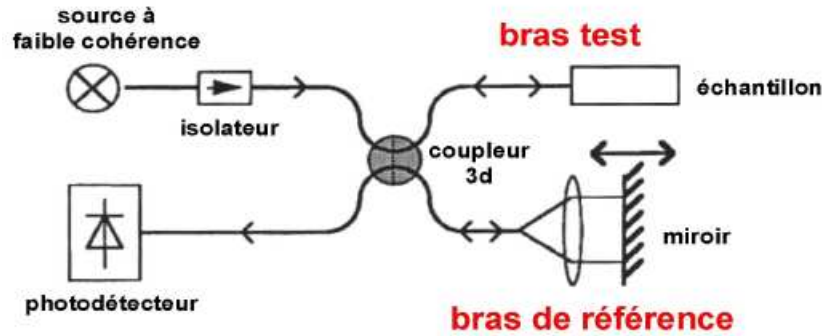
Figure II.C-4 : schéma simplifié d'un système de caractérisation OLCR
