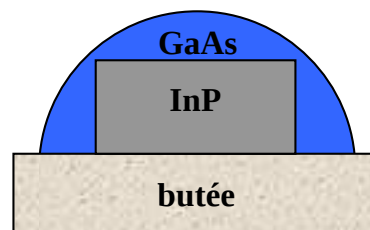
Figure I.B-16 : principe de l'alignement manuel des substrats, vue de dessus
