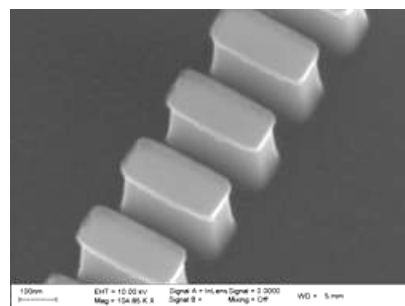
(d) réseau de Bragg, pas 240 nm
