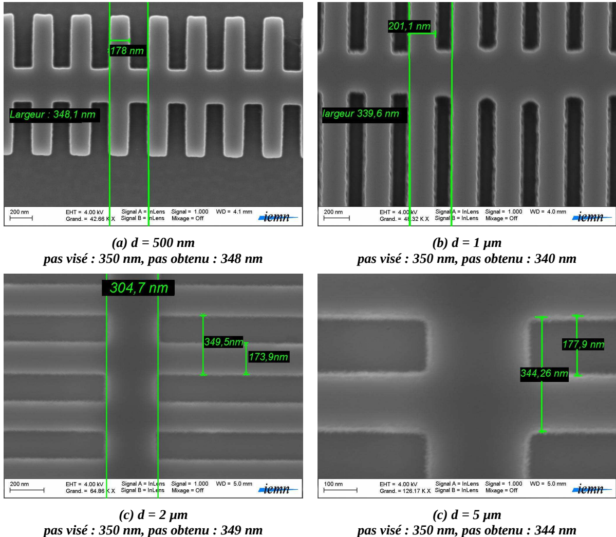
Figure III.B-10 : masque de gravure en HSQ des réseaux de Bragg pour la polarisation TM
