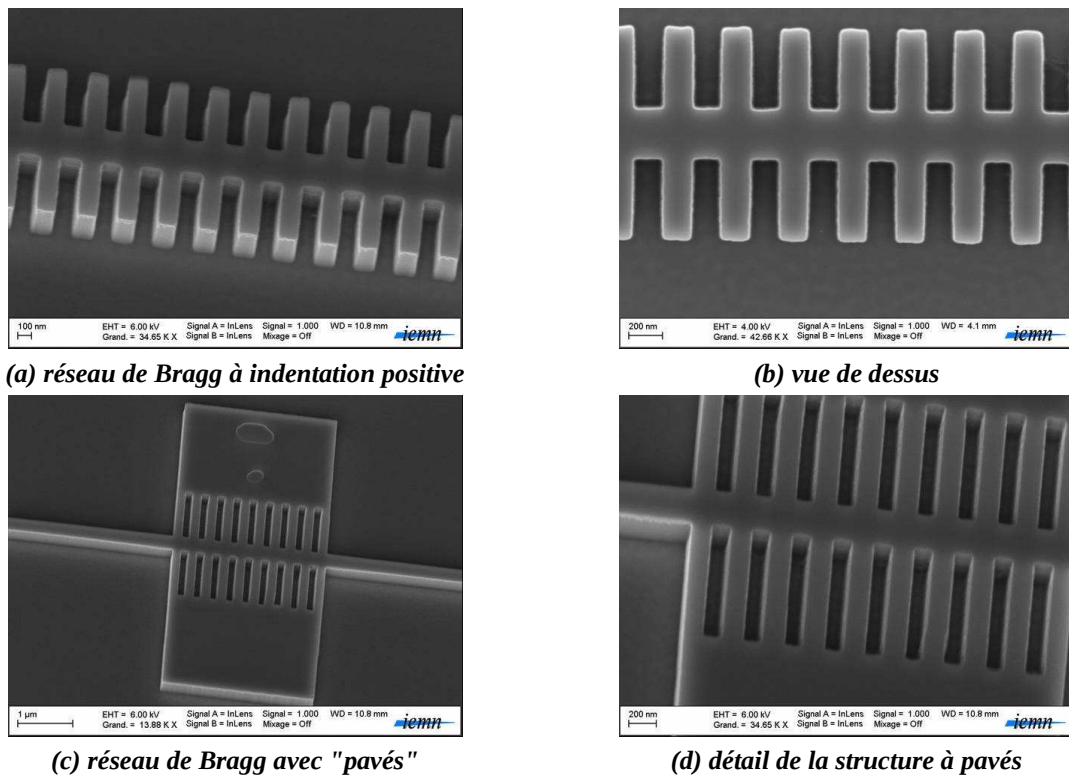
Figure III.B-9 : exemples de réseaux de Bragg sur nanofils d'InP avant leur report dans le BCB ( d = 500 nm, \Lambda = 350 nm)
