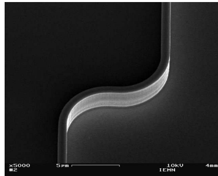
Figure I.A-5 : guides de 0,8 \mu\text{m} de large présentant des coudes de 5 \mu\text{m} de rayon ; profondeur de gravure : 2,7 \mu\text{m} [6]
