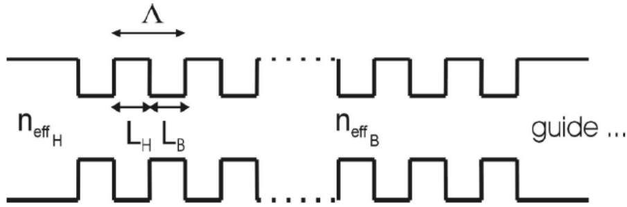
Figure III.A-2 : schéma d'un réseau vertical
