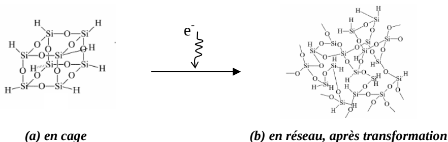
Figure I.B-2 : structure de la HSQ [29]
