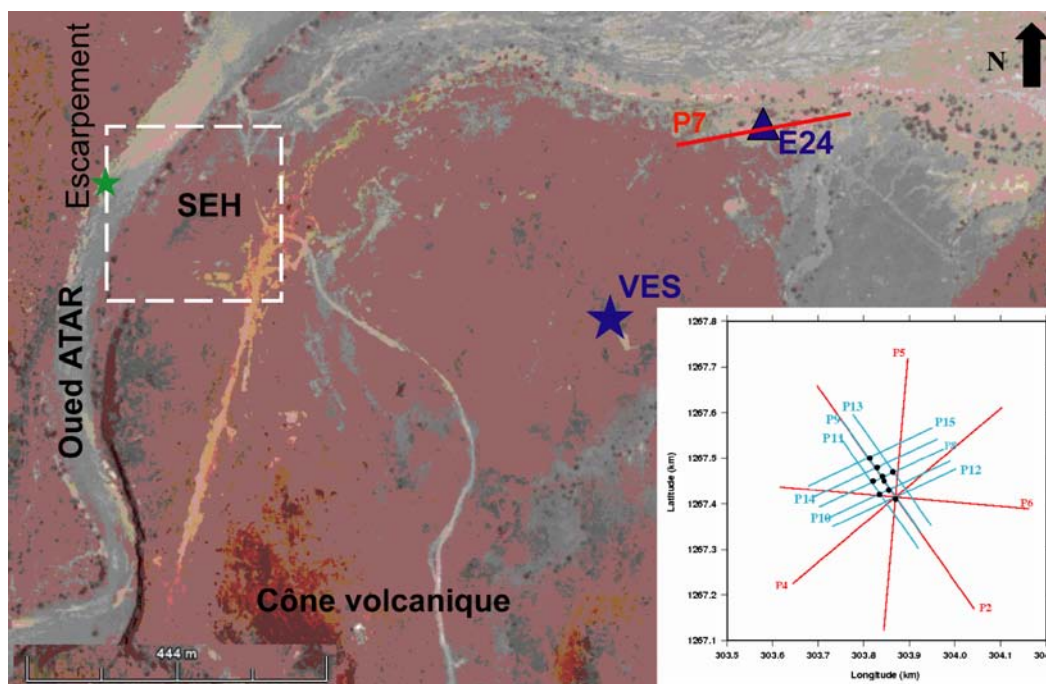
FIG. 5.6: Carte de localisation du site expérimental hydrogéologique (cadre blanc en pointillé) et les différents panneaux électriques réalisés sur celui-ci (encart) et à son voisinage. Un long panneau électrique (P7 en trait rouge) a été réalisé à l'emplacement de l'ancien forage E24 (triangle bleu). Un sondage électrique (étoile bleue) avait été réalisé lors de la campagne CGG(1987). Encart : les profils réalisés sur le SEH, avec en rouge les panneaux longs (pas=10m) et en bleu les panneaux courts (pas=5m). Les points noirs représentent les positions des forages et des piézomètres. Cette carte de localisation du site est tirée de Google Earth.
