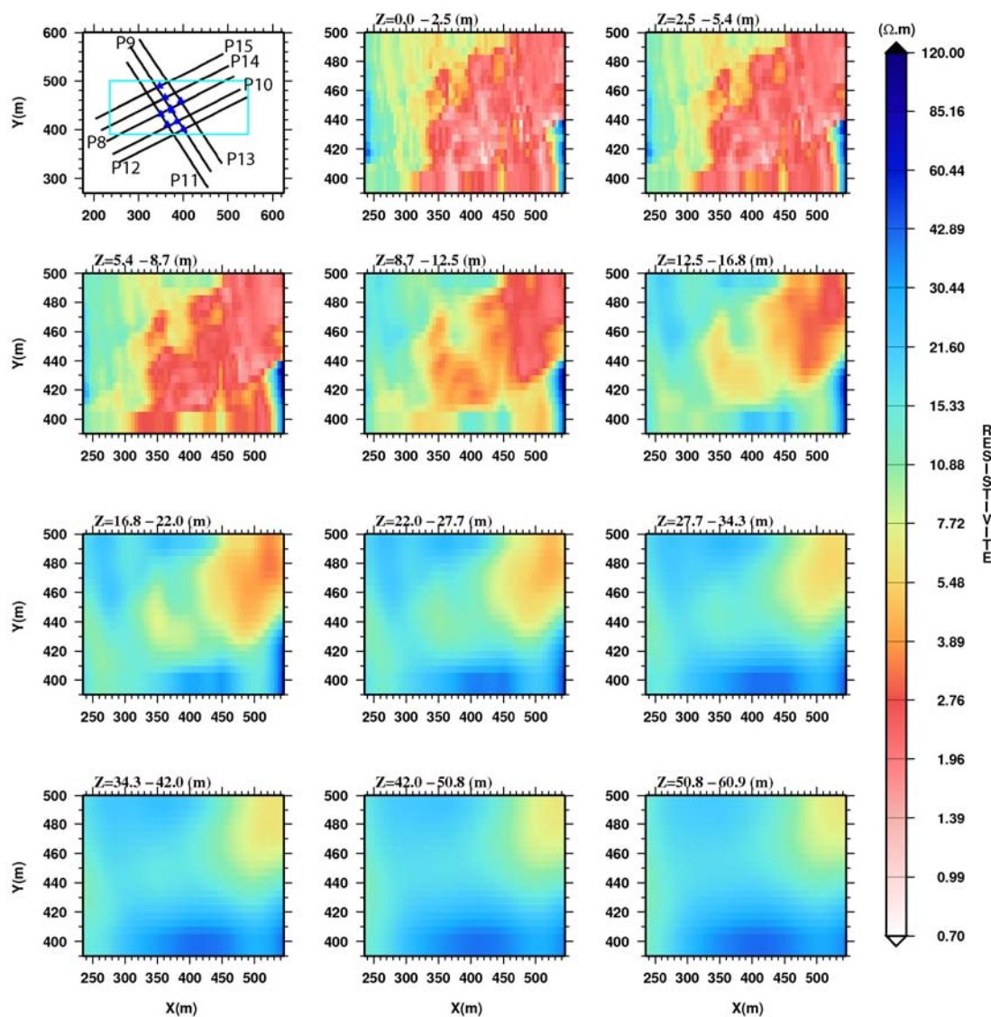
FIG. 5.31: Résultat de l'inversion 3D obtenue à partir des panneaux qui ont un espacement entre électrodes de 5 m et une carte qui montre les panneaux considérés et les positions des forages. Le cadre bleu correspond à la taille du modèle inversé.
