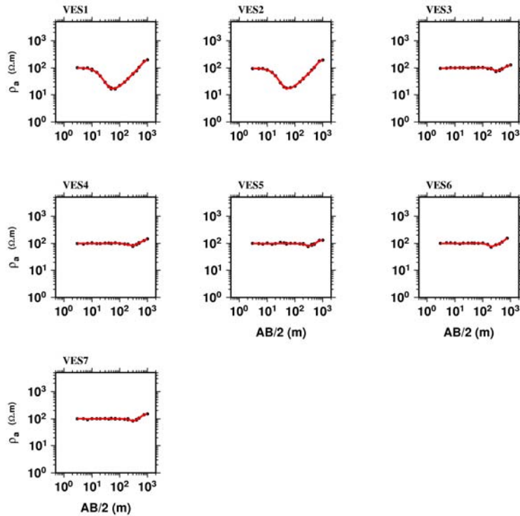
FIG. 3.12: Réponse du modèle de résistivité obtenu avec les données simulées à partir du troisième modèle synthétique (Exemple 3). Les points noirs représentent les données et les courbes rouges sont la réponse du modèle pour chaque sondage.
