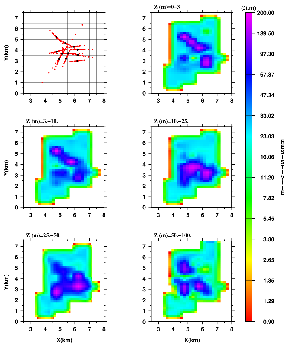
FIG. 4.17: Résultat de l'inversion 3D des 11 VES en utilisant un modèle à priori homogène de résistivité 70 Ohm.m (résistivité moyenne des données). La première section horizontale représente la zone d'étude avec les sondages électriques considérés. Points noirs : Centre de chaque dispositif (VES). Points rouges : Azimuts de chaque VES (ou positions des électrodes).
