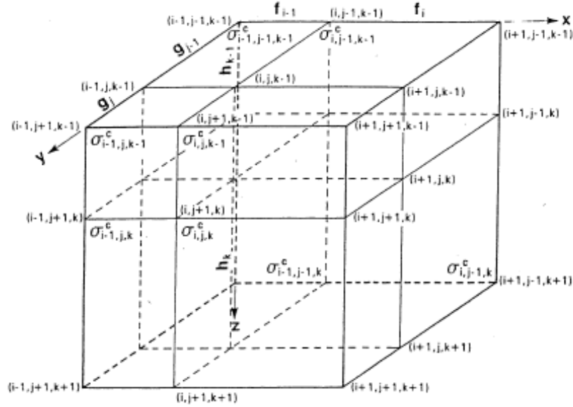
FIG. 3.1: Grille définie pour le programme de calcul direct 3D indiquant le dimensionnement des mailles ( f, g, h ) et la conductivité des cellules ( \sigma^c ). Les variables i, j, k représentent les indices des noeuds de la grille dans les 3 directions (D'après Spitzer, 1995).
