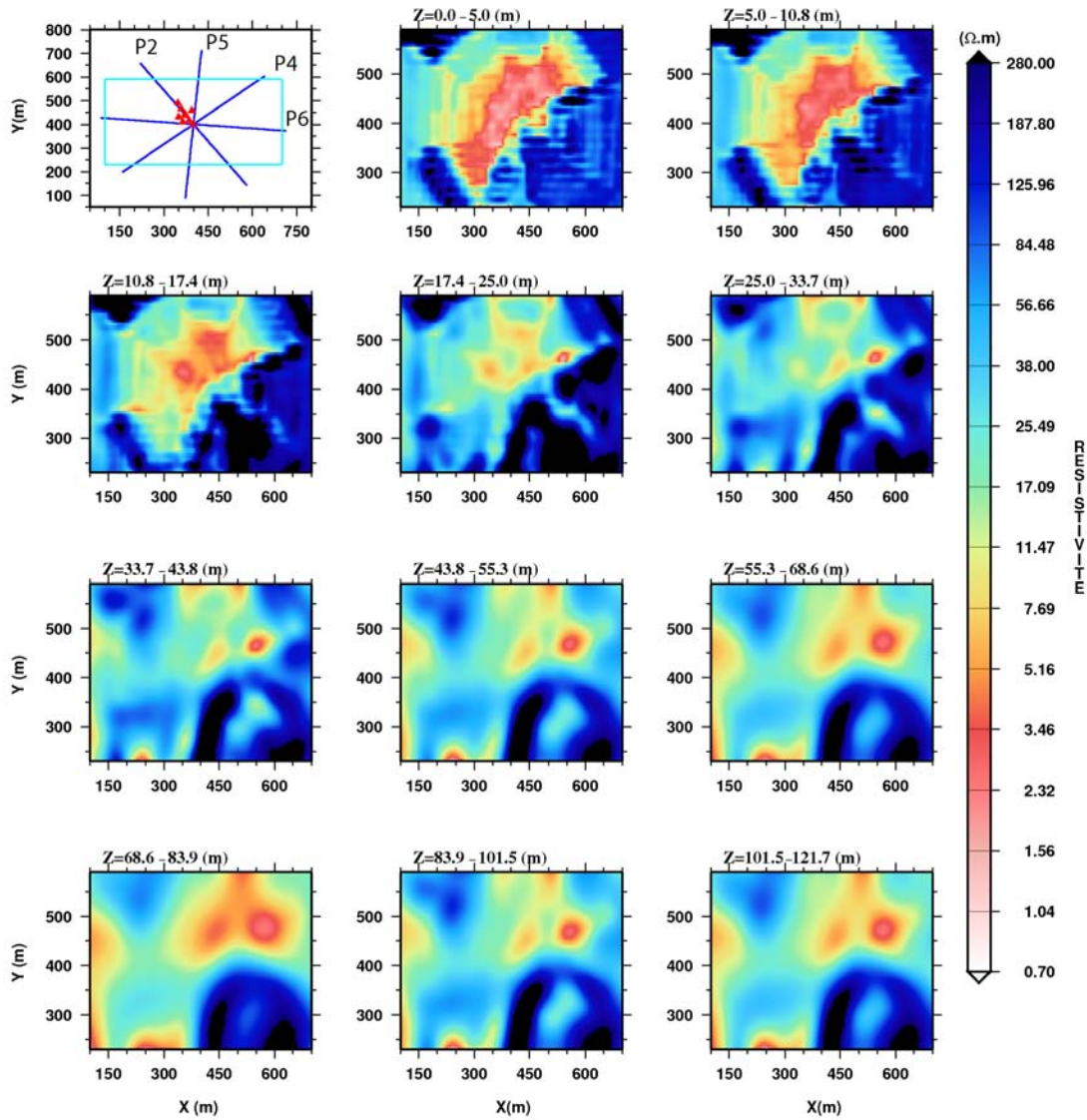
FIG. 5.26: Résultat de l'inversion 3D obtenue à partir des panneaux avec un espacement de 10 m. En haut à gauche : carte qui montre les panneaux considérés à l'origine (avant interpolation) et les positions des forages. Le cadre bleu correspond à la surface du modèle considéré pour l'inversion 3D.
