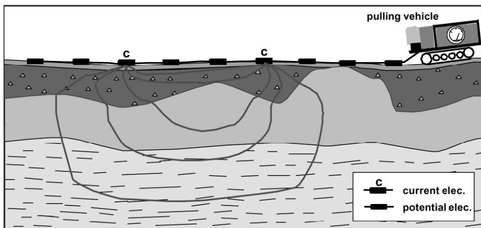
FIG. 1.6: Panneau électrique mobile de type PACES.(selon Christiansen, 1998)
