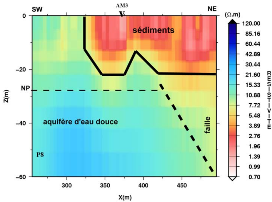
FIG. 5.40: Section verticale extraite du modèle 3D selon la direction du panneau P8 avec les interprétations géologiques.
