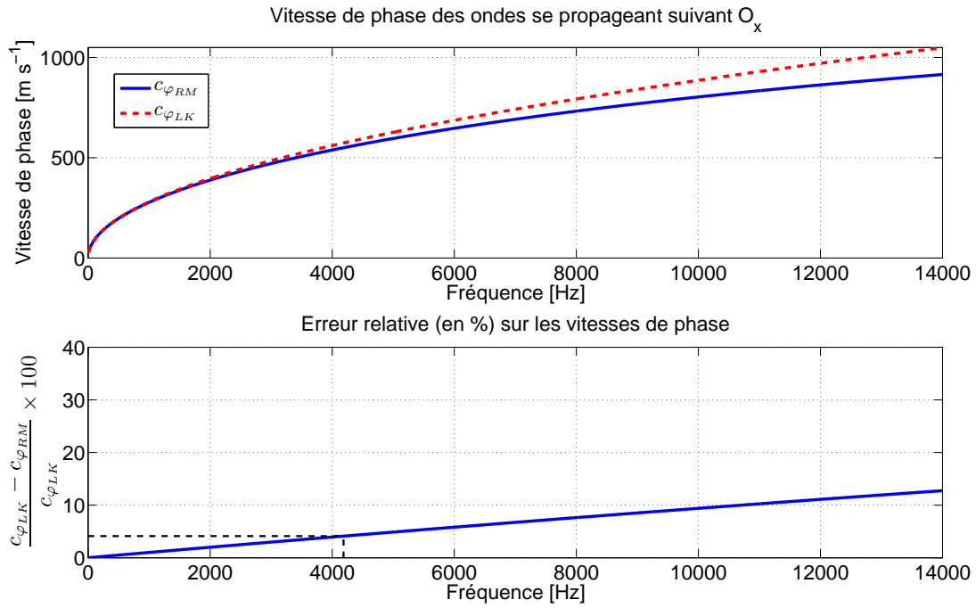
FIG. A.3 – Influence du cisaillement et de l’inertie de rotation pour des ondes de flexion se propageant dans la direction longitudinale d’une plaque en épicéa de 8 mm taillée dans le plan LR. À 4200 Hz, l’erreur sur la vitesse de phase est d’environ 4%.
