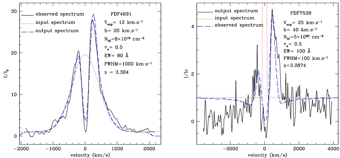
FIG. 3.3: Objets avec une raie Ly \alpha symétrique. L'ajustement de ces deux profils est réalisé avec une coquille quasi-statique ( v_{exp} = 10 - 25 km s ^{-1} ) et le reste des paramètres est donné dans la légende. On peut difficilement reproduire l'extension des ailes des pics de FDF4691 sans recourir à raie Ly \alpha intrinsèque anormalement large ( FWHM = 1000 km s ^{-1} ) pour un starburst. Ce pourrait être le seul objet de notre échantillon dont l'émission Ly \alpha serait le résultat d'une excitation par un AGN.
