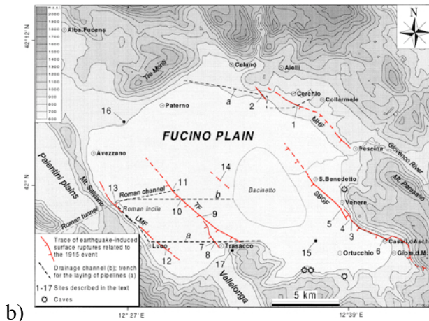
FIG. 3.16 : Evolution du bassin du Fucino. a) Représentation schématique de l'évolution temporelle depuis le Pliocène du bassin du Fucino d'après l'étude des relations stratigraphiques et tectoniques (Galadini et Messina, 1994). 1- ouverture en demi-graben de direction NE-SW sur la faille de Tre-Monti (Pliocène). 2- ouverture en demi-graben d'orientation NW-SE sur les failles du Ventrino, Parasano, Serrone et Trasacco (fin Pliocène – milieu Pléistocène). 3- persistance du régime extensif responsable de l'évolution du demi-graben de direction NW-SE et des mouvements transtensifs sénestres sur certaines failles (Celano-Ovindoli). 'a' failles normales, 'b' failles transtensives sénestres, 'c' pendage des sédiments fluvio-lacustres après déformation due à l'évolution des demi-grabens. b) Ruptures de surface du séisme d'Avezzano (Mw 7) représentées en rouge (Galadini et Galli, 1999). c) Déplacements co-sismiques (m) du séisme d'Avezzano. LMF : faille de Luco dei Marsi, TF : faille de Trasacco, SBF : faille du Mont Serrone, MHF : faille du Mont Parasano.
