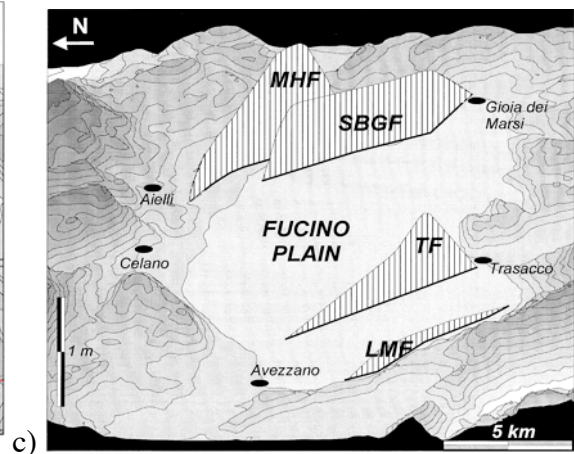
FIG. 3.16 : Evolution du bassin du Fucino. a) Représentation schématique de l'évolution temporelle depuis le Pliocène du bassin du Fucino d'après l'étude des relations stratigraphiques et tectoniques (Galadini et Messina, 1994). 1- ouverture en demi-graben de direction NE-SW sur la faille de Tre-Monti (Pliocène). 2- ouverture en demi-graben d'orientation NW-SE sur les failles du Ventrino, Parasano, Serrone et Trasacco (fin Pliocène – milieu Pléistocène). 3- persistance du régime extensif responsable de l'évolution du demi-graben de direction NW-SE et des mouvements transtensifs sénestres sur certaines failles (Celano-Ovindoli). 'a' failles normales, 'b' failles transtensives sénestres, 'c' pendage des sédiments fluvio-lacustres après déformation due à l'évolution des demi-grabens. b) Ruptures de surface du séisme d'Avezzano (Mw 7) représentées en rouge (Galadini et Galli, 1999). c) Déplacements co-sismiques (m) du séisme d'Avezzano. LMF : faille de Luco dei Marsi, TF : faille de Trasacco, SBF : faille du Mont Serrone, MHF : faille du Mont Parasano.
