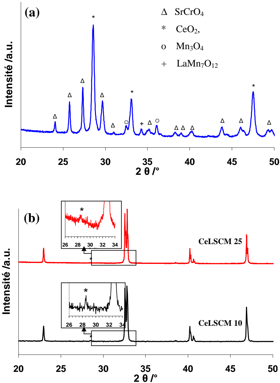
Figure III- 30 : diffractogrammes enregistrés pour les poudres de CeLSCM x ( Ce_xLa_{0,75-x}Sr_{0,25}Cr_{0,5}Mn_{0,5}O_{3-\delta} ) avec x = 0,375 (a) et x = 0,10 et 0,25 (b) traitées sous air à 900\text{ }^\circ\text{C} pendant 48 h.
