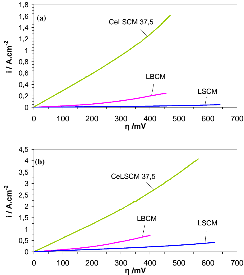
Figure V- 16 : caractéristiques stationnaires à (a) 800 °C et (b) 900 °C sous \text{H}_2 -3 % \text{H}_2\text{O} (géométrie de type P).
