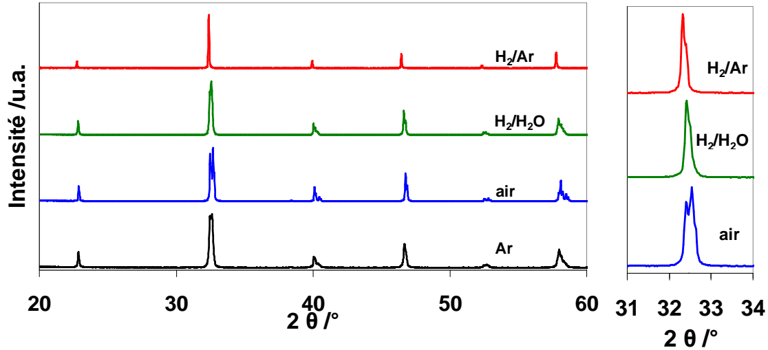
Figure V- 4 : diffractogrammes enregistrés pour LSCM en fonction de l'atmosphère gazeuse. Le diffractogramme enregistré pour LSCM après synthèse sous argon est également présenté.
