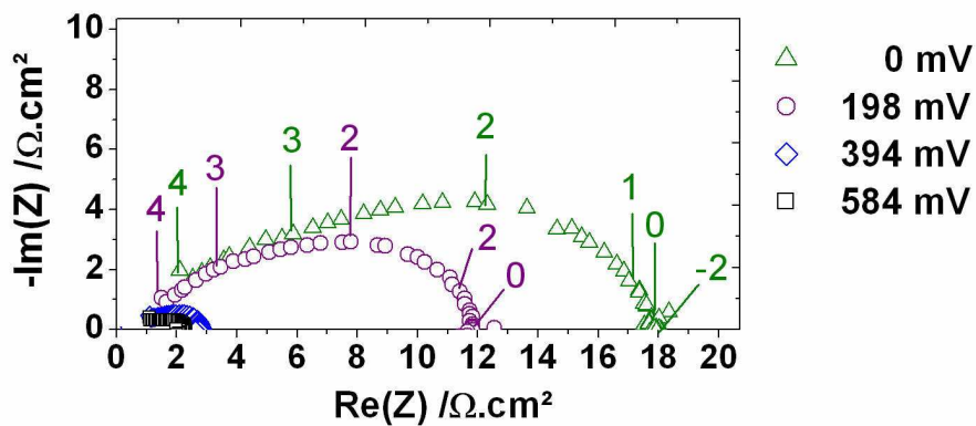
Figure V-17 : caractéristiques d'électrode de LBCM à 800 °C sous \text{H}_2 -3 % \text{H}_2\text{O} (géométrie de type P).
