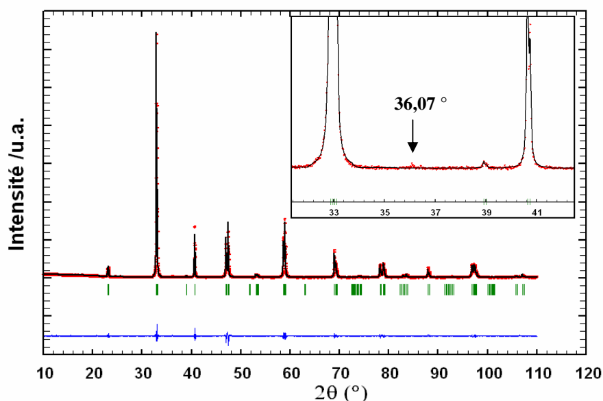
Figure IV- 1 : affinement des paramètres de maille du composé CeSM 25 calciné sous air ( 1500\text{ }^{\circ}\text{C} pendant 10 h) dans le groupe d'espace \text{I4/mcm} . Les diffractogrammes observé et calculé sont respectivement représentés par les points (.) et la ligne continue (—). La ligne continue du bas représente la différence entre ces deux diffractogrammes, et les traits verticaux (I) indiquent les positions des réflexions de Bragg.
