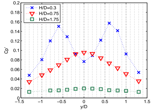
FIG. 5.33 – Répartition du coefficient de pression fluctuante sur la ligne transversale x/D=2.74 : \square H/D=1.75 ; \nabla H/D=0.75 ; \times H/D=0.3
