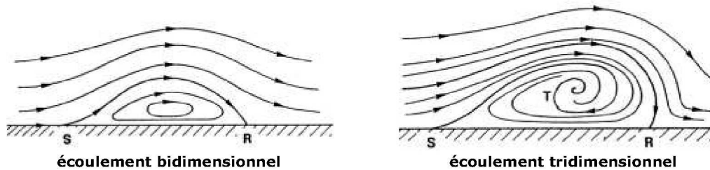
FIG. 2.13 – (gauche) Décollement bidimensionnel idéalisé; (droite) Décollement tridimensionnel réel
