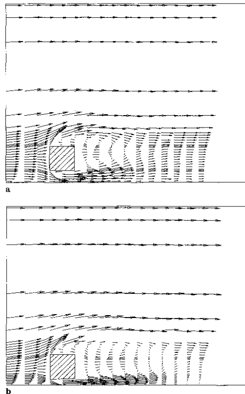
FIG. 2.8 – Écoulement autour du cylindre à base carrée placé proche d'une paroi : (a) H/D = 0.5 ; (b) H/D = 0.25 (Durao et al 1991 [26])
