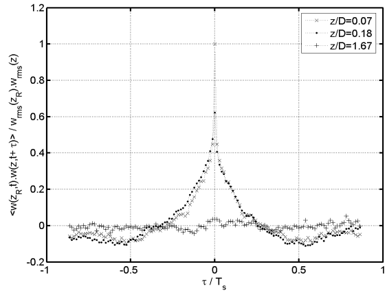
FIG. 7.5 – Evolution temporelle des corrélations spatio-temporelles R_{ww} en x/D = 1.74 pour H/D = 0.3
