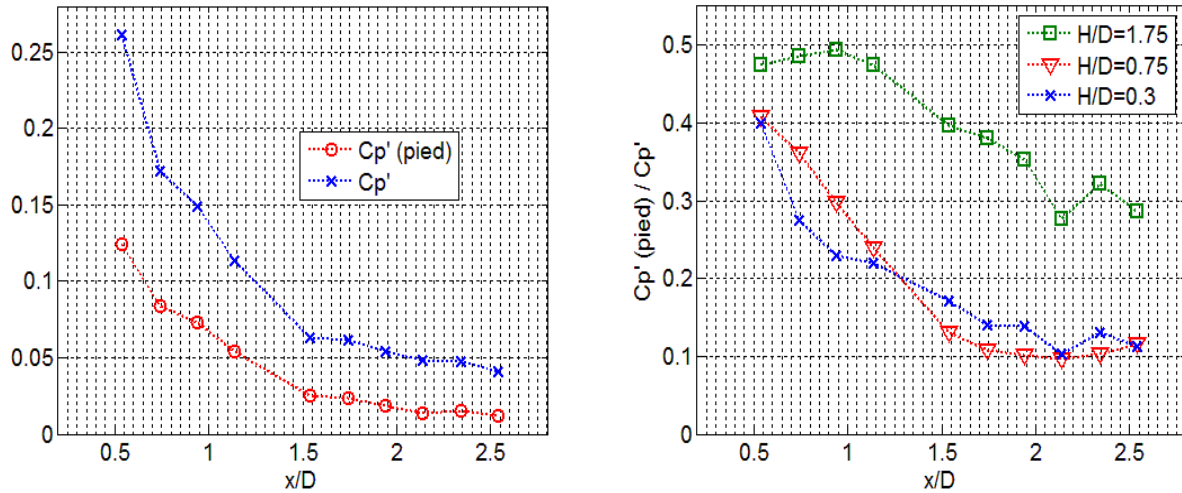
FIG. C.2 – (gauche) Evolution longitudinale du Cp' et du Cp'_{pied} pour H/D = 1.75 ; (droite) Evolution longitudinale de \frac{Cp'_{pied}}{Cp'_{pied} + Cp'_{disque}} .
