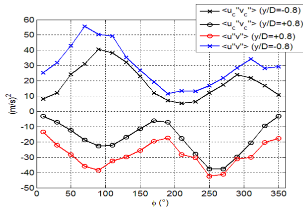
FIG. 7.76 - Evolution de \langle u'' \cdot v'' \rangle et \langle u_c'' \cdot v_c'' \rangle en \langle z_L \rangle ( x/D = 2.74 ) et \langle z_U \rangle ( x/D = 2.74 ) en fonction de la phase \phi_{a_1-a_2} .
