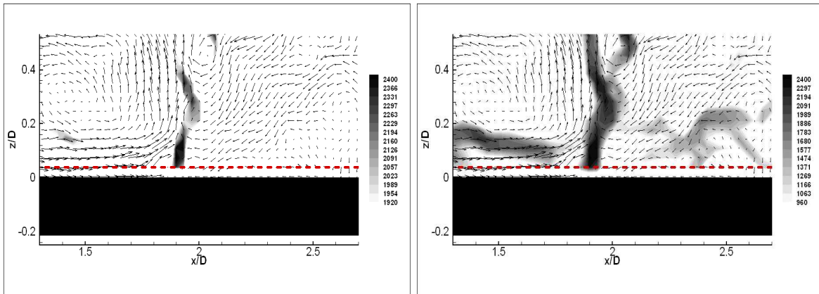
FIG. 7.28 – Champ instantané de FTLE superposé au champ instantané de vitesse : (gauche) filtré à 80% du maximum du champ de FTLE ; (droite) filtré à 40% du maximum du champ de FTLE. — : ligne z/D = 0.039
