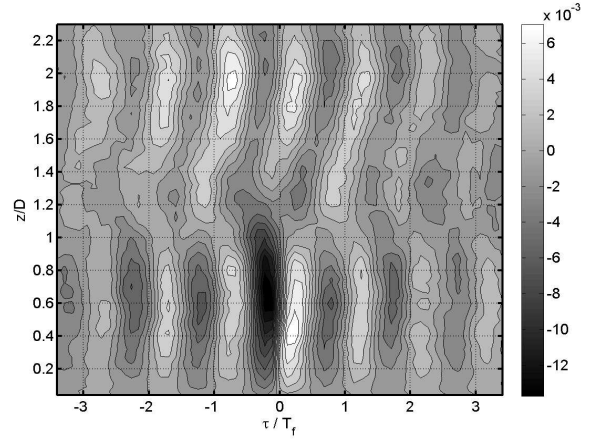
FIG. 6.24 – Corrélations spatio-temporelles R_{pw} en x/D = 1.74 pour H/D = 0,75 .
