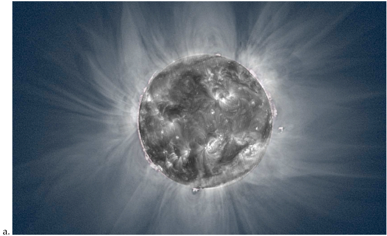
FIGURE 1.1 – Images composites de la couronne solaire observée le 11 août 1999 proche du maximum d'activité (figure du haut a ) puis le 29 mars 2006 en période de minimum (figure du bas b ) à 19.5 nm par l'instrument EIT à bord de la sonde la sonde SOHO (crédits :ESA/NASA) et dans le visible aux limbes lors d'une éclipse totale (crédits :M.Druckmüller).
