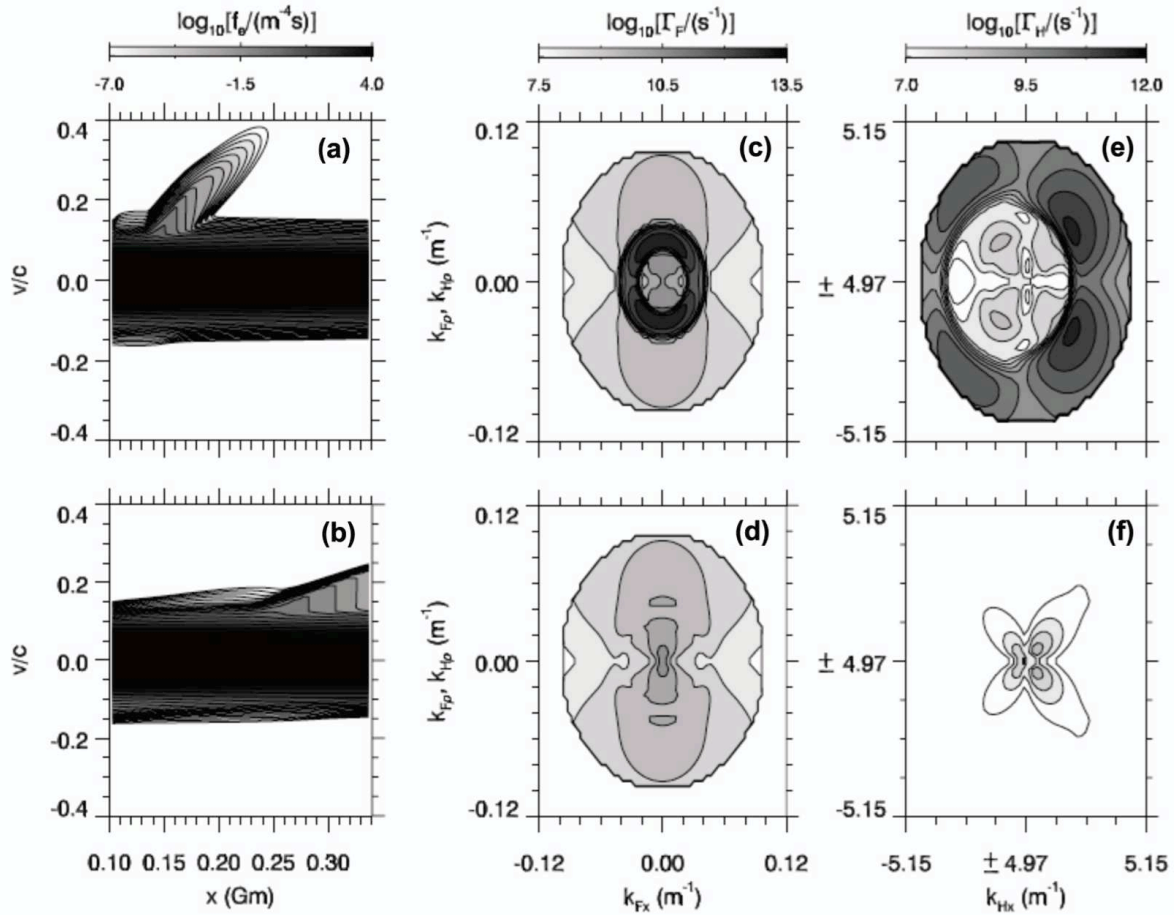
FIGURE 2.7 – Figures a et b : fonction de distribution des électrons f_e ( m^{-4}s ) (nuance de gris en échelle logarithmique) en fonction de l'altitude x (Gm), et de la vitesse normalisée v/c des électrons, à différents instants t_a = 1.2 s, et t_b = 4 s de la simulation. Figures c et d : taux d'émission \Gamma_F ( s^{-1} ) (nuance de gris en échelle logarithmique) du mode F en fonction des vecteurs d'onde k_{Fx} et k_{Fp} , respectivement parallèle et perpendiculaire à la direction de propagation des électrons énergétiques, aux instants t_a et t_b . Figures e et f : même figures que a et b mais pour le mode H. (D'après Li et al. (2008b)).
