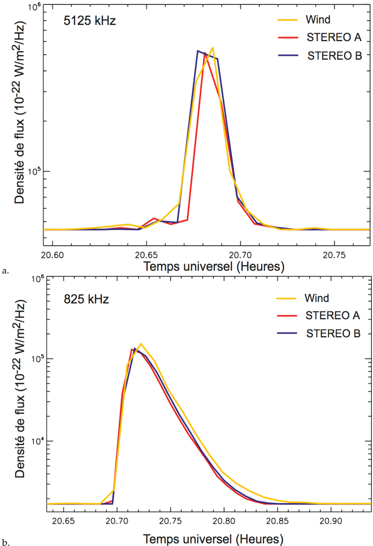
b. FIGURE B.3 – Comparaison des données radio étalonnée en flux sur Wind, STEREO-A, et STEREO-B. la figure a représente le profil temporel d'intensité à 5125 kHz d'un sursauts de type III observé le 23 janvier 2007 par les sondes : Wind (courbe jaune), STEREO-A (courbe rouge), et STEREO-B (courbe bleue). A cette époque, les trois sondes se trouvent encore dans l'environnement terrestre. La résolution temporelle vaut environ 30 s pour les trois sondes. La figure b représente le même sursaut observé à 825 kHz.
