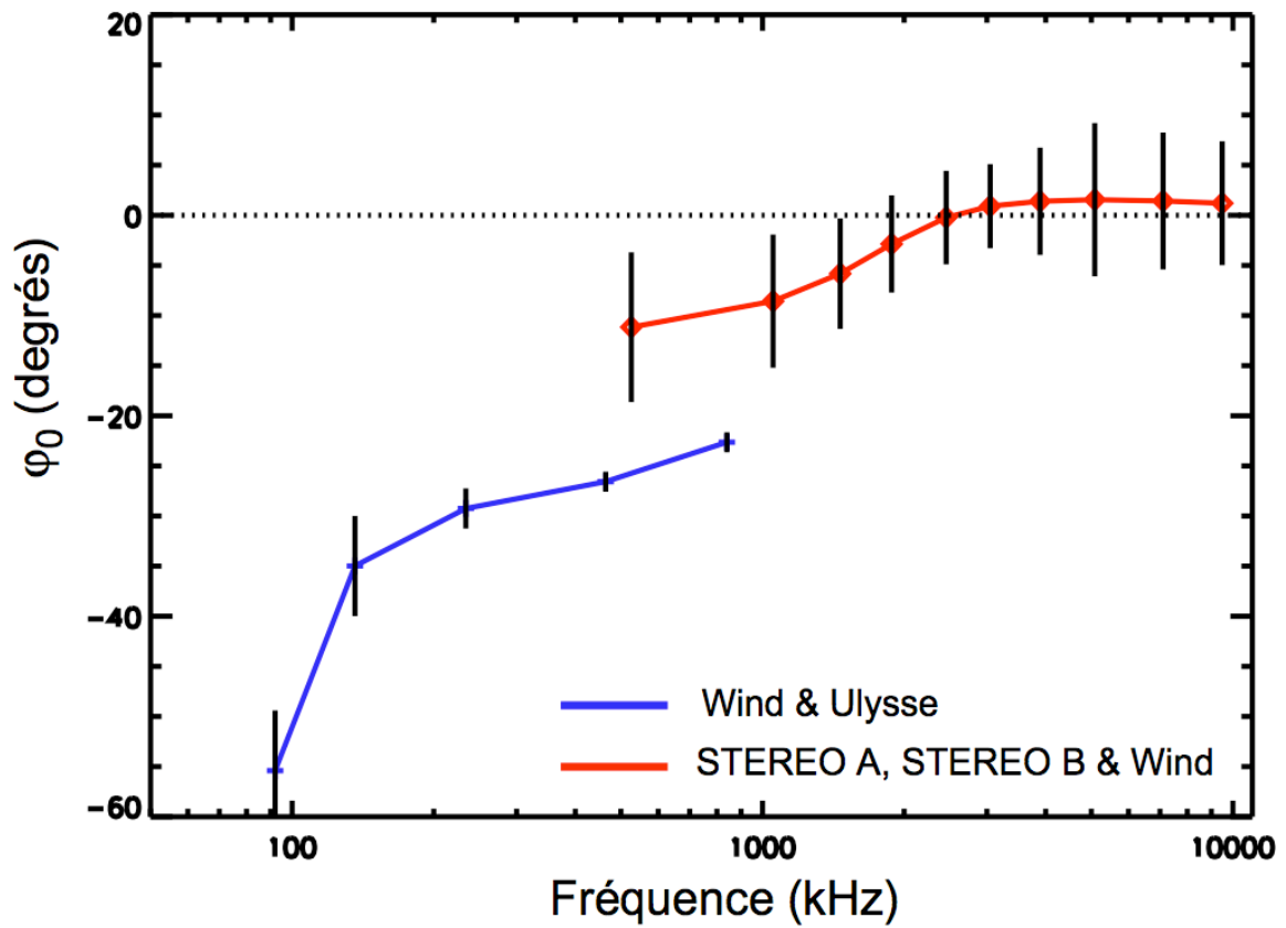
FIGURE 4.2 – Paramètres \varphi_0 (a) et \Delta\varphi_2 (b) en fonction de la fréquence. Les losanges et la courbe rouge correspondent aux valeurs obtenues par ajustement avec les données STEREO-A, STEREO-B, et Wind. Pour comparaison, les croix noires et la courbe bleue présentent les valeurs issues de l'étude réalisée en dessous de 1 MHz par Wind et Ulysse.
