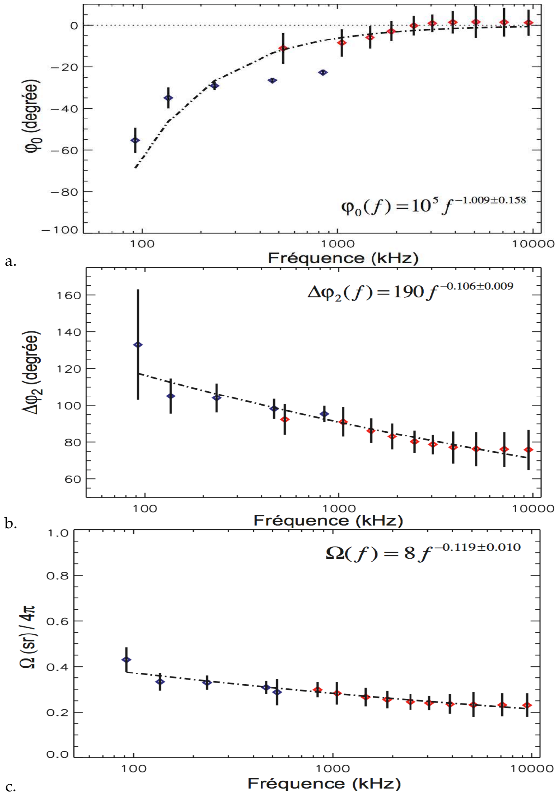
FIGURE 4.3 – Les figures a , b , et c , présentent respectivement l’ajustement de l’axe du diagramme \varphi_0 (degré), de l’ouverture angulaire du diagramme \Delta\varphi_2 (degré), et de l’angle solide \Omega (stéradian) normalisé à 4\pi de la source, en fonction de la fréquence. Les points bleus et rouges correspondent respectivement aux paramètres obtenus à partir des Wind et Ulysses d’une part, et STEREO-A, STEREO-B, et Wind d’autre part. Les courbes pointillées noires sur chaque graphe représentent les fonctions (4.6), (4.7), et (4.8) après ajustement ; fonctions qui sont également indiquées avec les valeurs ajustées.
