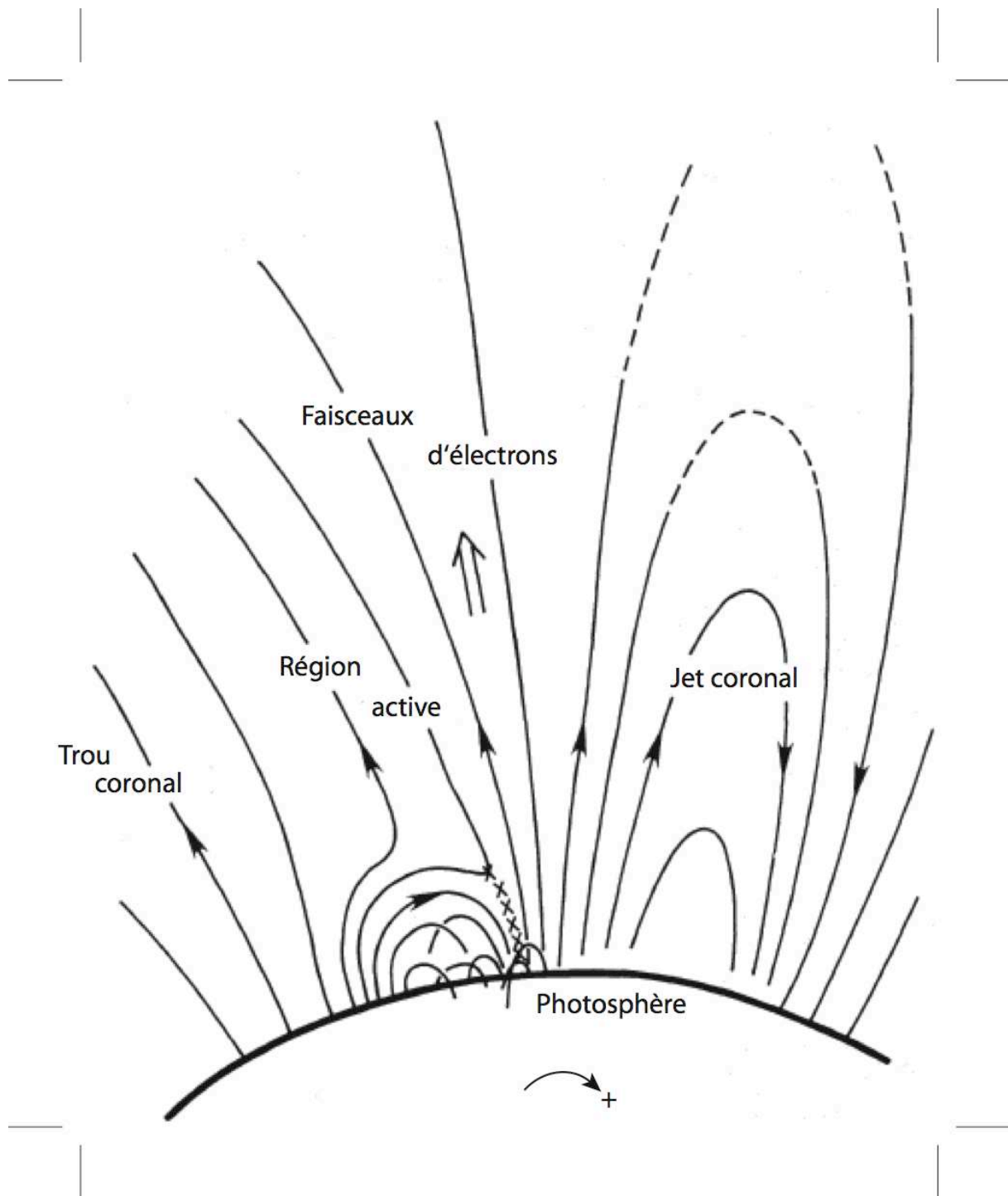
FIGURE 2.4 – Illustration simplifiée de la région de propagation des faisceaux d'électrons produisant les sursauts de type III dans la couronne (adaptée de Poquérousse et al. 1988). Les électrons sont éjectés le long de lignes de champ ouvertes sur le milieu interplanétaire, préférentiellement en périphérie des régions actives où règne un réseau complexe de boucles magnétiques fermées s'élevant dans la couronne.
