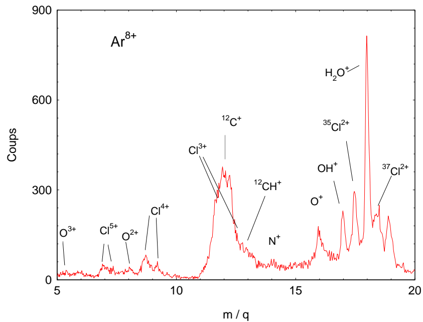
FIGURE 3.15 – Spectre montrant les petits fragments positifs formés lors de la collision de la molécule de porphyrine avec \text{Ar}^{8+} à 80 keV.
