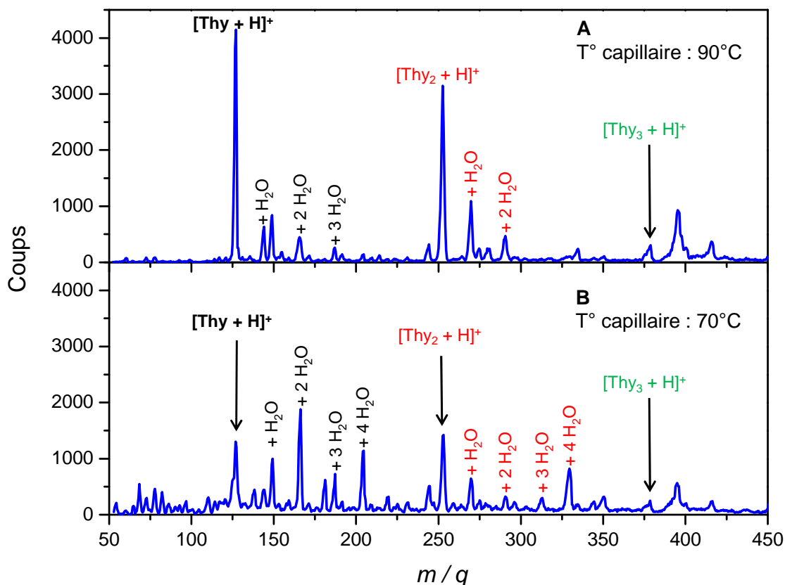
FIGURE 8.10 – Effet de la température du capillaire chauffant sur la désolvatation de la thymine dans une solution de méthanol additionnée d'1% d'acide acétique. Remarquons que le nombre de molécules d'eau restant attachées à la thymine est beaucoup plus important que dans le cas de l'adénine.
