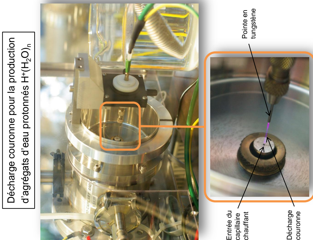
FIGURE 8.14 – Dispositif utilisé pour la production d'agrégats d'eau protonnés de la forme H^+(H_2O)_n . Le principe consiste à créer une décharge couronne entre une pointe de tungstène et l'entrée du capillaire chauffant de la source electro-spray. La fabrication de la pointe est réalisée à partir d'un barreau de tungstène par une réaction électrochimique dans une solution de KOH.
