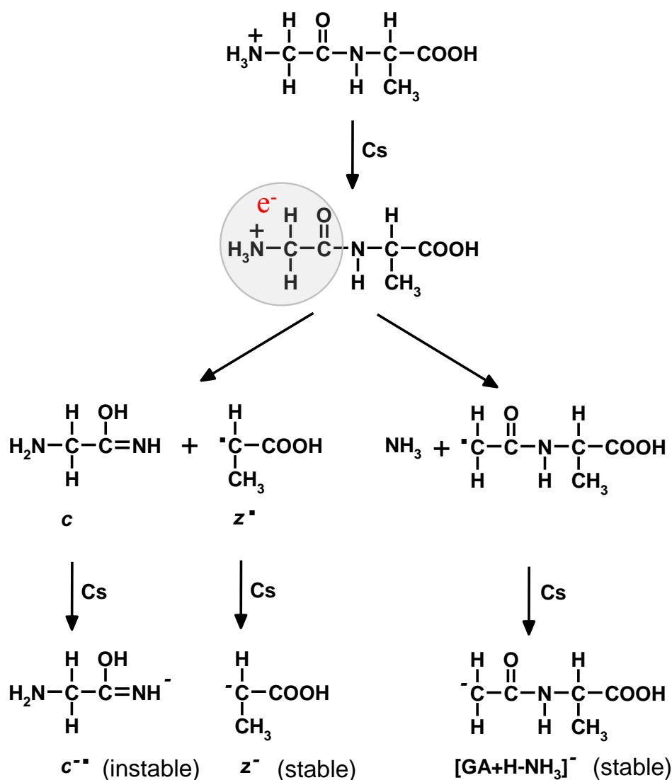
FIGURE 7.3 – La capture électronique au niveau de la région N-terminal conduit à la perte d'ammoniac ( \text{NH}_3 ) ou à la cassure de la liaison \text{N-C}_\alpha .
