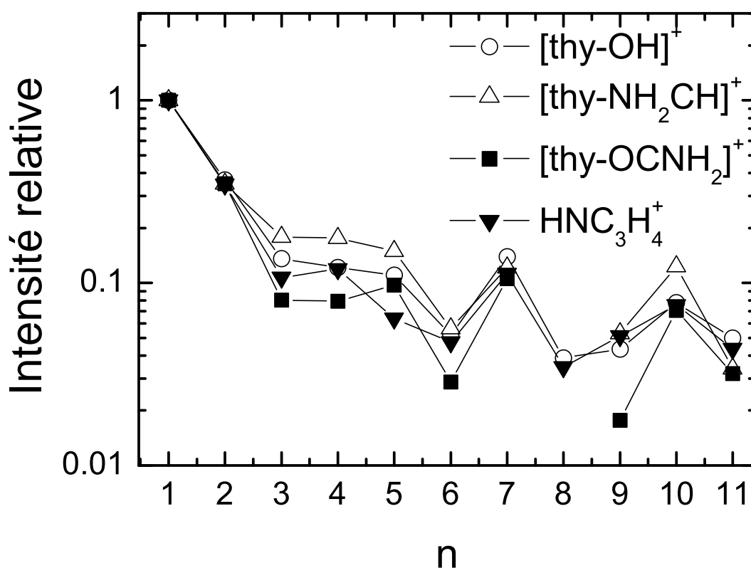
FIGURE 5.17 – Représentation sur une échelle logarithmique de l'intégrale des pics des fragments [\text{thy-OH}]^+ , [\text{thy-NH}_2\text{CH}]^+ , [\text{thy-OCNH}_2]^+ et \text{HNC}_3\text{H}_4^+ observés en coïncidence avec l'espèce \text{thy}_n^+ . Ces données sont obtenues lors de la collision d'agrégats neutres de thymine avec des ions \text{O}^{5+} à 50 keV. L'intensité des fragments produits lors de la détection du cation \text{thy}^+ a été normalisée à 1.
