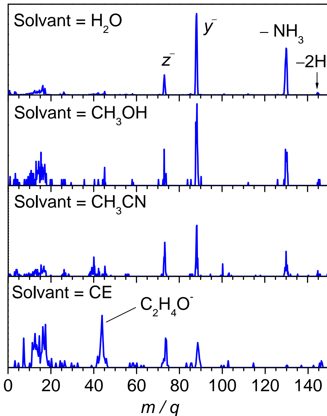
FIGURE 7.4 – Spectres de fragmentation issus de la collision entre le dipeptide solvatoé [GA+H] + (S) et des atomes de césium. Il s'agit de spectres de « charge opposée » des fragments négatifs formés lorsqu'une molécule de H 2 O, de CH 3 OH, de CH 3 CN et enfin d'éther couronne est attachée à la biomolécule.
