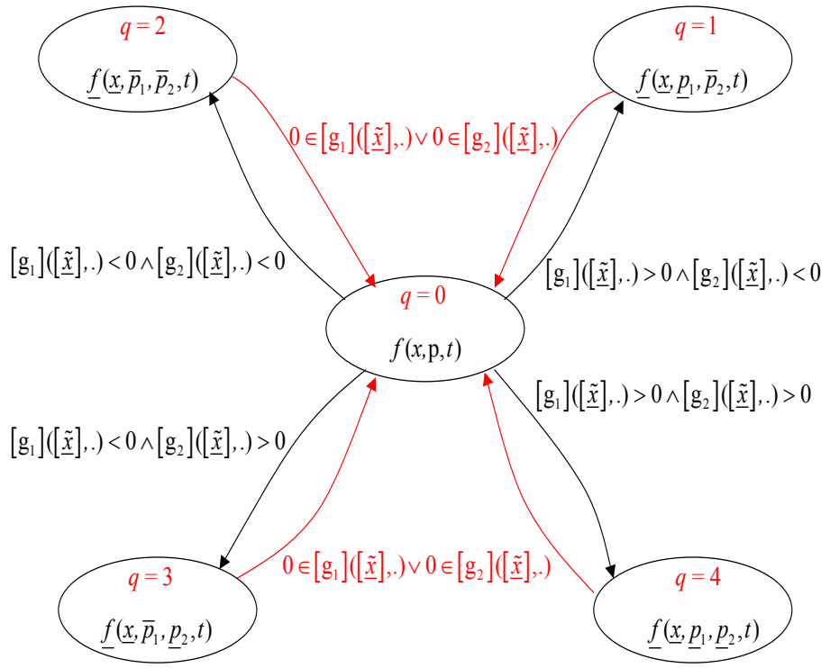
FIG. IV.9 : Automate hybride inférieur
