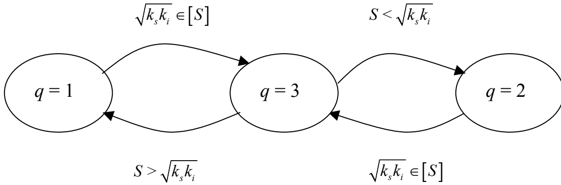
FIG. VI.21 : Automate hybride d'observation.
