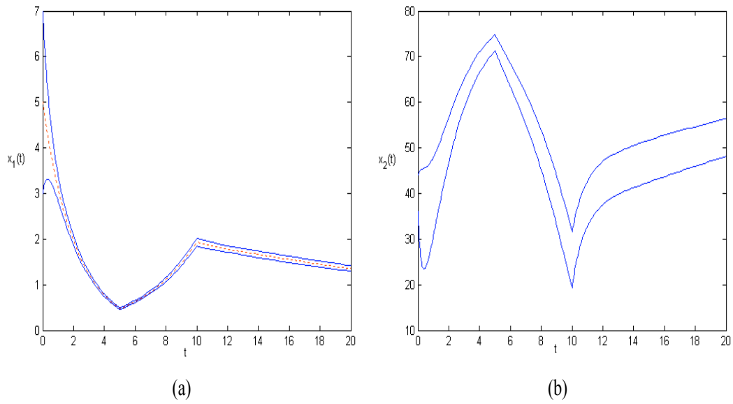
FIG. VI.22 : Encadrement de toutes les trajectoires d'état admissibles : (a) [x_1](t) ; (b) [x_2](t) .
