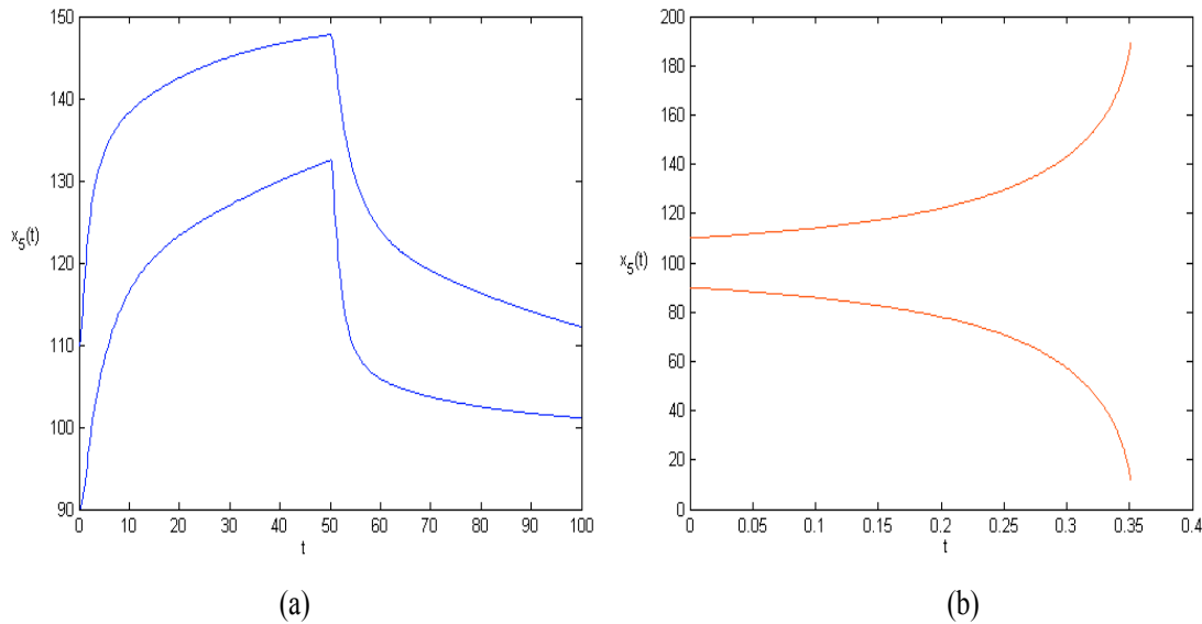
FIG. IV.11 : Encadrement de toutes les solutions possibles de x_5(t) : (a) Méthode hybride d'encadrement; (b) Méthode de Hermite-Obreschkoff intervalle. Arrêt de l'algorithme de calcul après 0.35 seconde d'intégration.
