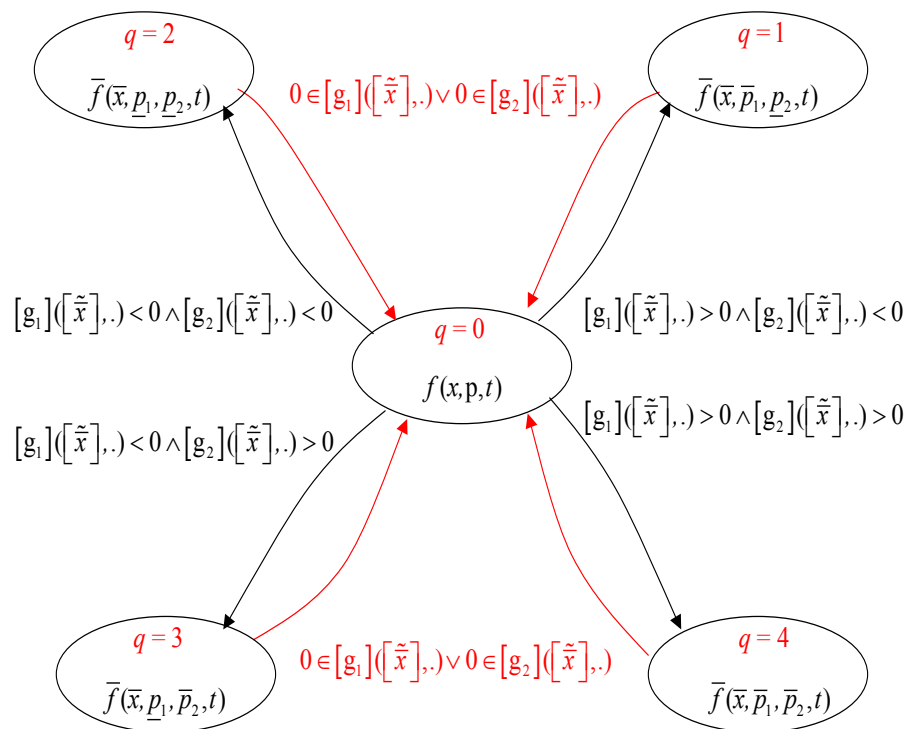
FIG. IV.10 : Automate hybride supérieur
