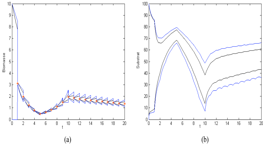
FIG. VI.11 : Encadrement de toutes les valeurs possibles des deux variables d'état dans le contexte de l'essai 3 : (a) Biomasse ; (b) Substrat.
