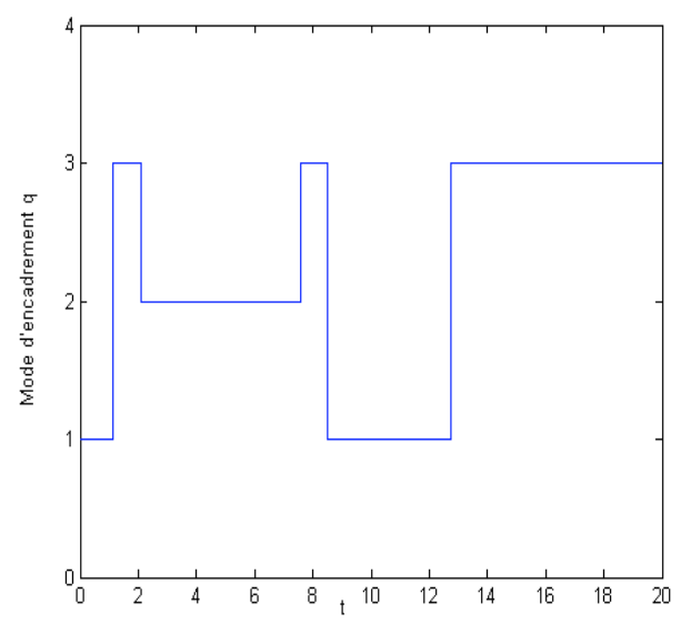
FIG. VI.23 : Evolution du mode d'encadrement
