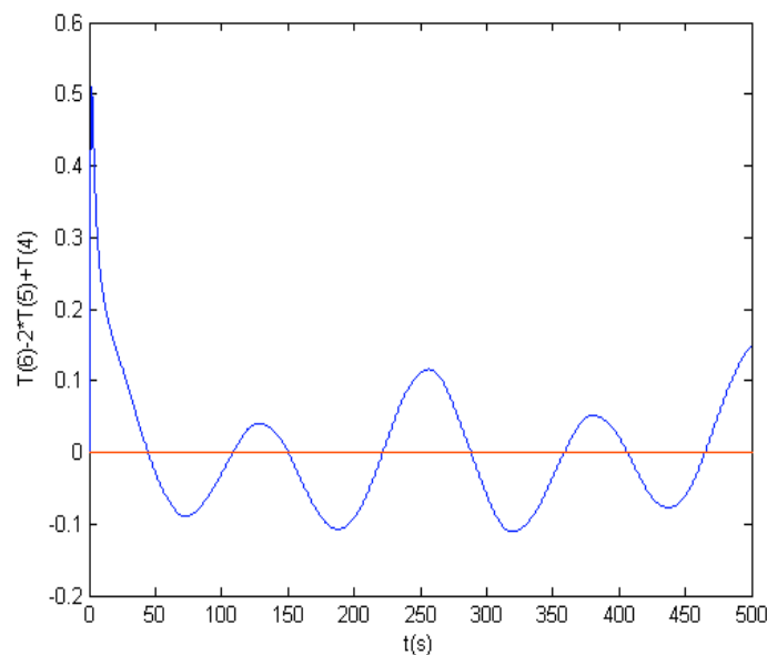
FIG. V.22 : L'évolution temporelle de la dérivée partielle g_{5,1}(\cdot) du système (V.7)
