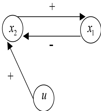
FIG. III.1 : Graphe d'incidence d'un système non préservateur d'ordre.
