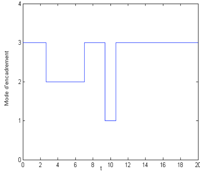
FIG. VI.14 : Evolution du mode d'encadrement dans le contexte de l'essai 4.
