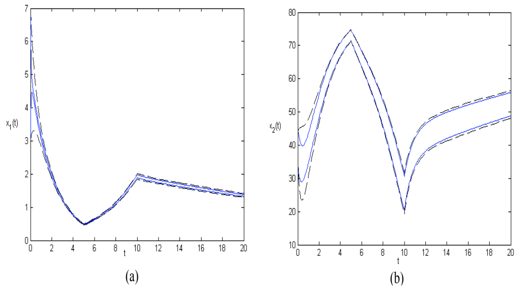
FIG. VI.24 : Encadrement de toutes les trajectoires d'état possibles dans le contexte du deuxième essai : (a) [x_1](t) ; (b) [x_2](t) .
