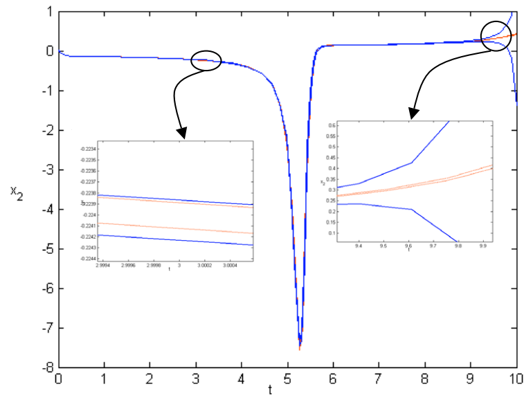
FIG. II.7 : Exemple d'intégration avec la méthode de Hermite-Obreschkoff : Deuxième composante du vecteur solution \mathbf{x}(t) .
