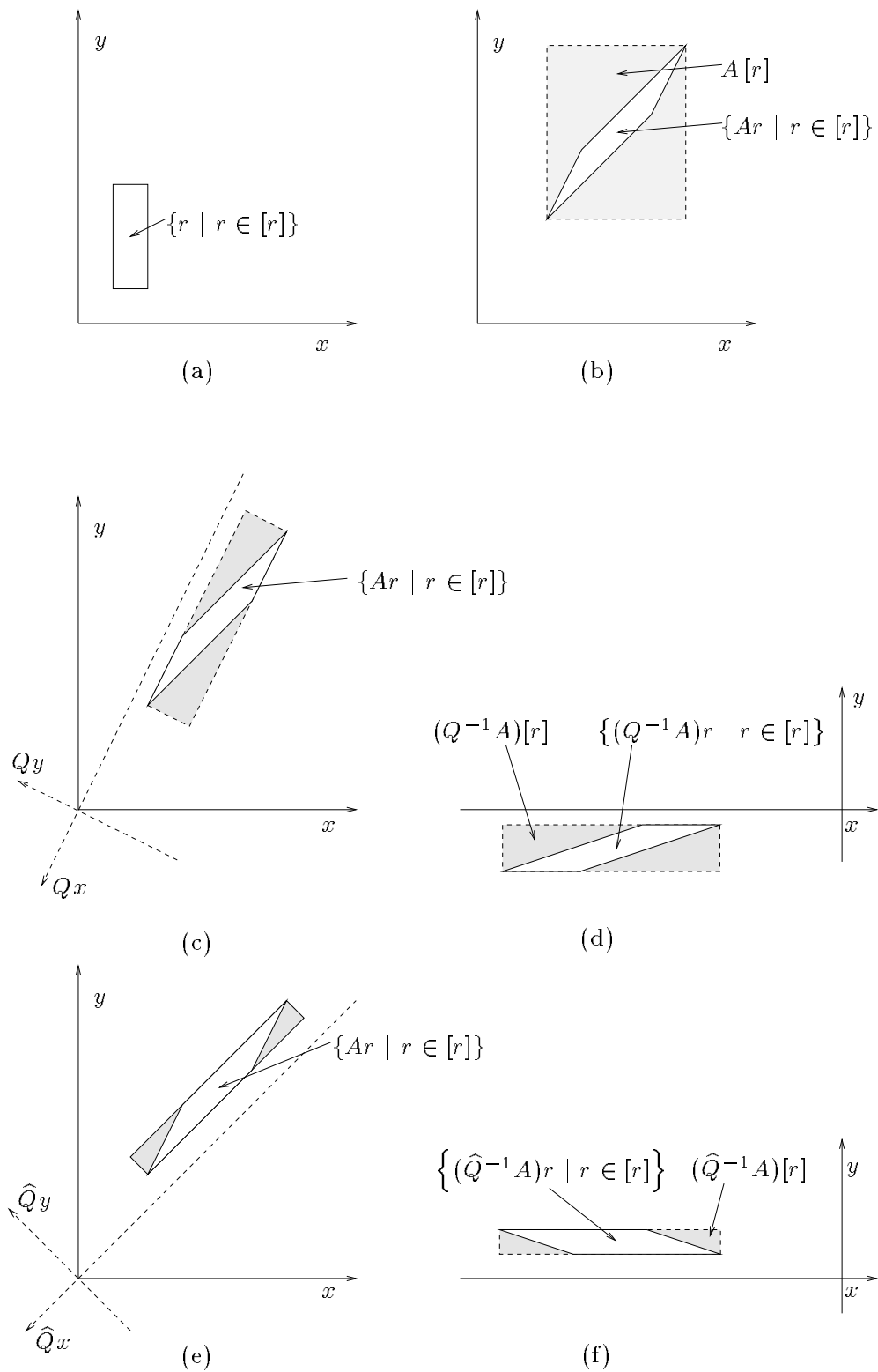
FIG. II.3 : Factorisation QR [69].
