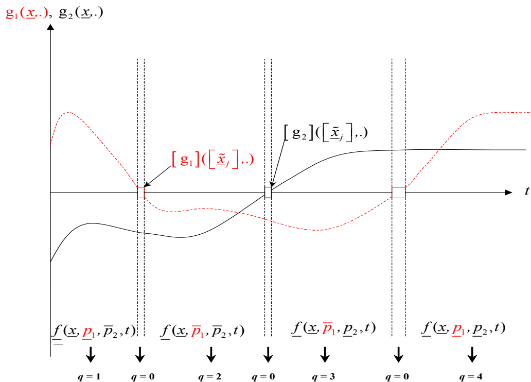
FIG. IV.7 : Les différents modes d'encadrement inférieurs possibles de (IV.18)
