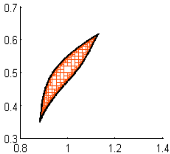
FIG. V.16 : Approximation intérieure (pavés en rouge) de l'ensemble solution. Couche d'incertitude (pavés en noir), TC=6h .
