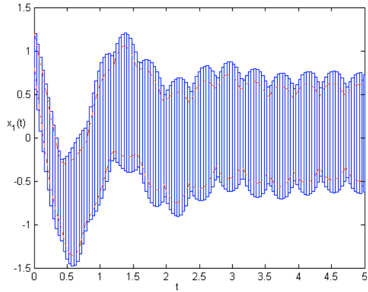
FIG. VII.4 : L'évolution temporelle de [x_1] . Simulation par la méthode de HOI.
