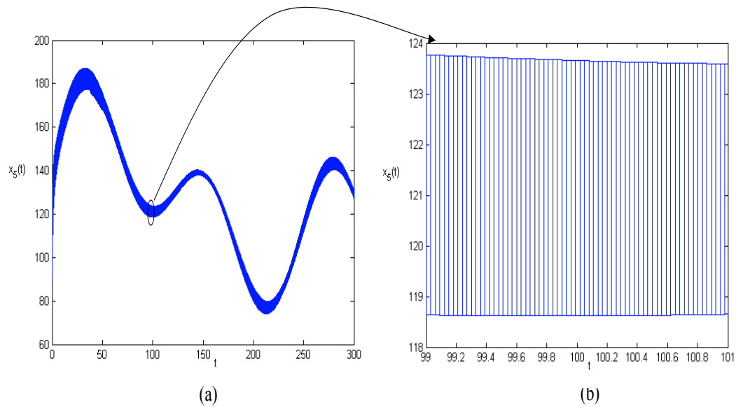
FIG. VII.10 : L'évolution temporelle de la variable d'état [x_5](t) . Simulation par l'algorithme Hybrid_Bound_Solution . Temps CPU=250s.
