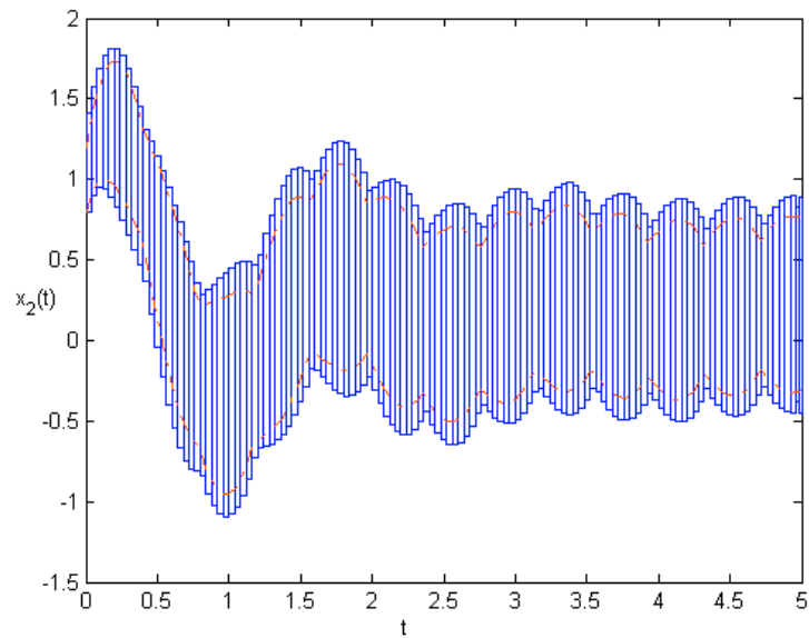
FIG. VII.5 : L'évolution temporelle de [x_2] . Simulation par la méthode de HOI. Temps CPU=0.5 sec (PIII 1.2MHz)
