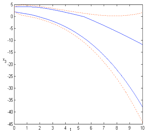
FIG. IV.5 : Encadrement de toutes les solutions possibles de x_3(t) : courbes rouges pointillées méthode de Hermite-Obreschkoff; courbes bleues continues méthode hybride d'encadrement.
