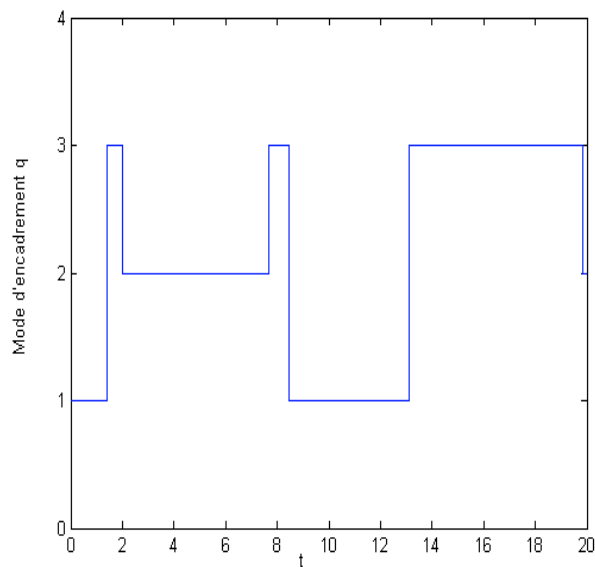
FIG. VI.25 : Evolution du mode d'encadrement dans le contexte du deuxième essai
