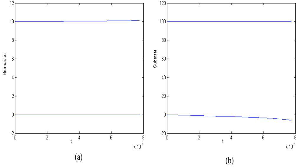
FIG. VI.3 : Arrêt de l'algorithme d'estimation d'état après quelques pas d'intégration (essai 1).
