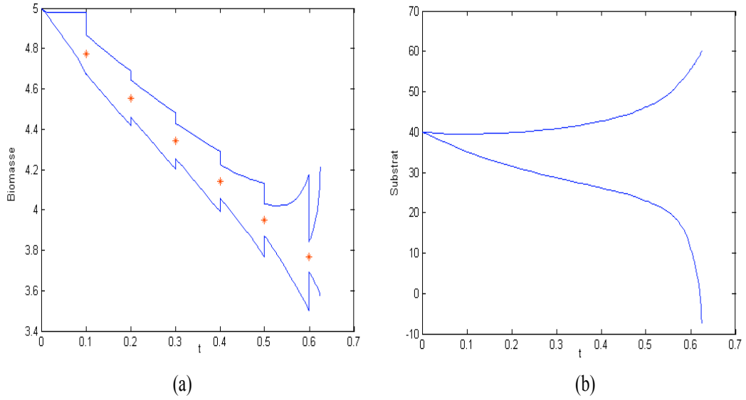
FIG. VI.4 : Divergence de la taille des encadrements des variables d'état représentées par les courbes bleues continues (essai 2). La courbe rouge pointillée représente le signal discret de mesure.
