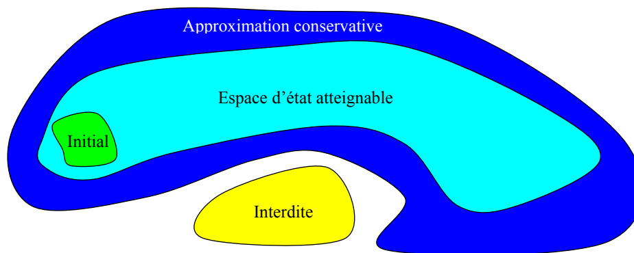
FIG. VII.1 : Exemple de vérification de sûreté d'un système incertain
