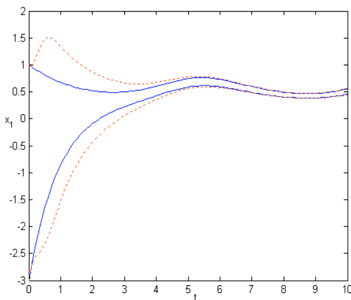
FIG. III.13 : Encadrement de toutes les valeurs possibles de x_1(t) . Courbes bleues continues méthodes basées sur le théorème de Müller, courbes rouges pointillés méthode de Hermite-Obreschkoff intervalle.
