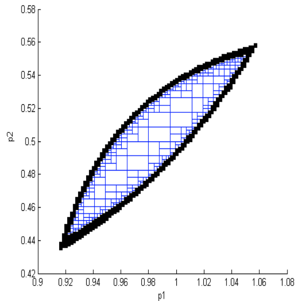
FIG. V.28 : Approximation intérieure (pavés en bleu) de l'ensemble solution. Couche d'incertitude (pavé en noir), TC=24h .
