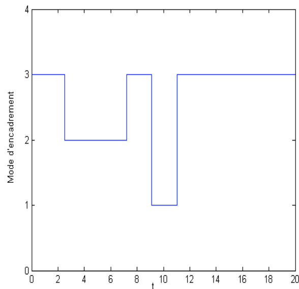
FIG. VI.8 : Evolution du mode d'encadrement dans le contexte de l'essai 1.
