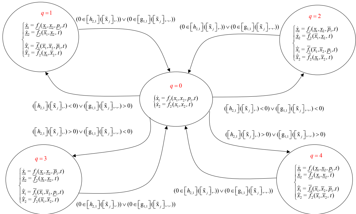
FIG. IV.2 : Automate hybride
