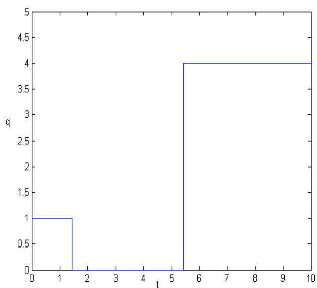
FIG. IV.6 : Les différents modes d'encadrement utilisés au cours de l'intégration garantie (IV.14).
