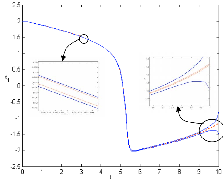
FIG. II.6 : Exemple d'intégration avec la méthode de Hermite-Obreschkoff : Première composante du vecteur solution \mathbf{x}(t) .
