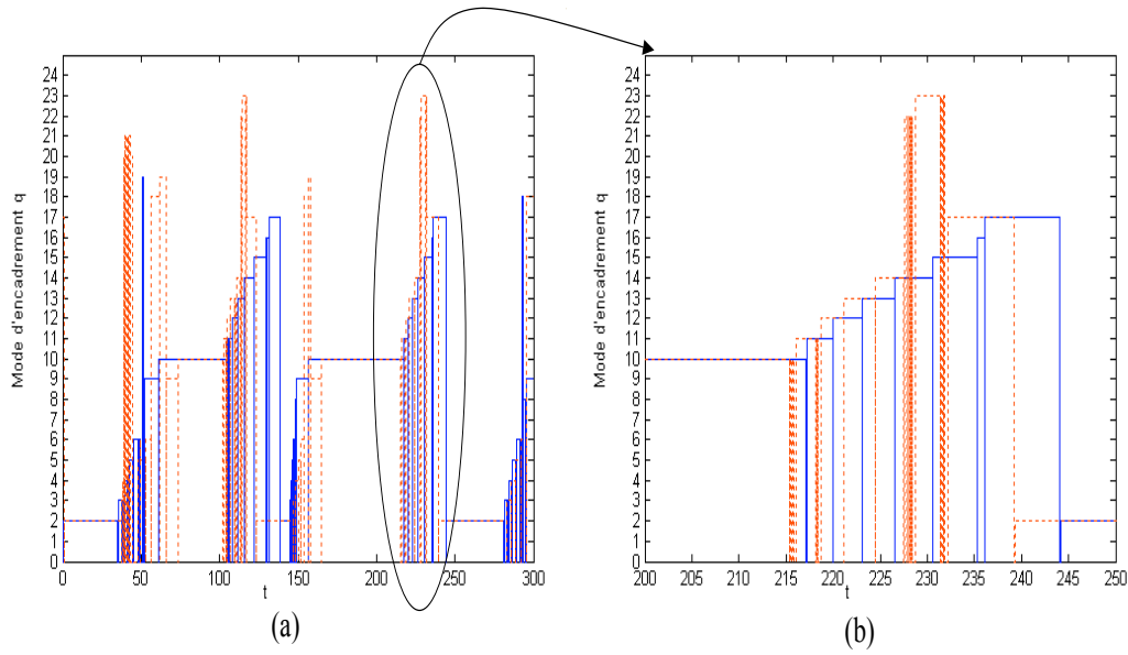
FIG. VII.12 : L'évolution du mode d'encadrement (ligne continue : système supérieur, ligne discontinue : système inférieur). Simulation par l'algorithme Hybrid_Bound_Solution .
