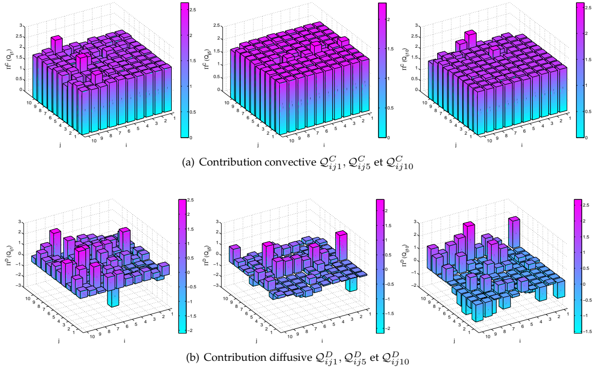
Figure F.3 : Comparaison des contributions relatives des termes convectifs et diffusifs quadratiques Q_{ijk}^C et Q_{ijk}^D .
