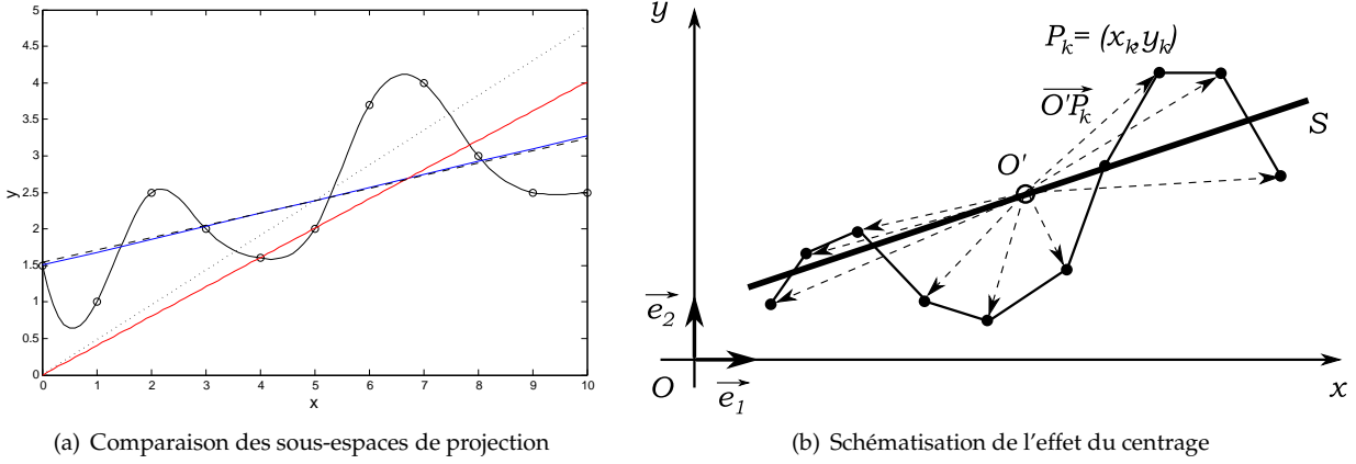
Figure 2.2 : Effet du centrage des clichés sur l'approximation POD d'un ensemble de points de \mathbb{R}^2 .
