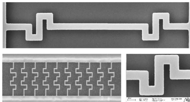
FIGURE 2.18 – Images MEB de nanofils créneaux. Ces fils ont une largeur de 200\text{nm} , le décrochement est de 400\text{nm} .
