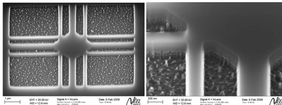
FIGURE 2.14 – Image MEB d'échantillons réalisés à NANOFAB au cours de cette thèse. Des réseaux de nanofils et des membranes suspendues ont été développés pour l'étude des propriétés thermiques à l'échelle mésoscopique. En haut à gauche, un réseau de 50 nanofils droits d'une longueur de 8\mu\text{m} et d'une section de 200\times 200\text{ nm}^2 . En haut à droite un réseau de 10 nanofils de 5\mu\text{m} de longs présentant des cavités, qui peuvent entraîner une diminution de la conductance thermique [42,67,89]. En bas à gauche une membrane de silicium suspendue de 1\mu\text{m} de côté, et en bas à droite un premier prototype de futurs capteurs suspendus pour la mesure par une méthode statique de la conductance thermique des nanobras de suspension (chapitre 6).
