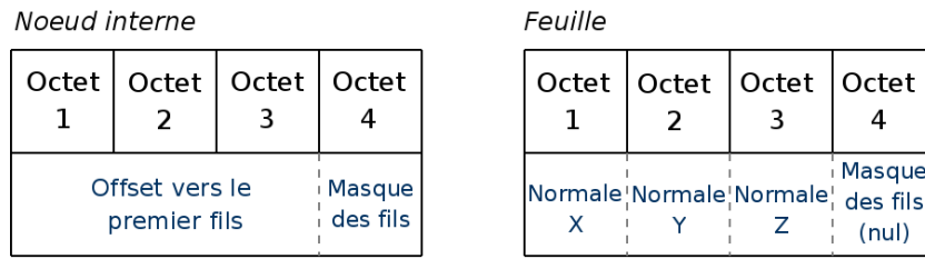
FIG. 3.17 – Encodage sur 4 octets des nœuds et feuilles de l'octree.
