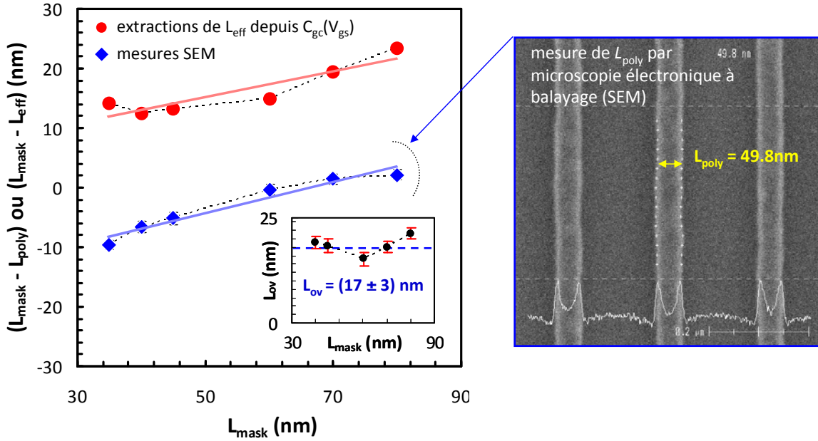
Fig. IV.21 – Comparaison entre la valeur de la réduction de la longueur de canal L_{mask} - L_{eff} obtenue par mesures capacitive et la valeur L_{mask} - L_{gate} mesurée grâce à des techniques de microscopie électronique à balayage. Les deux longueurs L_{eff} et L_{gate} présentent des variations similaires et la longueur de recouvrement L_{ov}(L_{mask}) est quasi-constante ( L_{ov} = 17 \pm 3 nm), en accord avec le fait que l’architecture de jonction reste la même quelque soit la longueur du dispositif.
