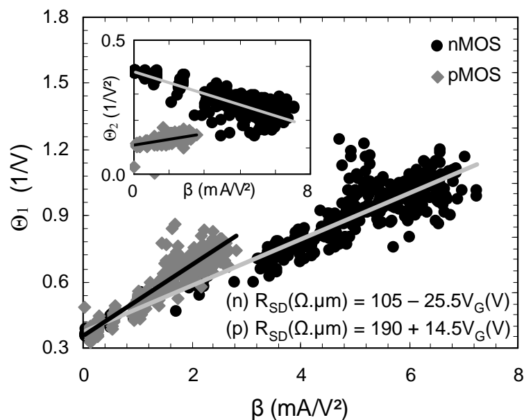
Fig. III.27 – Extraction de R_{sd}(V_{gs}) pour les n MOS et p MOS de la technologie 45nm. Les longueurs de grille vont de 35nm à 1\mu\text{m} , la largeur étant fixée à W = 1\mu\text{m} .
