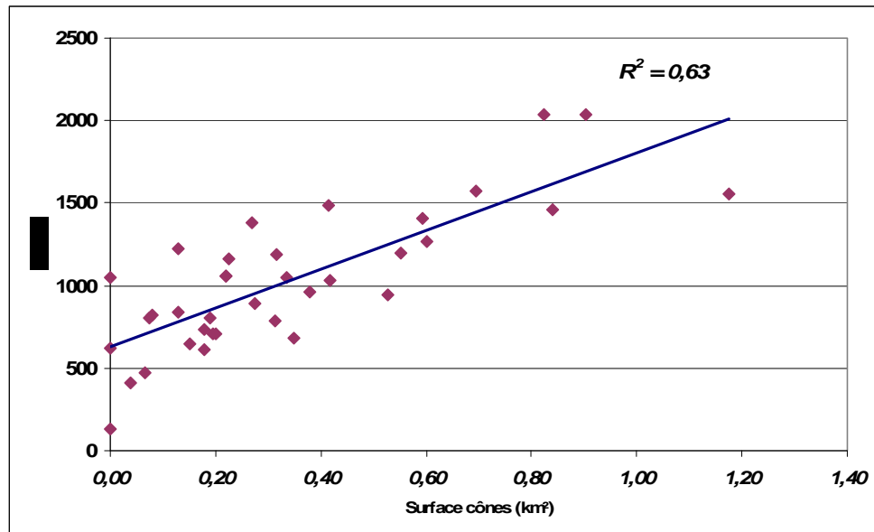
Figure 68: Relation entre la largeur de vallée et la surface des cônes torrentiels.
