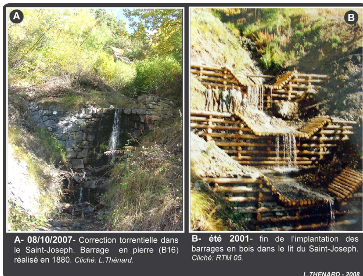
Figure 106: Correction RTM passée et actuelle dans le torrent de Saint-Joseph (Comm. du Monétier-les-Bains).
