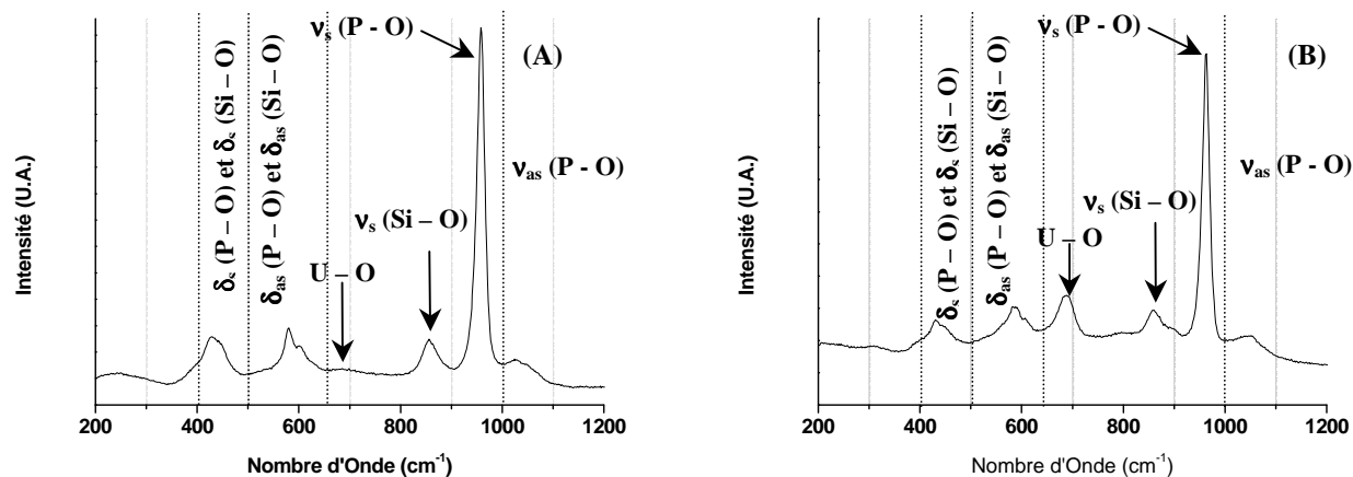
Figure II.3. Spectres \mu -Raman d'échantillons de britholites - Th (A) et de britholites - (Th,U) (B) calcinés à 1390°C pendant 12 heures.
