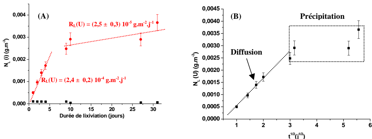
Figure III.12. Evolution des pertes de masse normalisées relevées lors de la dissolution de \text{Ca}_{0,5}\text{Th}_{0,4}\text{U}_{0,1}\text{PO}_4 ( N_L(\text{Th}) (■), N_L(\text{U}) (●) à 90^\circ\text{C} dans \text{HNO}_3 10^{-1} M (A) et variation de la perte de masse normalisée N_L(\text{U}) (■) en fonction de la racine carrée du temps (B).
