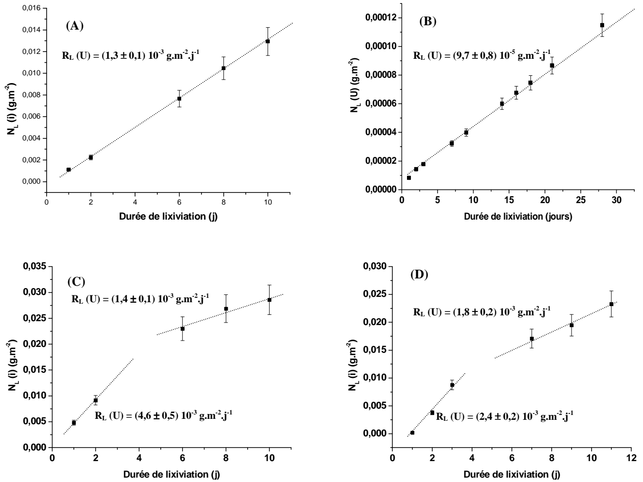
Figure III.19. Evolution des pertes de masse normalisées N_L(U) lors de la dissolution d'échantillons de \text{Ca}_{0,5}\text{Th}_{0,3}\text{U}_{0,2}\text{PO}_4 à 70^\circ\text{C} (A), de \text{Ca}_{0,5}\text{Th}_{0,4}\text{U}_{0,1}\text{PO}_4 à 70^\circ\text{C} (B), de \text{Ca}_{0,5}\text{Th}_{0,2}\text{U}_{0,3}\text{PO}_4 à 70^\circ\text{C} (C) et de \text{Ca}_{0,5}\text{Th}_{0,1}\text{U}_{0,4}\text{PO}_4 (B) dans \text{HNO}_3 10^{-1}\text{M} .
