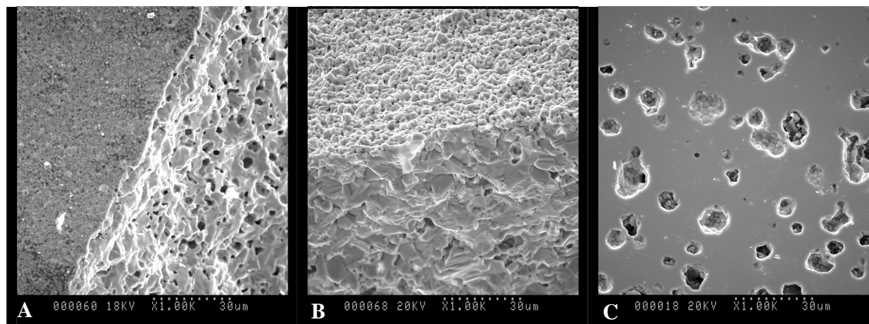
Figure II.8. Observations réalisées par MEB d'échantillons frittés de Ca_{0,5}Th_{0,4}U_{0,1}PO_4 (face de rupture) (A) , de La_{0,5}Ca_{0,25}Th_{0,15}U_{0,1}PO_4 (face de rupture) (B) et de Ca_{0,5}Th_{0,25}U_{0,25}PO_4 (surface polie) (C) calcinés à 1300^\circ C pendant 10 heures.
