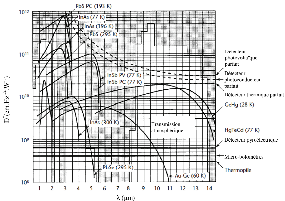
Figure 4.4 : Détectivité D^* en fonction de la longueur d'onde \lambda pour différents types de capteurs infrarouges (Maldague, 2001).
