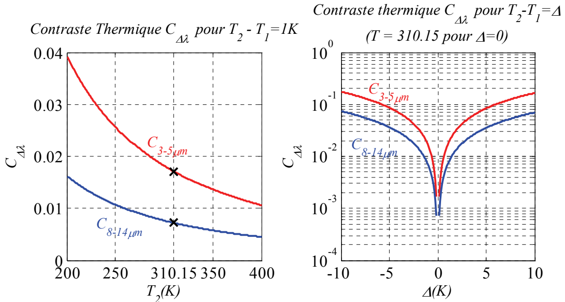
Figure 4.5 : Contraste thermique dans les bandes MWIR et LWIR , à gauche, nous avons tracé le contraste pour T_2 - T_1 = 1\text{K} , à droite, nous avons tracé le contraste pour des \Delta(\text{K}) autour de T_{\text{corps}}=310.15\text{K} .
