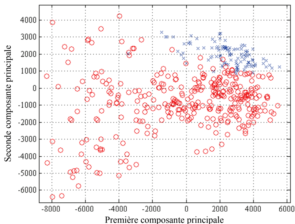
Figure 3.20 : Projection des spectres Log-polaires des images de bouche sur les 2 premières composantes principales données par ACP. Le nuage de points bleus correspond aux bouches fermées, le nuage de points rouges correspond aux bouches ouvertes.
