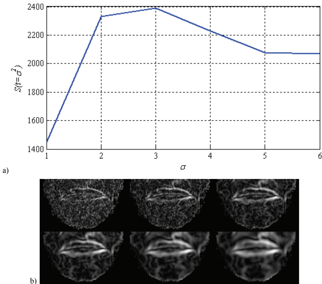
Figure 2.19 : Évolution de S(t=\sigma^2) , a) tracé de S(t=\sigma^2) , b) images de l'intensité des gradients \nabla_{norm}L(x, y, t) pour 1 < \sigma < 6 .
