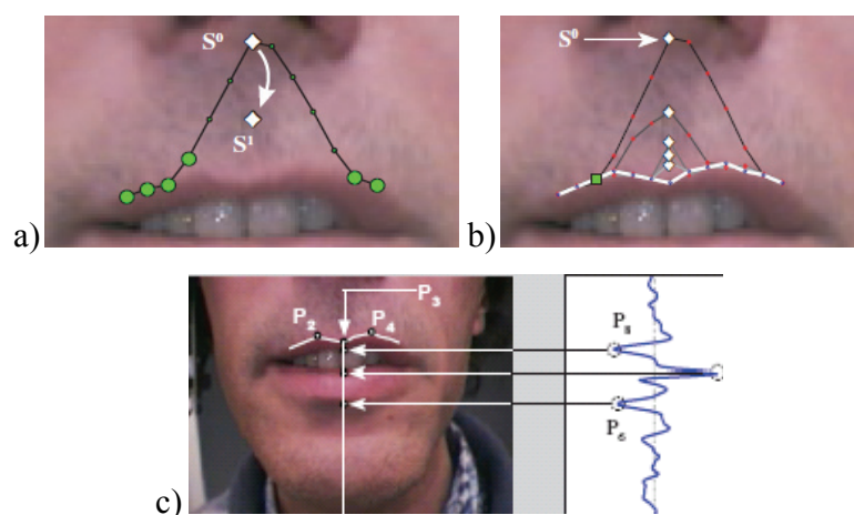
Figure 1.31 : Jumping snake (Eveno, 2004), a) Snake initial, b) Tracés des snakes pour les nouvelles positions du germe, c) Recherche du point bas du contour externe inférieur.
