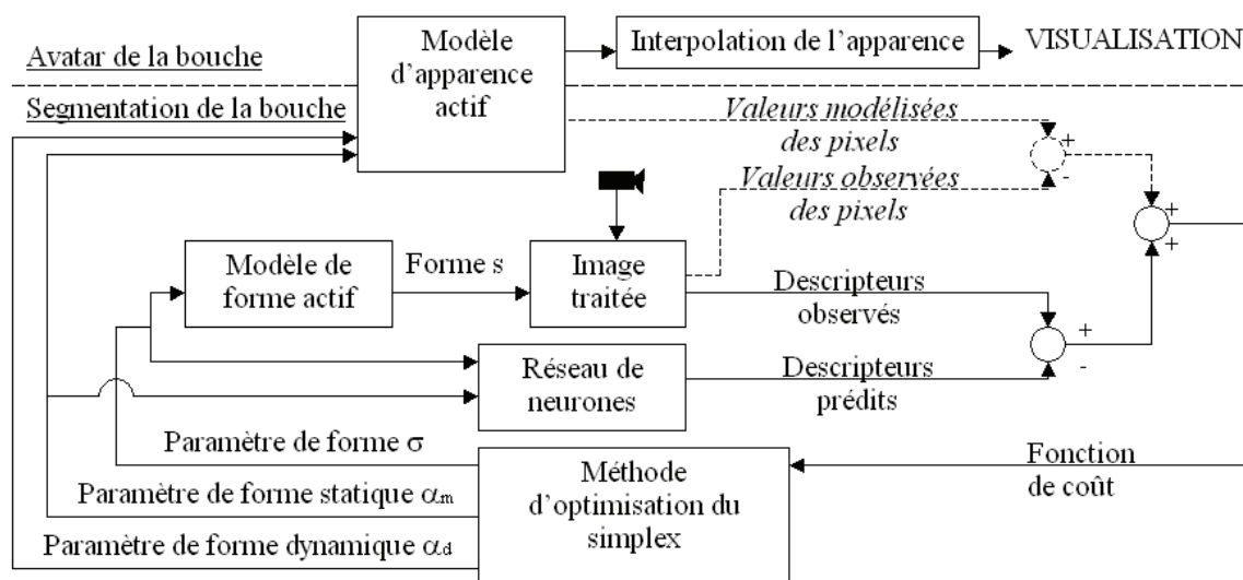
Figure 1.16 : Schéma de principe de l'algorithme proposé par (Gacon, 2005)
