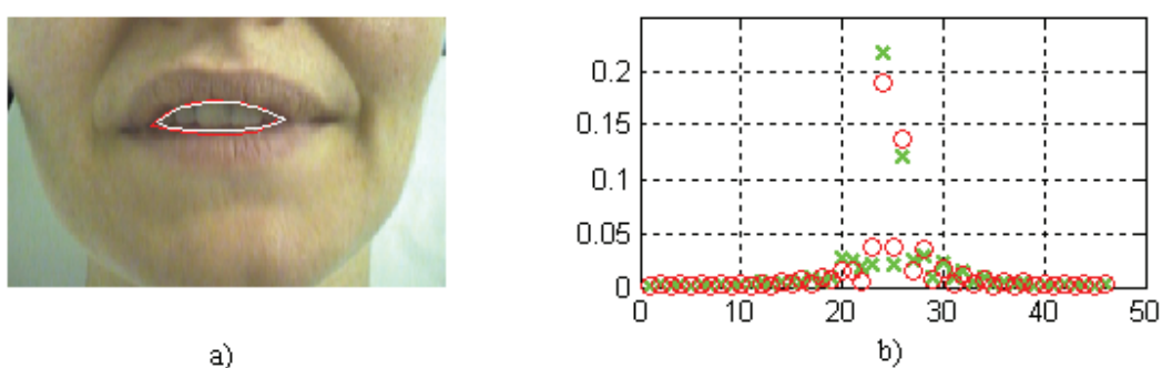
Figure 5.35 : Exemple de tracé de spectres d'amplitude normalisés des descripteurs de Fourier, pour \{k=-N_p/2+1, \dots, -1, 2, \dots, N_p/2\} , du contour interne de la vérité terrain et du contour obtenu par nos algorithmes de segmentation, a) Tracés de la vérité-terrain (blanc) et du résultat de la segmentation (rouge), b) Tracés des spectres d'amplitude normalisés pour la vérité-terrain (croix vertes) et pour le contour obtenu par segmentation (rond rouge).
