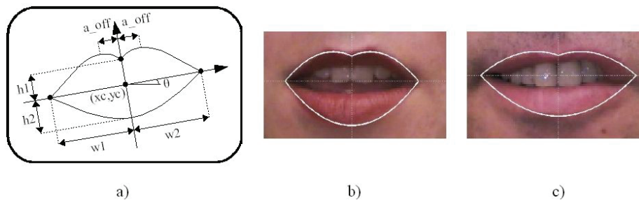
Figure 1.26 : Modèle de contour externe à 3 paraboles, a) Modèle paramétrique à 3 paraboles, b) et c) Exemples de convergence.
