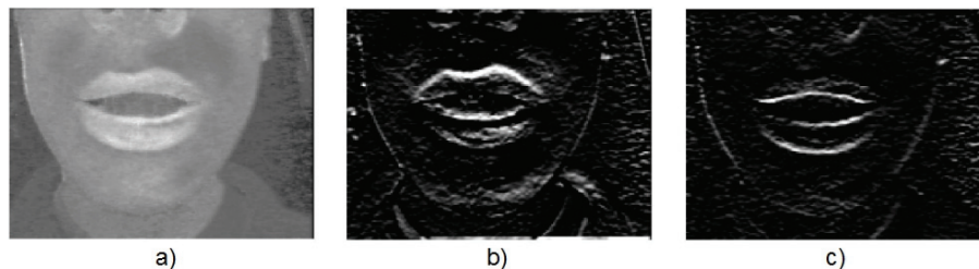
Figure 1.7 : Images des gradients R_{top} et R_{bottom} , a) image de R/G , b) R_{top} , c) R_{bottom} .
