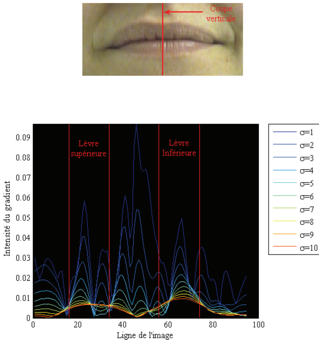
Figure 2.7 : Intensité des gradients \nabla L(x, y, t) de \hat{U} le long de la coupe centrale de l'image de bouche pour des valeurs de \sigma allant de 1 à 10.
