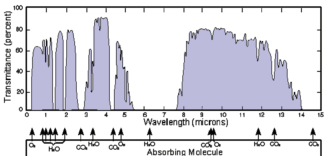
Figure 4.3 : Transmittance atmosphérique pour le domaine infrarouge avec une atmosphère standard aux États-Unis en 1976, au niveau de la mer, T=288\text{K} , taux d'humidité 46%, pression atmosphérique 1013 millibar, et sur un parcours d'un kilomètre horizontal. En abscisse, on donne la longueur d'onde en \mu\text{m} . En ordonnée, on donne la transmittance en %. Les gaz causant l'absorption sont également indiqués (Wikipedia, 2009).
