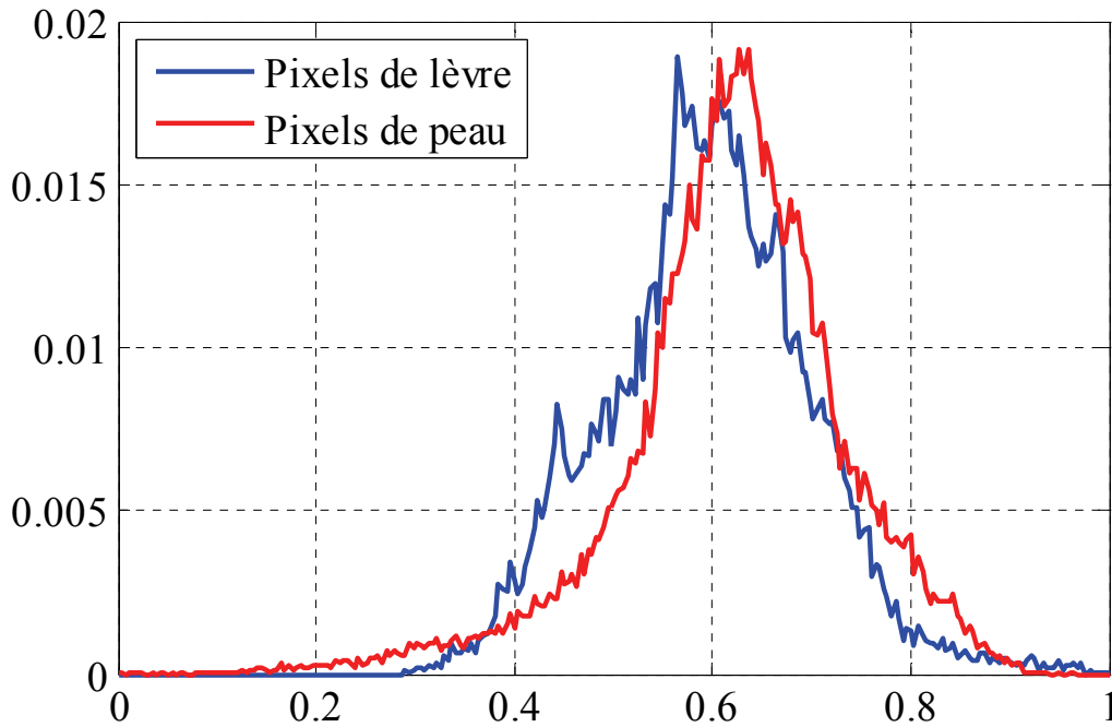
Figure 4.10 : Histogrammes normalisés des ensembles de pixels de la peau et des lèvres segmentés manuellement pour la modalité infrarouge.
