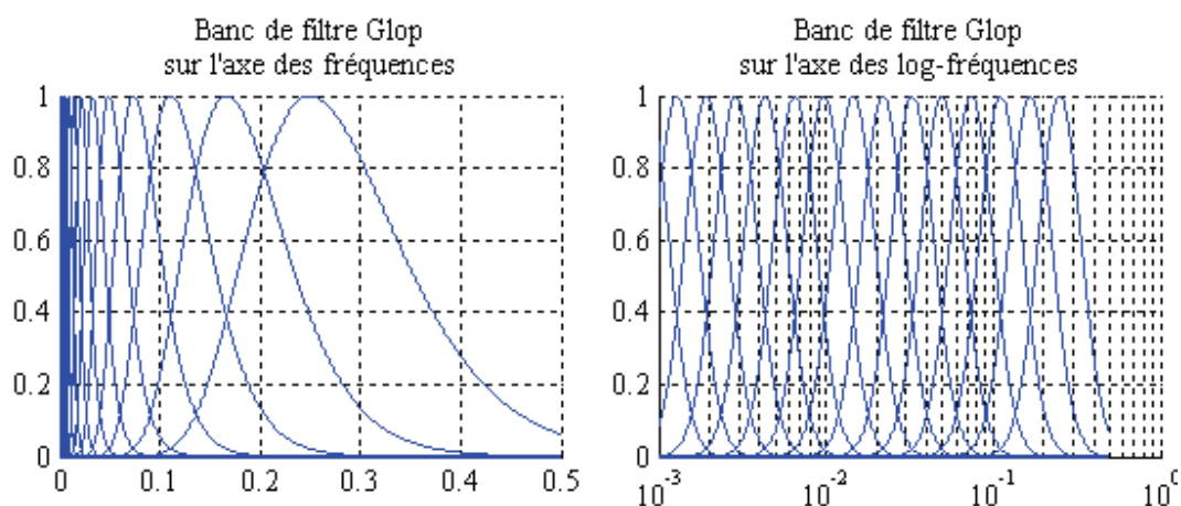
Figure 3.15 : Banc de filtres Glop en 1 dimension, à gauche nous avons tracé les profils des filtres sur l'axe des fréquences et à droite sur l'axe des log-fréquences. Les amplitudes des filtres ont été normalisées entre 0 et 1 pour améliorer la visualisation de la forme des filtres.
