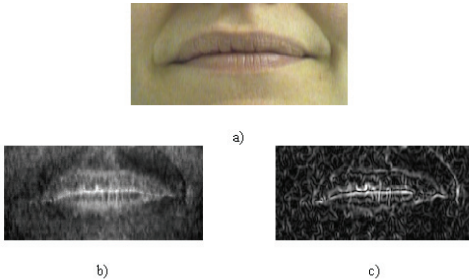
Figure 2.5 : Exemple de calcul du gradient de \hat{U} pour une image de bouche : a) Image de bouche, b) Teinte \hat{U} , c) Intensité du gradient de \hat{U} .
