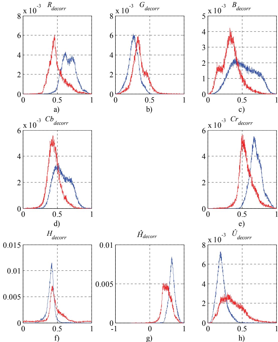
Figure 5.14 : Tracés des histogrammes des distributions des ensembles de pixels de la zone interne de la bouche (en rouge) et des lèvres (en bleu), a) R_{decorr} b) G_{decorr} c) B_{decorr} d) Cb_{decorr} e) Cr_{decorr} f) H_{decorr} g) \hat{H}_{decorr} et h) \hat{U}_{decorr} .
