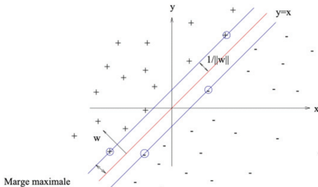
Figure 3.21 : Hyperplan optimal dans le cas d'un problème de séparation linéaire à 2 classes. En rouge est tracée la frontière de décision, les échantillons entourés en bleu sont les vecteurs de support. ( http://fr.wikipedia.org/wiki/Machine_a_vecteurs_de_support ).
