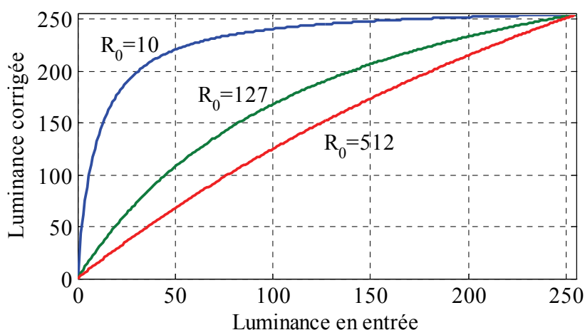
Figure 3.5 : Tracés des réponses d'un photorécepteur pour différentes valeurs de R_0 .
