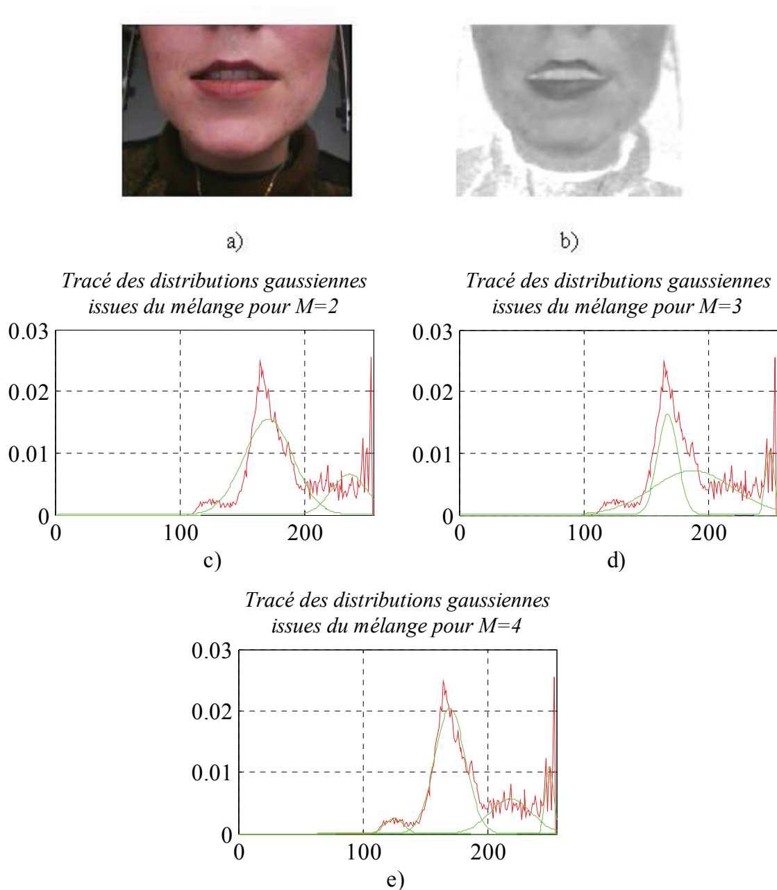
Figure 2.10 : Tracés des mélanges de gaussiennes pour M=[2,3,4] : a) Image d'entrée, b) Image de teinte \hat{U} , c) Mélange pour M=2 , d) Mélange M=3 , e) Mélange pour M=4 , en rouge, on donne l'histogramme de l'image dans \hat{U} , en vert, on donne les tracés des distributions gaussiennes issues des mélanges.
