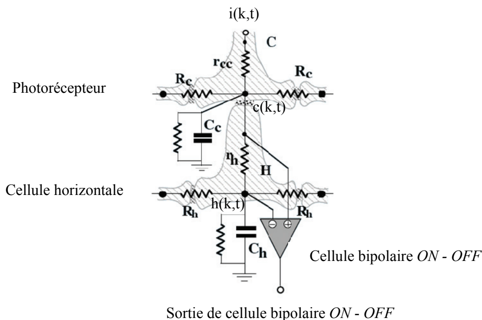
Figure 3.7 : Modélisation d'une triade synaptique (Hérault, 2001).
