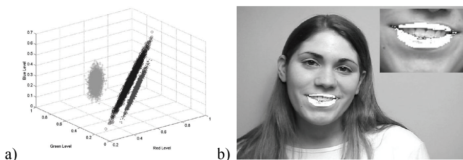
Figure 1.11 : Modélisation des classes de pixels de visage, de lèvre et de fond (Patterson, 2002), a) Estimation des distributions des pixels de visage, de lèvre, et de fond dans l'espace RGB , b) Exemple de segmentation labiale.
