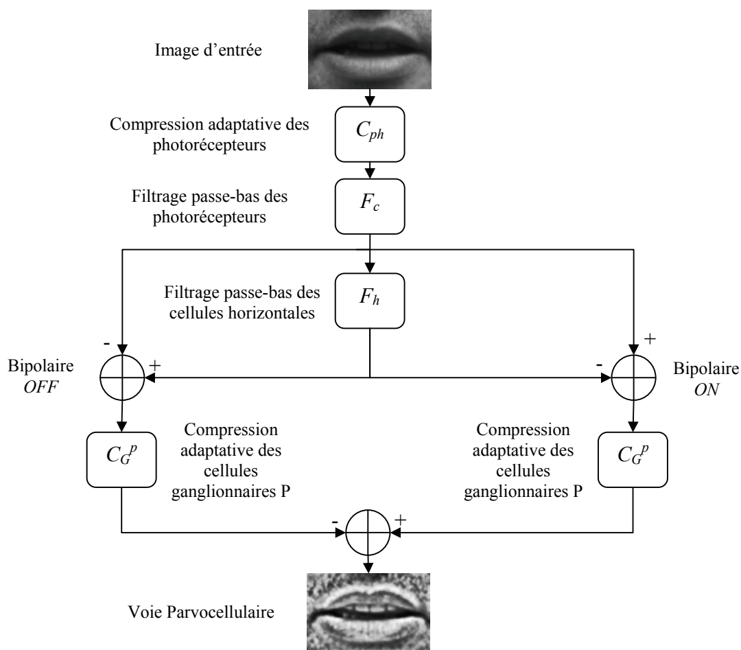
Figure 3.13 : Modélisation de la rétine pour l'analyse d'images statiques
