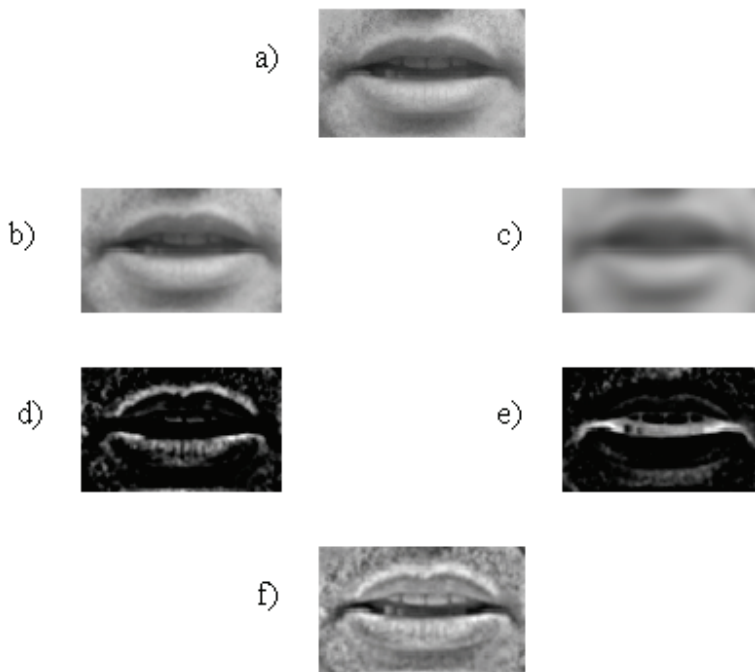
Figure 3.10 : Effet des différents réseaux de cellules de la PLE , a) image après compression adaptative, b) filtrage passe-bas des photorécepteurs, c) filtrage passe-bas des cellules horizontales, d) sortie des cellules bipolaires ON , e) sortie des cellules bipolaires OFF , f) sortie ON-OFF .
