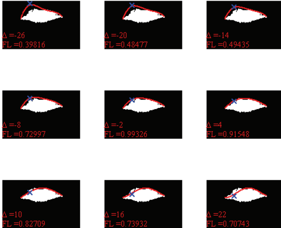
Figure 5.4 : Déformation de la courbe modélisant le contour C_{sup} avec deg_{sup}=4 sous l'action du déplacement d'un point de contrôle symbolisé par une croix bleue. On donne la somme FL des flux des gradients \gamma -normalisés \nabla_{norm}L(x, y, t) à travers la courbe ainsi que le déplacement \Delta par rapport à la position verticale d'origine du point de contrôle.
