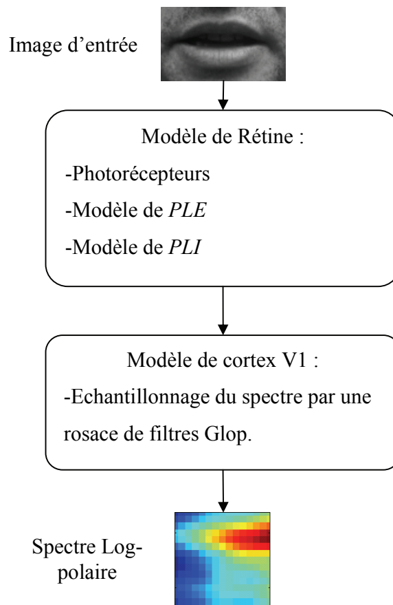
Figure 3.16 : Schéma global des traitements rétine+cortex V1
