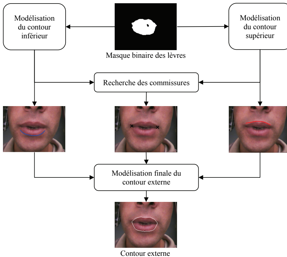
Figure 5.2 : Schéma bloc des étapes de modélisation du contour externe de la bouche à partir du masque binaire des lèvres.
