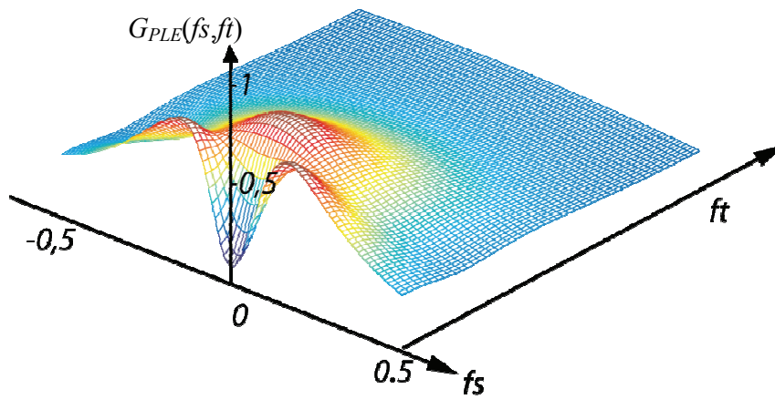
Figure 3.9 : Fonction de transfert G_{PLE}(f_s, f_t)
