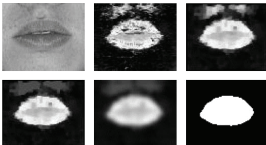
Figure 1.13 : Exemple de segmentation des lèvres (Liew, 2003). Du coin haut-gauche au coin bas-droit, image d'entrée, partition floue de la classe lèvre, partition après des opérations de morphologie mathématique, partition après application des contraintes de symétrie, partition après filtrage gaussien et enfin masque binaire des lèvres après seuillage.
