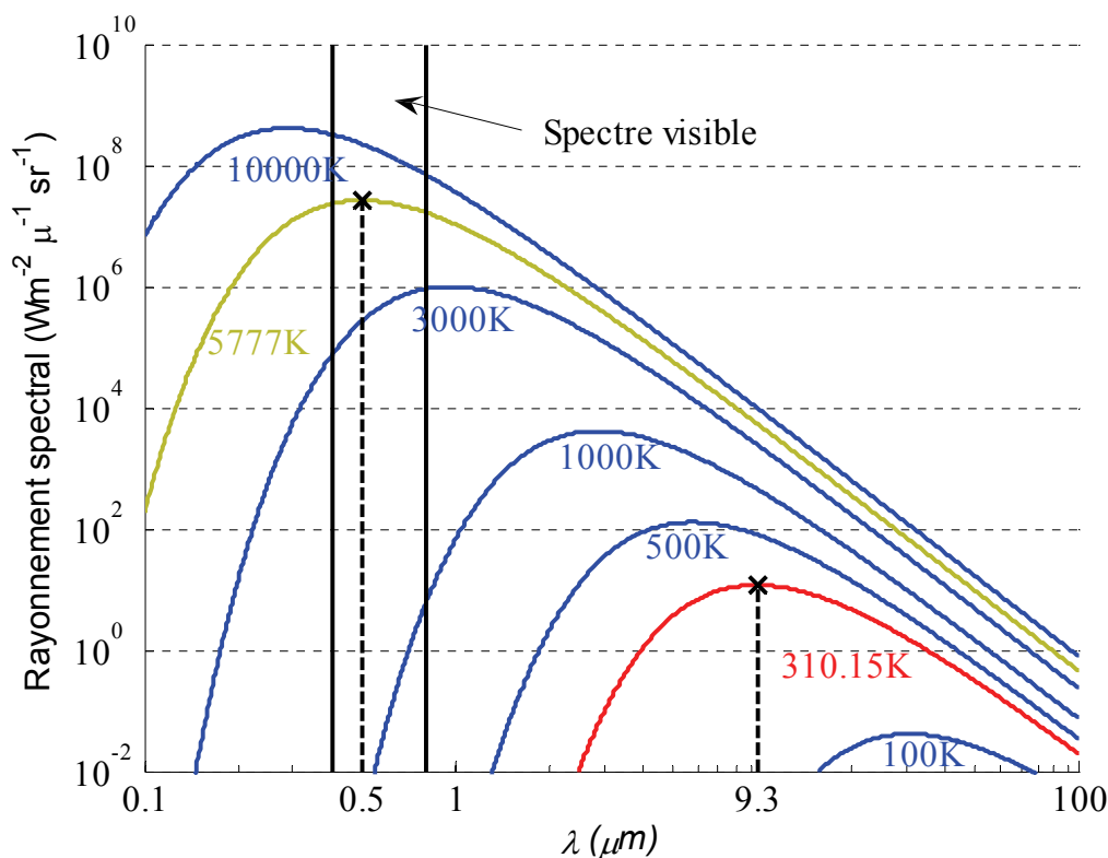
Figure 4.2 : Spectre de rayonnement de Planck pour différentes températures du corps noir. En rouge, nous avons tracé la courbe à T=310.15\text{K} ce qui correspond à la température du corps humain. En jaune, nous avons tracé la courbe du rayonnement pour T=5777\text{K} qui correspond approximativement à la température à la surface du soleil.
