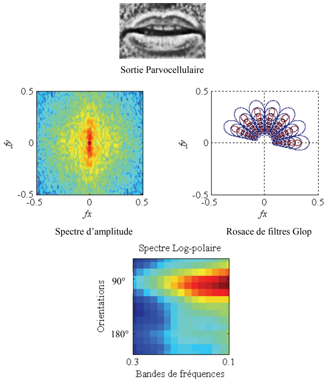
Figure 3.14 : Exemple de calcul d'un spectre Log-polaire. Le spectre d'amplitude de l'information visuelle, issue du modèle de rétine, est échantillonnée par une rosace de filtres Glop pour obtenir le spectre Log-polaire.
