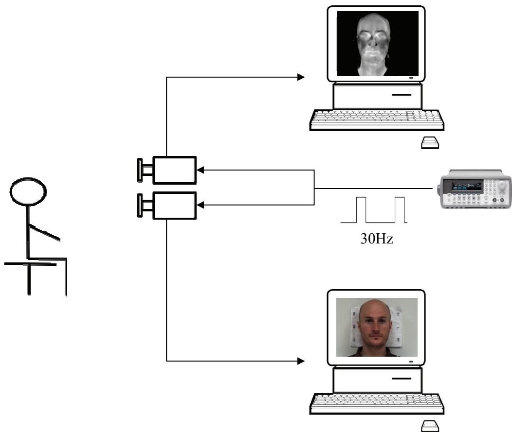
Figure 4.7 : Schéma du système d'acquisition de la base d'image de visage visible/infrarouge
