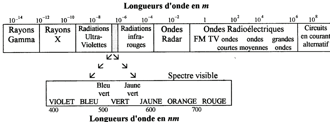
Figure 4.1 : Spectre électromagnétique
