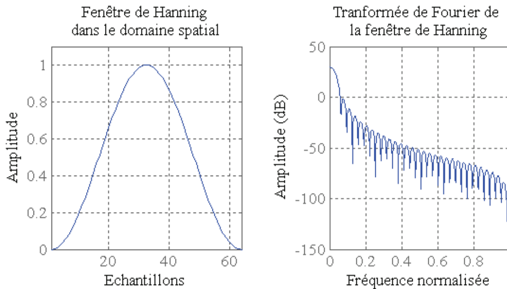
Figure 3.19 : Transformée de Fourier de la fenêtre de Hanning
