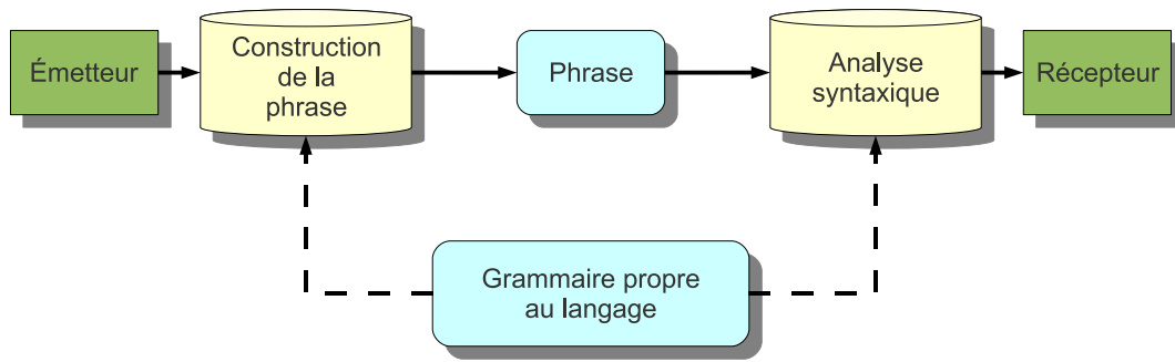
FIG. 3.1 – L'analyse syntaxique
