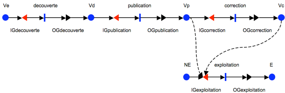
Figure 3.5 : Modélisation des interdépendances entre cycle de vie et comportement de l'attaquant avec l'hypothèse d'une découverte d'origine non malveillante
