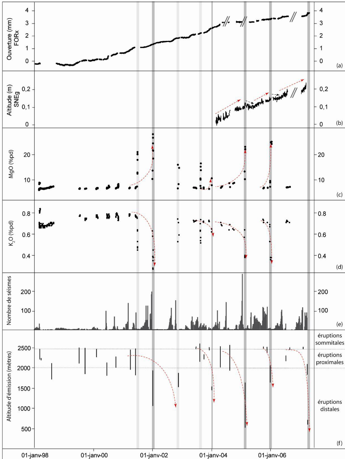
Figure 5.1 : Comparaison entre l'évolution (a) de l'ouverture de la fracture FORx (corrégée « des éruptions ») (b) de l'altitude du point SNEg (corrégée « des éruptions ») (c) de la teneur en MgO (%pds) (d) et K 2 O (%pds) des laves émises (e) du nombre de séismes journaliers (f) et de l'altitude des fissures éruptives au cours de la période 1998-2007. Les colonnes en gris foncé représentent les éruptions distales à océanites et les colonnes en gris clair les éruptions à basaltes à olivines. Les flèches représentent les différents cycles définis dans le texte.
