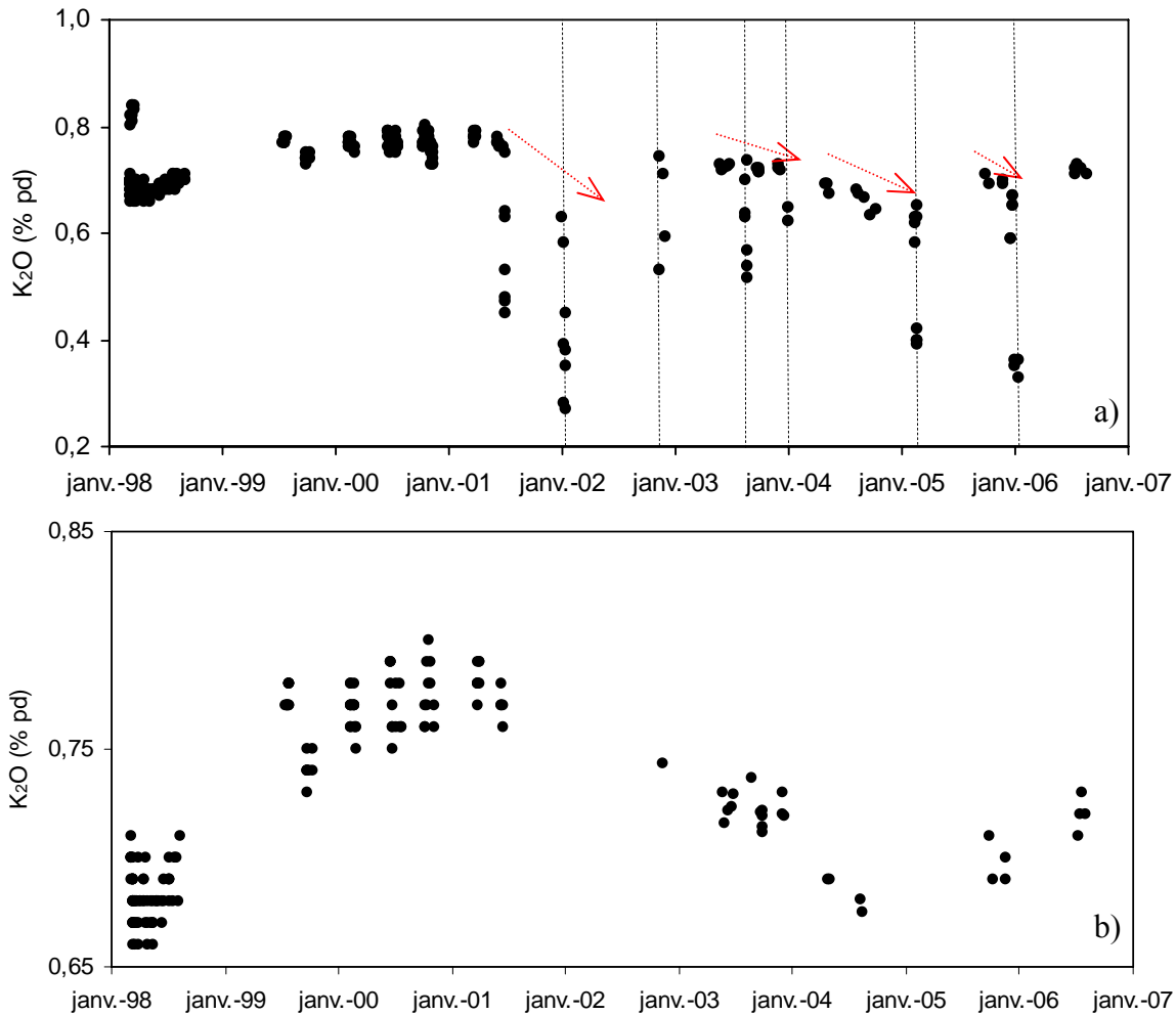
Figure 4.35 : (a) Evolution du K_2O (%pds) en fonction du temps pour l'ensemble des laves émises au Piton de La Fournaise depuis 1998 et (b) pour les laves dont les teneurs en MgO sont inférieures à 7,2. Les pointillés correspondent aux éruptions à océanites et basaltes à olivine.
