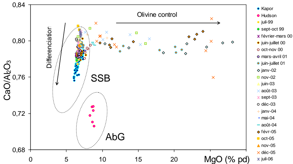
Figure 4.7 : Diagramme \text{CaO}/\text{Al}_2\text{O}_3 vs \text{MgO} des basaltes émis par le Piton de La Fournaise depuis 1998.
