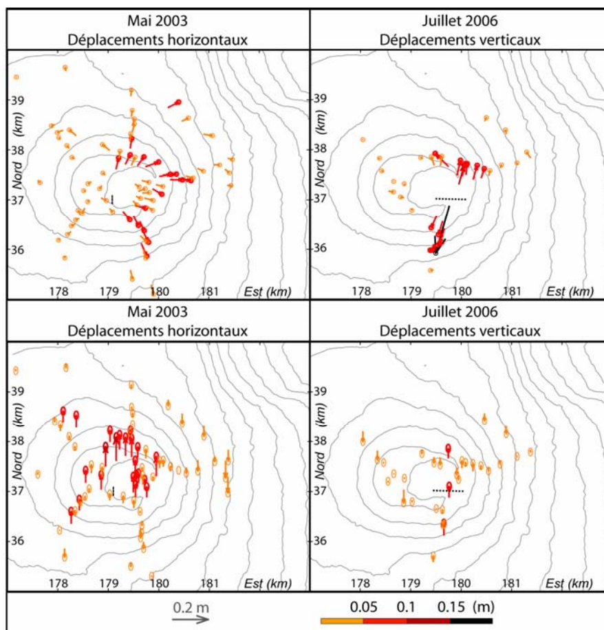
Figure 2.54: Déplacements associés aux éruptions sommitales de mai 2003 (campagnes GPS d’avril et juin 2003) et juillet 2006 (campagnes GPS de mars et juillet 2006). Localisation des fissures éruptives en pointillé. (Coordonnées en Gauss Laborde Réunion).
