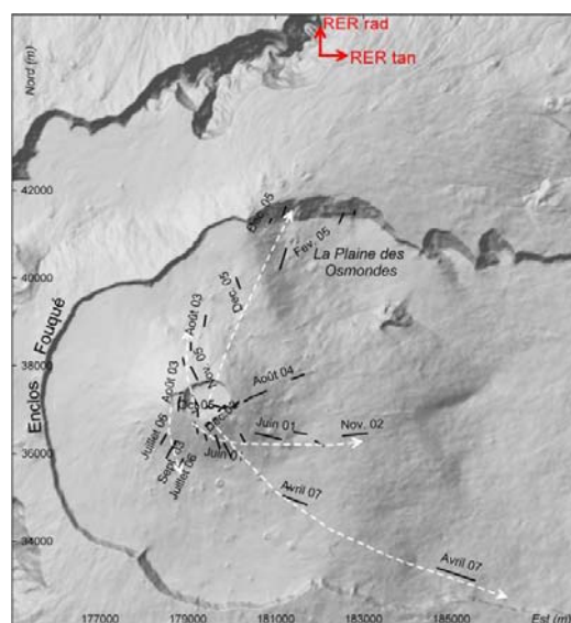
Figure 2.60 : Localisation de la station RER et des fissures éruptives associées aux éruptions étudiées. Les flèches blanches représentent les trajets préférentiels d'alimentation du Piton de La Fournaise.
