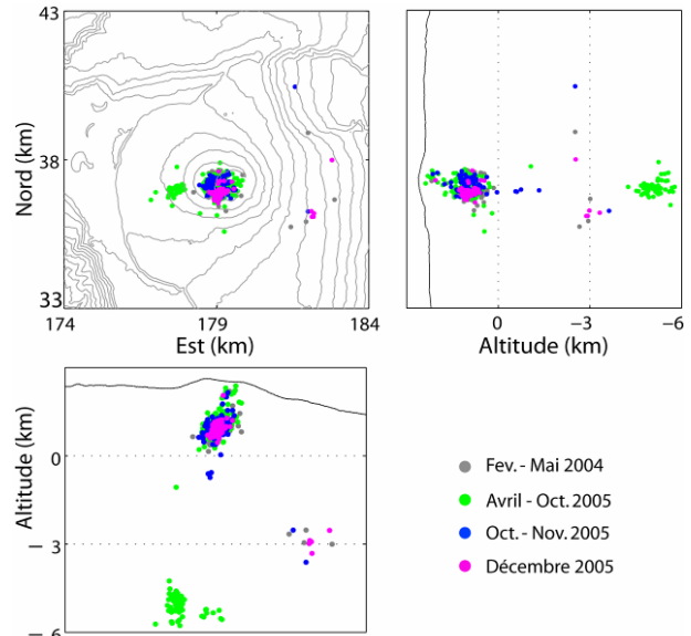
Figure 2.44 : Localisation de la sismicité pré éruptive. (Coordonnées en Gauss Laborde Réunion). Localisation des hypocentres, d'après Valérie Ferrazzini, communication personnelle.
