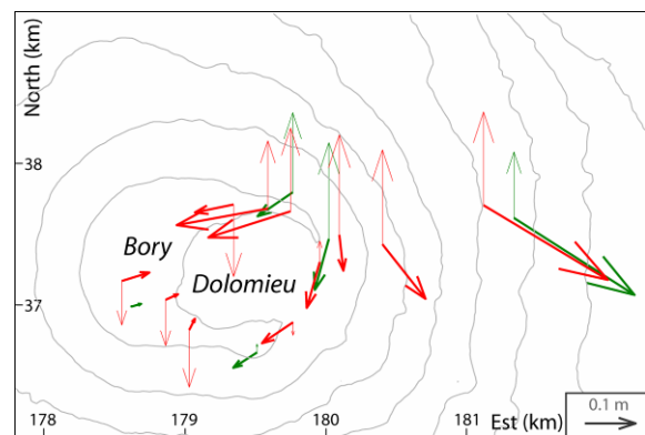
Figure 2.53 : Comparaison entre les déplacements mesurés entre les campagnes GPS ponctuel (rouge) du 8/12/05 et du 27/01/2006 et les déplacements mesurés par les GPS permanents le 26/12/06. Traits gras : déplacements horizontaux Traits fins : déplacements verticaux
