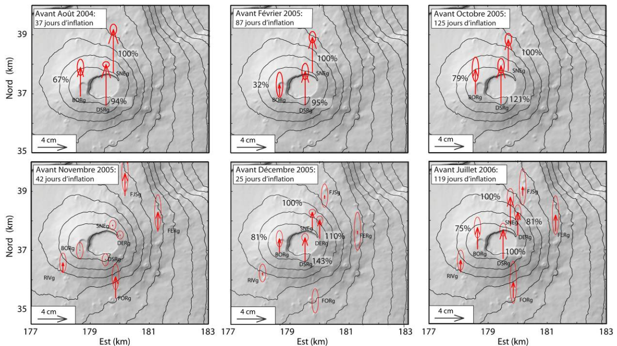
Figure 2.38 : Déplacements verticaux enregistrés sur l'ensemble du réseau GPS permanent lors des phases pré éruptives depuis le début de l'implantation du réseau en 2004. (Coordonnées en Gauss Laborde Réunion). Le réseau n'étant opérationnel qu'à partir de février 2004 nous ne disposons pas de l'intégralité des déplacements pré éruptifs associés à l'éruption de mai 2004.
