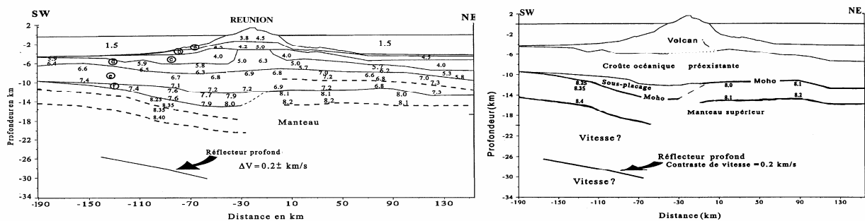
Figure 1.6 : Gauche : modèle de répartition des vitesses des ondes P (en \text{km.s}^{-1} ) pour l’île de la Réunion. Droite : modèle structural issu de l’interprétation des données sismiques (Driad, 1997).
