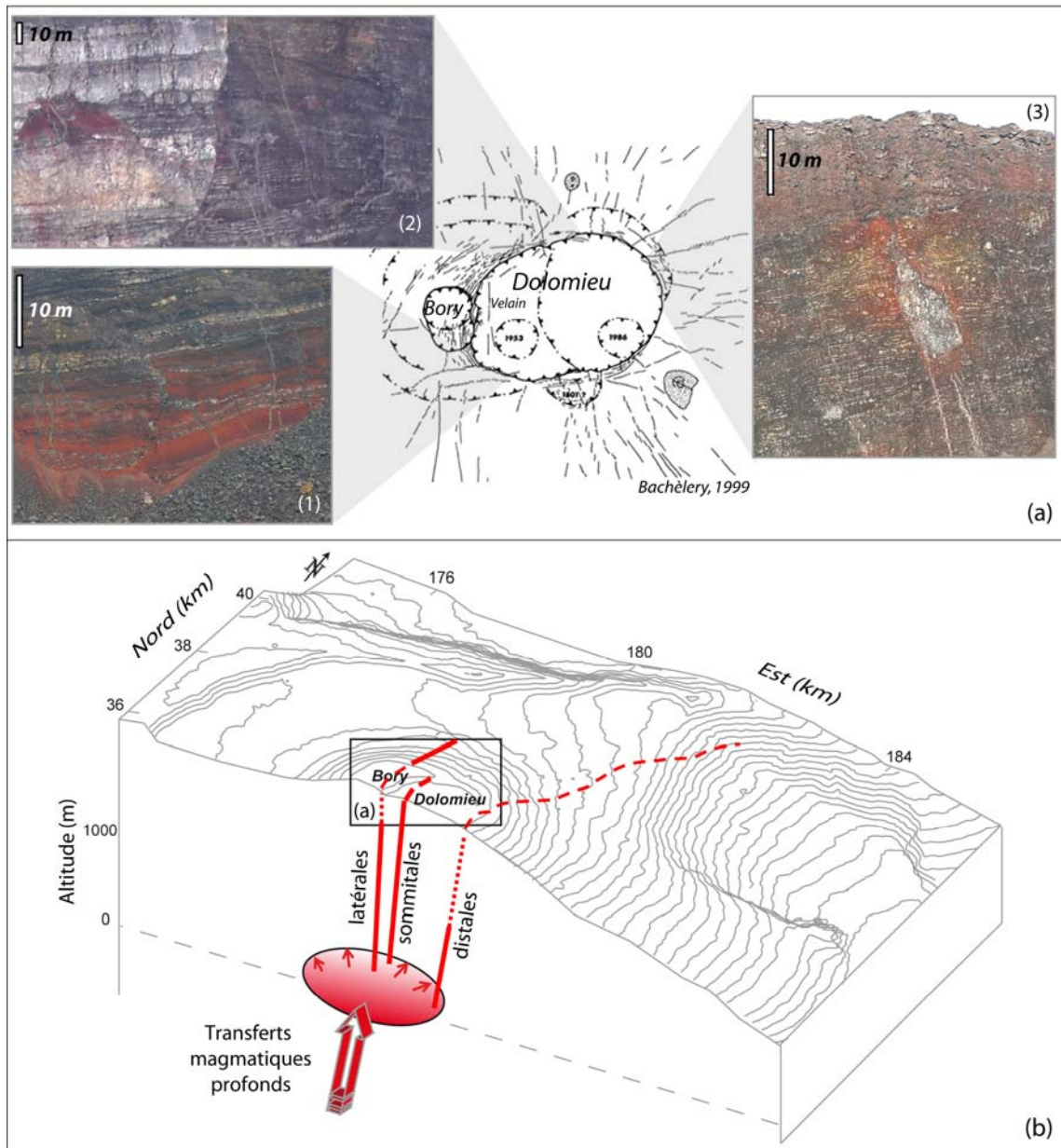
Figure 5.3 : (a) Cartographie des fractures et limites cratériques de la zone sommitale du Piton de la Fournaise (d'après Bachèlery, 1999) et photographies des remparts. (b) Système d'alimentation superficiel du Piton de La Fournaise.
