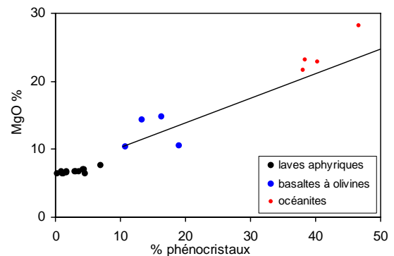
Figure 4.8 : Evolution de la teneur en \text{MgO}\% en fonction du pourcentage de cristaux de la roche, et droite de mélange calculée. La méthode et les paramètres utilisés pour les calculs de mélange sont reportés en annexe 6.
