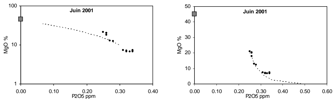
Figure 4.28 : Relation entre la teneur en MgO (%) et P 2 O 5 (ppm) des basaltes émis en juin 2001 avec la courbe théorique de mélange à gauche et la lignée d'évolution par cristallisation fractionnée à droite. La méthode et les paramètres utilisés pour les calculs de mélange et de cristallisation fractionnée sont en annexe 6.
