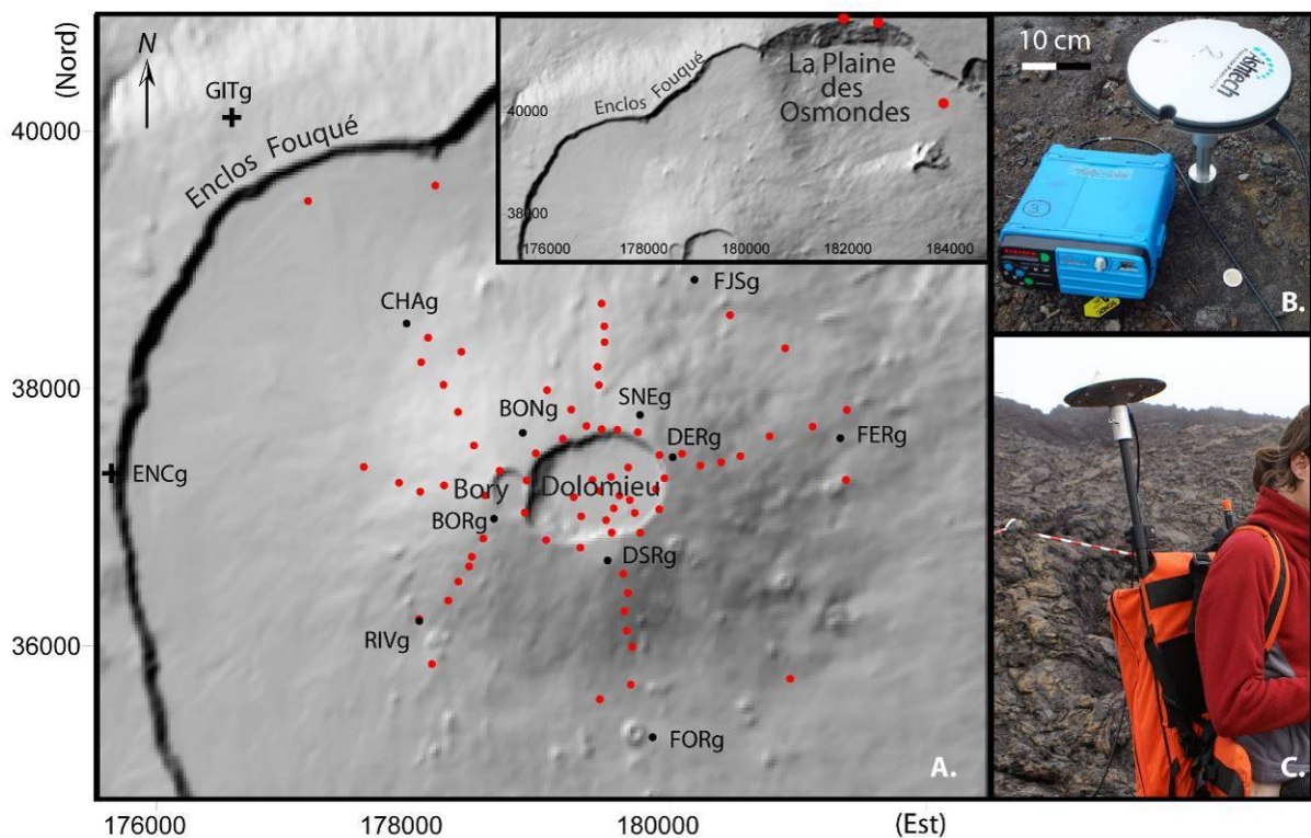
Figure 2.3 : (a) Disposition du réseau GPS implanté par l'OVPF. Points noirs : GPS permanents, Points rouges : Tiges réitérées par mesures ponctuelles, Croix noires : GPS de référence. (coordonnées en Gauss Laborde Réunion). (b) Photographie d'un récepteur et d'une antenne GPS Ashtech. (c) Mode cinématique des mesures GPS
