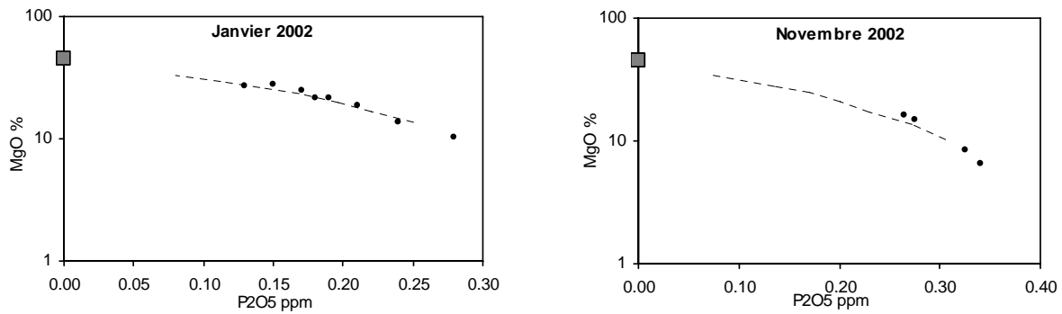
Figure 4.27 : Relation entre la teneur en MgO (%) et P 2 O 5 (ppm) des basaltes émis en janvier 2002 (à gauche) et novembre 2002 (à droite). En pointillé les courbes de mélange calculées. La méthode et les paramètres utilisés pour les calculs de mélange sont en annexe 6.
