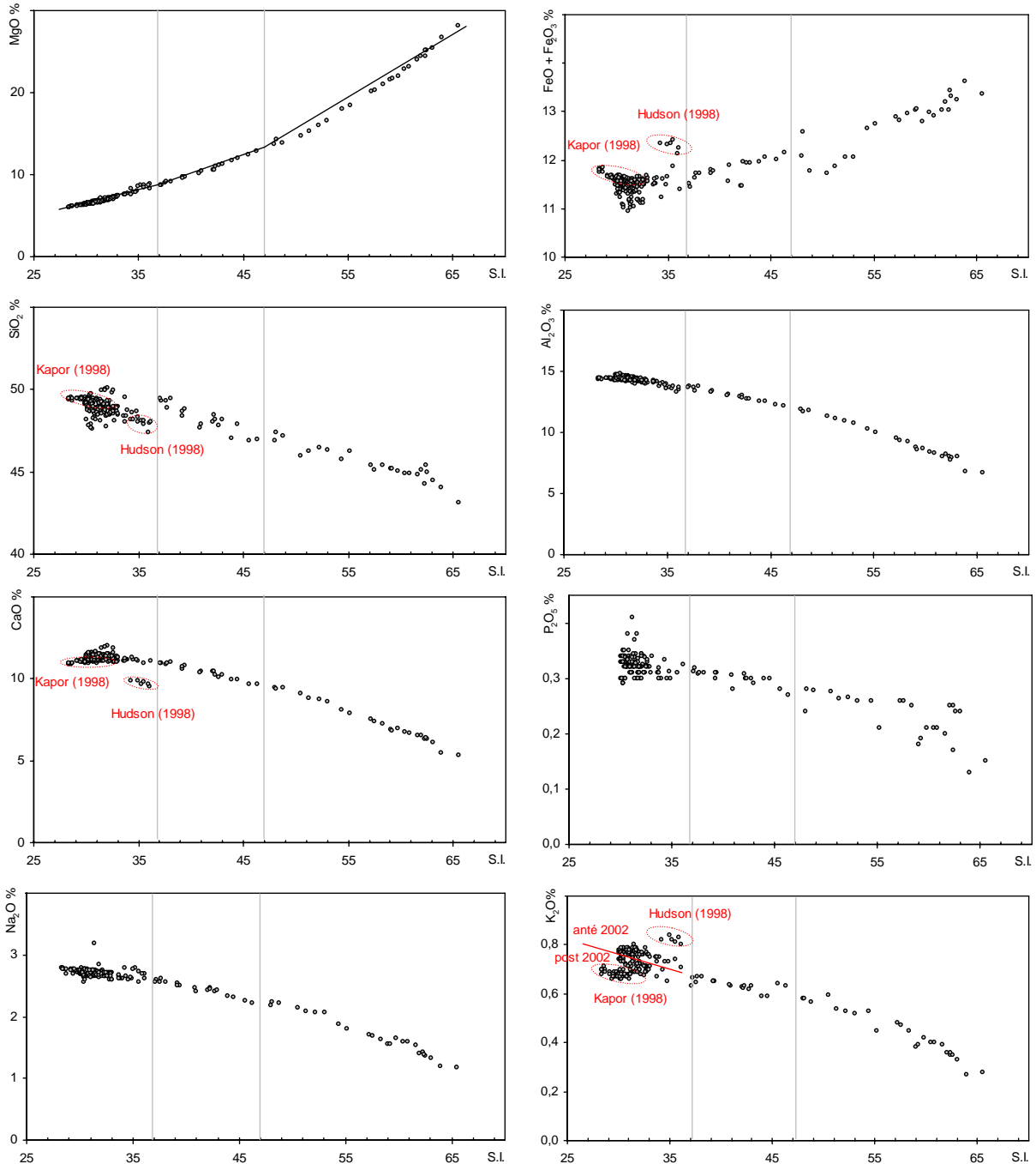
Figure 4.12 : Evolution de la teneur en MgO%, FeO+Fe 2 O 3 %, SiO 2 %, P 2 O 5 % et K 2 O% des basaltes émis au Piton de La Fournaise entre 1998 et 2005 en fonction du SI
