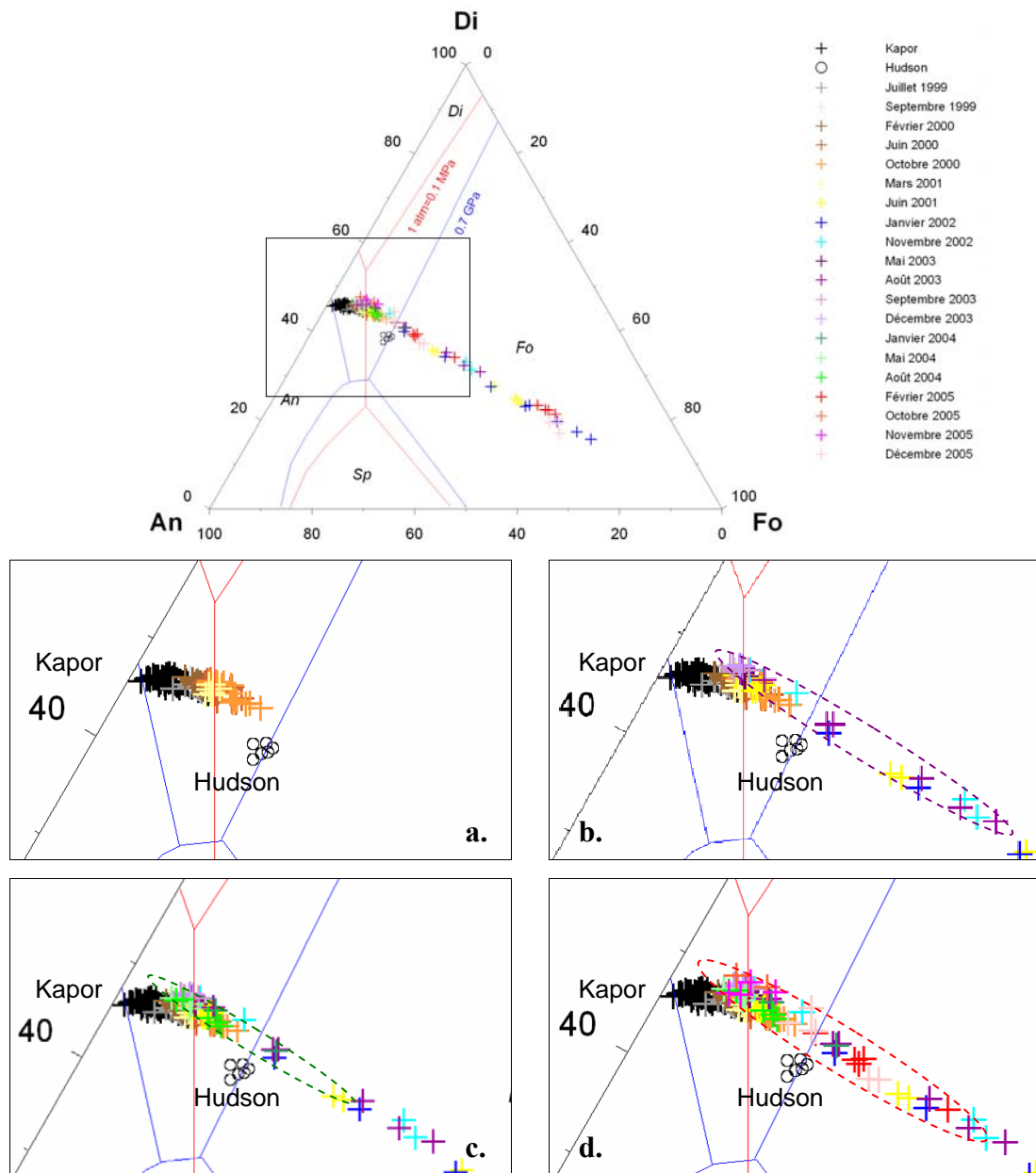
Figure 4.11 : Composition des laves émises au Piton de La Fournaise dans le système Forstérite - Diopside - Anorthite (Lignes cotectiques et pôles calculés d'après Presnall et al., 1978) . Zoom sur les périodes (a) 1998 à 2001, (b) 1998 à 2003, (c) 1998 à 2004, (d) 1998 à 2005.
