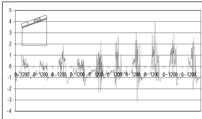
Figure 38 : Résidus (mesure-modèle) de la température d'air de la zone mi-haute (zone 5 - T_{toile} forcée)
