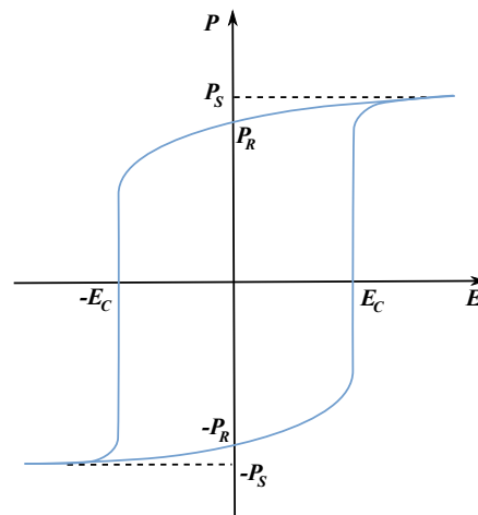
FIGURE III.2 – Cycle d'hystérésis de la polarisation P en fonction du champ électrique E pour un matériau ferroélectrique
