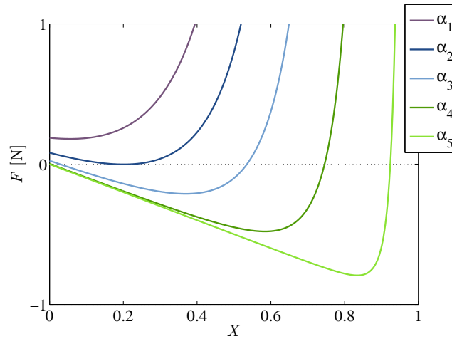
FIGURE III.12 – Tracé de la somme des forces en fonction du déplacement relatif pour différentes valeurs de \alpha
