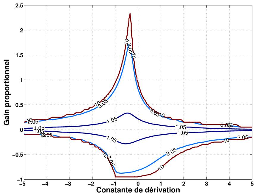
FIGURE 3.8 – Résultats relatifs à la commande proportionnelle dérivée. Les courbes de niveau de \rho en fonction du couple (T_D, k_P) . \rho est minimal et égal à 1 pour un k_P nul, autrement lorsque le contrôleur est off. Le rendement absolu augmente d'une manière trop importante aux limites du domaine de stabilité des paramètres T_D et k_P .
