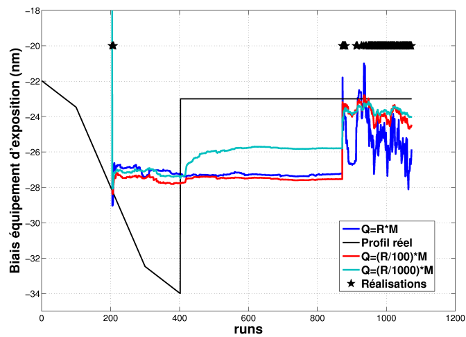
FIGURE 5.12 – Résultats de la simulation ( \sigma_\varepsilon^2 = 3 , \rho = 1 ). L'évolution de l'estimation du biais y_{sc} relatif à un équipement d'exposition donné pour plusieurs configurations du filtre de Kalman : 1/R = 3 & Q = RM en bleu, 2/R = 3 & Q = \frac{R}{100}M en rouge, et 3/R = 3 & Q = \frac{R}{1000}M en vert. Les étoiles noires indiquent les runs où le réticule est utilisé.
