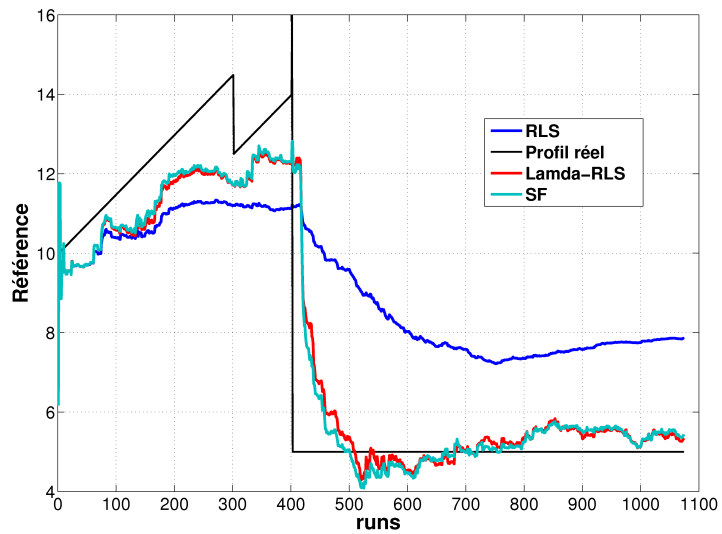
FIGURE 5.5 – Résultats de la simulation ( \sigma_\varepsilon^2 = 3 , \rho = 1 ). L'estimation de y_{reference} pour trois variantes des moindres carrés : 1/ Les moindres carrés classiques RLS en bleu, 2/l'algorithme \lambda - RLS avec \lambda = 0.99 en rouge et 3/ le SF ( \lambda_{sc} = \lambda_c = 0.99 ) en vert.
