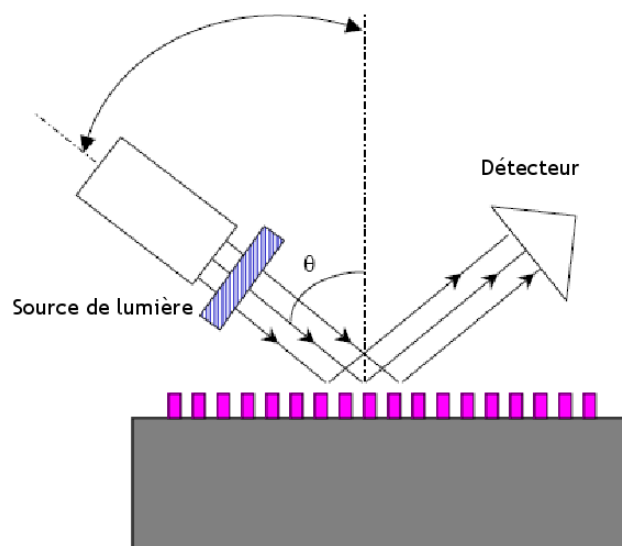
FIGURE 1.9 – Configuration de la scattérométrie 2 – \theta : Une seule longueur d'onde est utilisée ; l'angle d'incidence est variable. Seul l'ordre 0 de la lumière diffractée est collectée par le détecteur.
