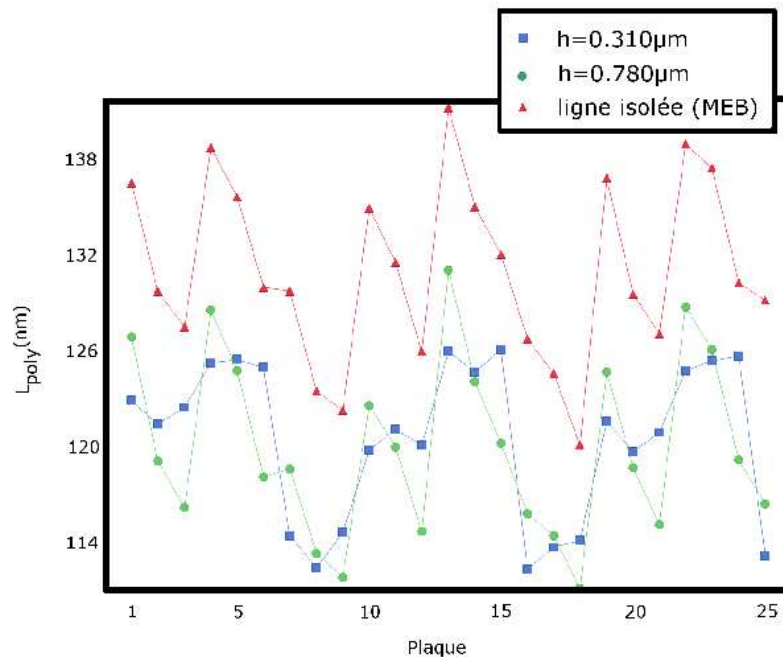
FIGURE 4.25 – Résultats du plan d'expérience au niveau de la mesure en ligne de la longueur du polysilicium : Dans l'espace de variation de la dose d'énergie et du \sigma_{inner} , le motif isolé et celui dont le pas h est égal à 0.780\mu\text{m} évoluent d'une manière équivalente. De ce point de vue, le motif dense ( h = 0.310\mu\text{m} ) est un intrus.
