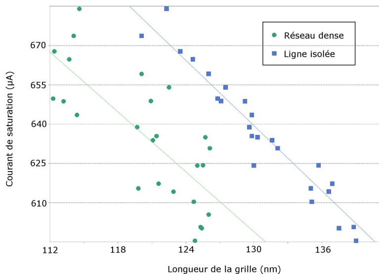
FIGURE 4.24 – Caractéristique I_{on} = f(L_{poly}) pour les transistors NMOS courts ( 0.13\mu\text{m} ). La variation du biais iso-dense \Delta implique la perte de la corrélation entre la longueur des lignes denses et les paramètres électriques à l’instar de I_{on} : R^2 = 59\% . La longueur des lignes isolées demeure corrélée au courant I_{on} ( R^2 = 92\% ).
