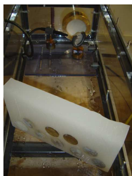
FIG. 2.10 – Photo de l'absorbant acoustique en paraffine lesté par du laiton.
