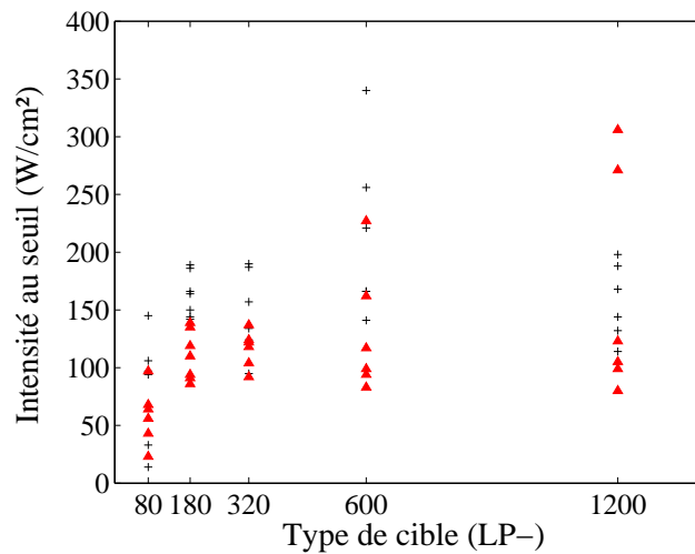
FIG. 3.15 – Influence de la granulométrie de la cible sur les seuils de cavitation pour des excitations mono- (croix noires) et bi-fréquentielle (triangles rouges).
