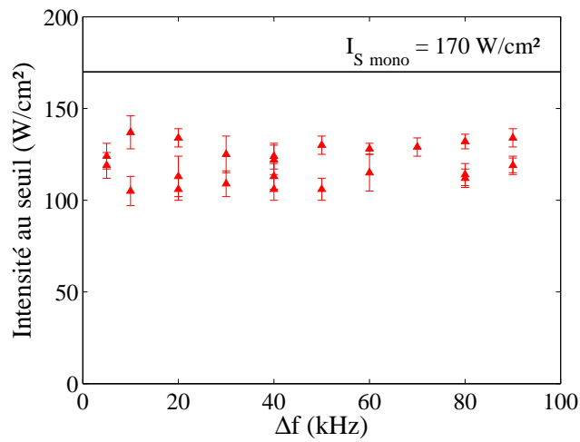
FIG. 3.13 – Seuils de cavitation en fonction de \Delta f pour des mesures dans des conditions expérimentales correspondant à un seuil nominal I_{S\ mono} = 170\text{ W/cm}^2 . Les barres d'erreurs correspondent aux incertitudes de mesures de seuil comme elles ont été définies au chapitre précédent (cf §2.4.3.2).
