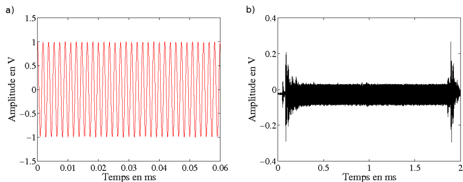
FIG. 2.12 – Signal temporel monofréquentiel a) généré (zoom) et b) un exemple de signal capté par l'hydrophone RESON .
