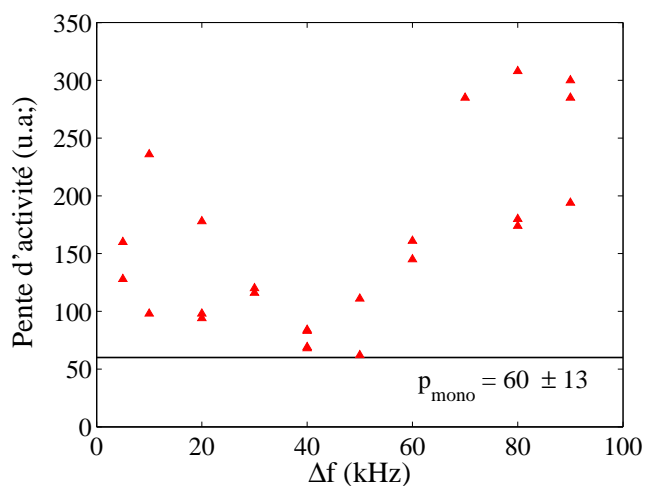
FIG. 3.14 – Pentes de l'activité au-delà du seuil en fonction de \Delta f . La pente monofréquentielle correspondante est p_{mono} = 60 \pm 13 .
