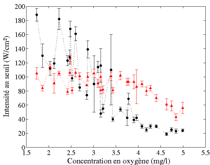
FIG. 3.2 – Évolution des seuils de cavitation monofréquentiel (ronds noirs) et bifréquentiel (triangle rouge) en fonction de la concentration en oxygène dissout dans l'eau. Les barres d'erreur montrent les valeurs minimale et maximale pour une série de 5 tirs de mesures.
