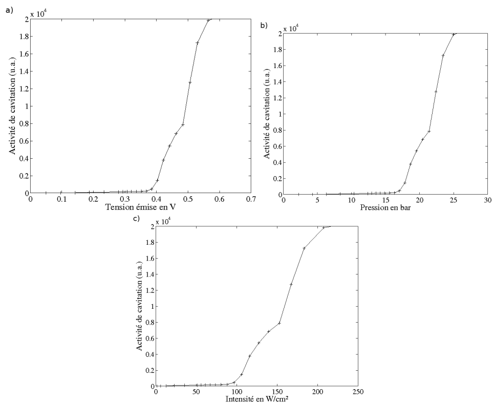
FIG. 2.22 – Activité de cavitation en fonction de a) la tension émise (en V) par le générateur de fonction, b) la pression au foyer (en bar) et c) l'intensité acoustique (en W/cm^2 ) évaluée au foyer en l'absence de cible.
