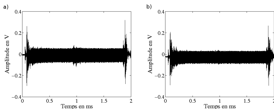
FIG. 2.11 – Signal temporel capté par l'hydrophone : a) en l'absence et b) en présence de l'absorbant.
