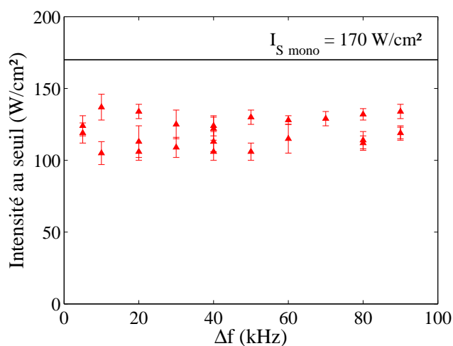
FIG. 3.13 – Seuils de cavitation en fonction de \Delta f pour des mesures dans des conditions expérimentales correspondant à un seuil nominal I_{S\ mono} = 170\ W/cm^2 . Les barres d'erreurs correspondent aux incertitudes de mesures de seuil comme elles ont été définies au chapitre précédent (cf §2.4.3.2).
