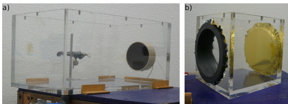
FIG. 4.3 – Cuves réalisées pour les essais de thromolyse : a) la cuve externe et b) la cuve interne.
