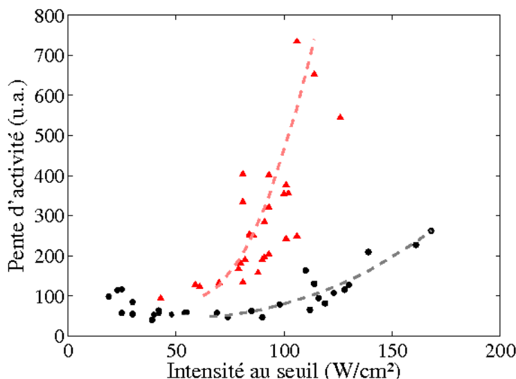
FIG. 3.7 – Pentés d'activité au-delà du seuil en fonction du seuil pour les excitations monofréquentielle (ronds noirs) et bifréquentielle (triangles rouges).
