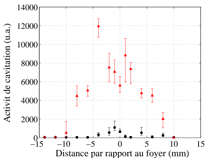
FIG. 3.10 – Activité de cavitation pour une excitation mono- (ronds noirs) et bifréquentielle (triangles rouges) en fonction de la position de la cible aux alentours du foyer le long de l'axe acoustique pour une intensité de 354 \text{ W/cm}^2 . Les barres d'erreurs montrent le minimum et le maximum obtenus pour chaque série de 5 tirs.
