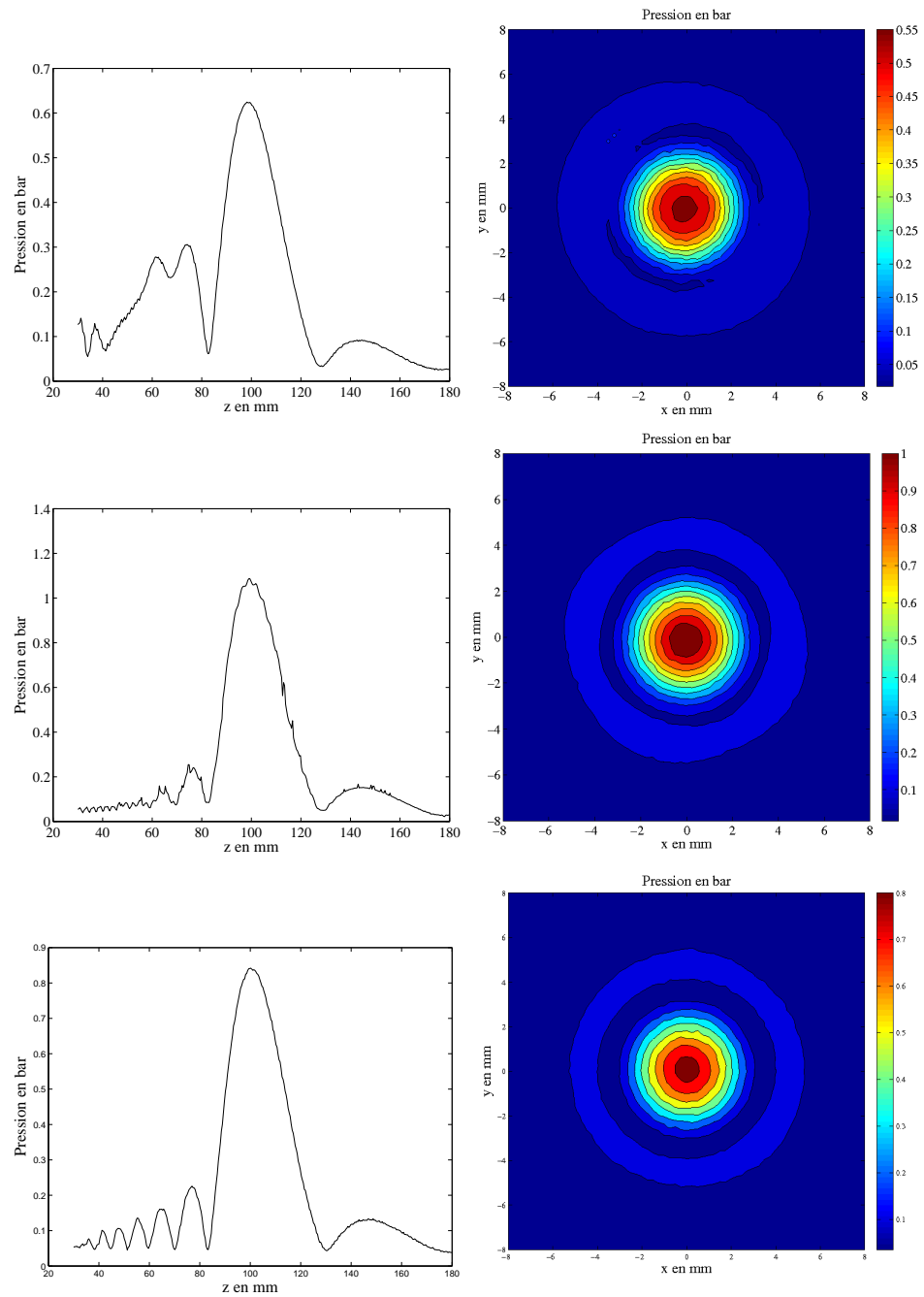
FIG. 2.7 – Champ de pression : à gauche le long de l'axe acoustique z et à droite dans le plan focal xy ; pour les transducteurs : en haut tx\_ceramique ; au milieu tx\_LB1 et en bas tx\_LB2 .
