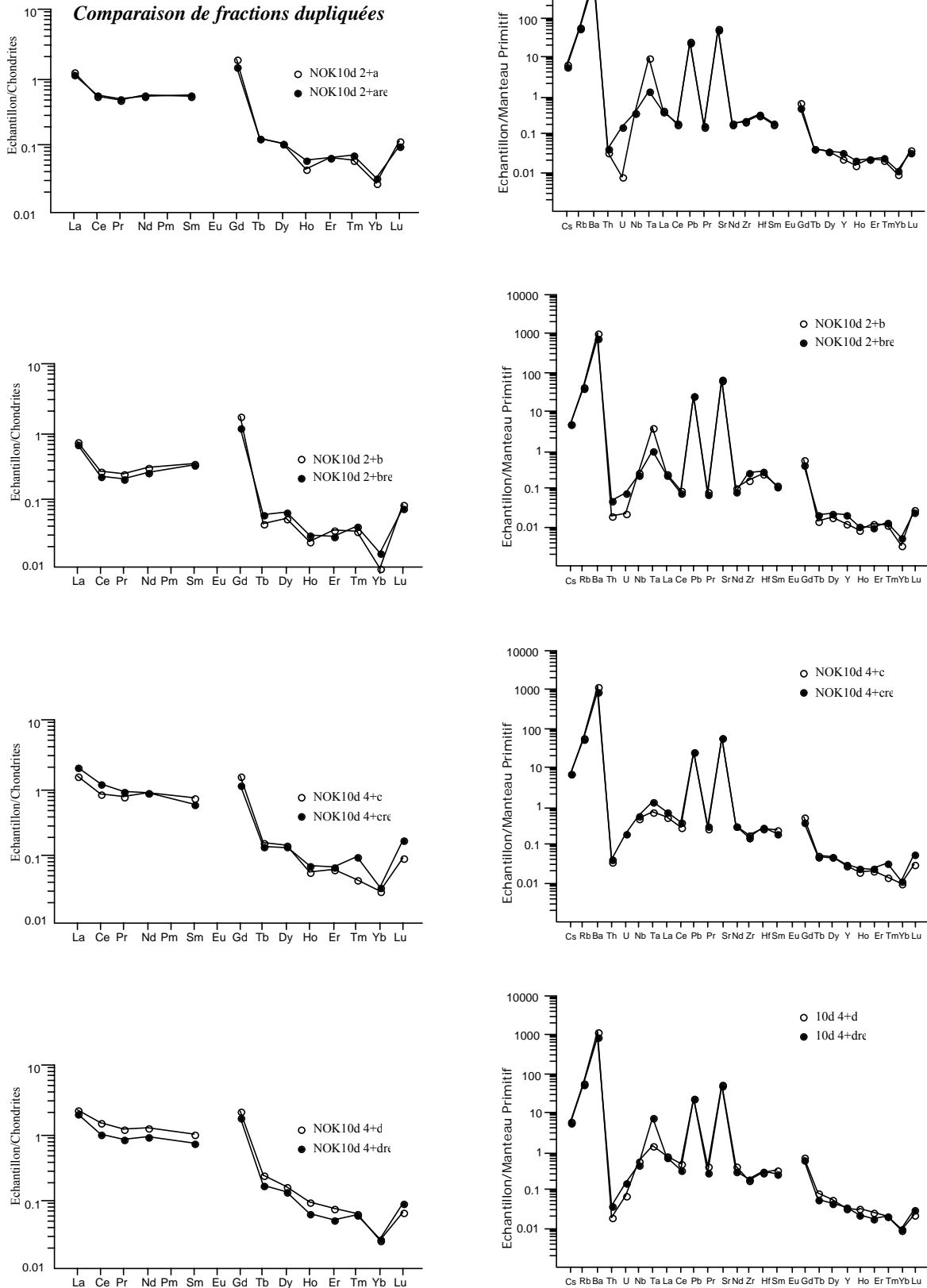
Figure A-7 : Comparaisons entre des données obtenues à l'ICP-MS de l'ISTEEM (Université Montpellier II) à un an d'intervalle sur des mêmes fractions de phengites. Pour les terres rares légères et moyennes, les données sont très reproductibles. La reproductibilité sur les terres rares lourdes est de moins bonne qualité, ce qui peut être expliqué par le fait qu'elles sont présentes en très faible concentration dans les phengites analysées, par conséquent l'erreur sur la mesure est plus importante. Globalement les différences au niveau des terres rares sont attribuées surtout à l'inhomogénéité des poudres (par exemple la différence importante en Tm pour l'échantillon NOK10d 4+c). Par contre on note des différences importantes au niveau des concentrations en Ta et U. Les données en Ta et U ne sont donc pas prises en considération dans la discussion des résultats.
