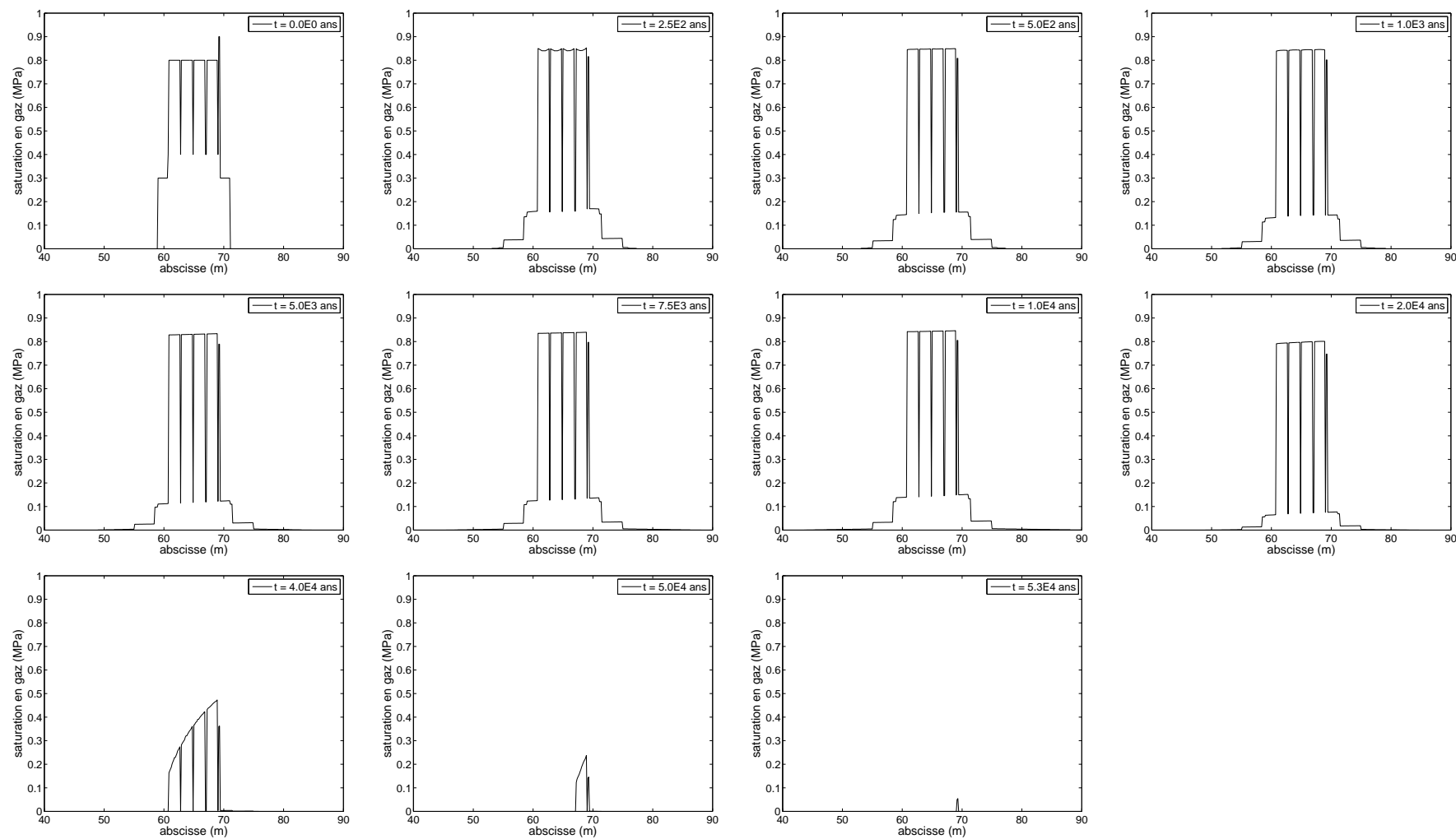
FIGURE 8.7 – Profils de la saturation en gaz en x = 103 m aux différents temps d’observation. L’abscisse 0 m correspond au bas du domaine ( z = 0 m) et l’abscisse 130 m correspond au haut du domaine ( z = 130 m).
