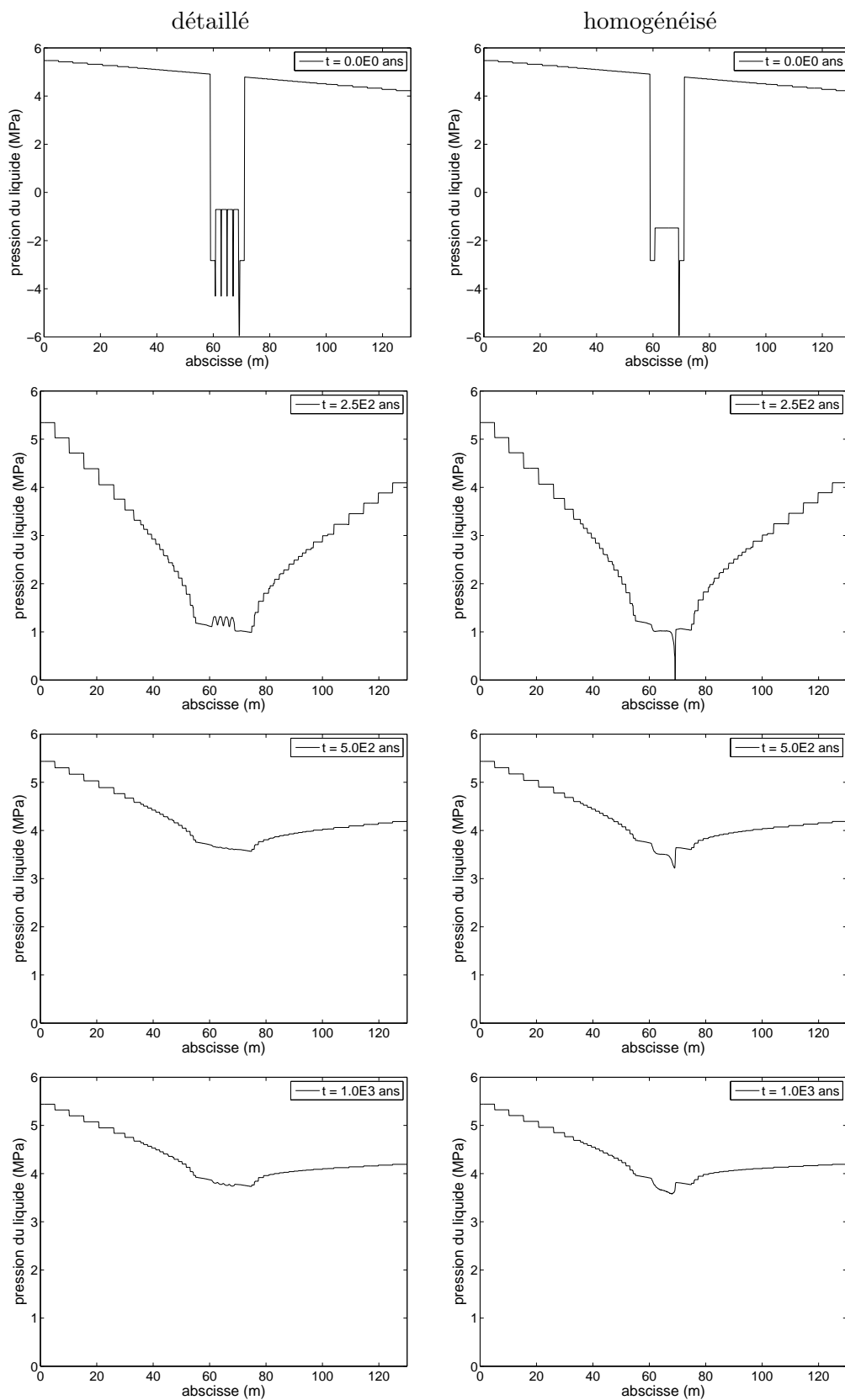
FIGURE 9.9 – Profils selon z de la pression du liquide en x = 130 m aux différents temps d’observation de 0 ans à 1000 ans Comparaison entre le problème détaillé (à gauche) et le problème homogénéisé (à droite).
