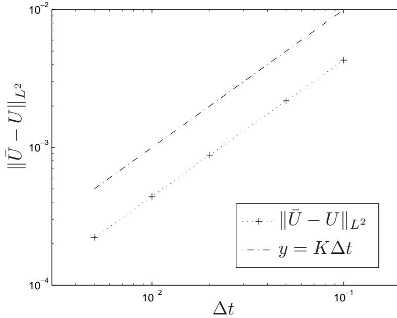
FIGURE 3.2 – Évolution de \|U - \bar{U}\|_{L^2} vs. \Delta t
