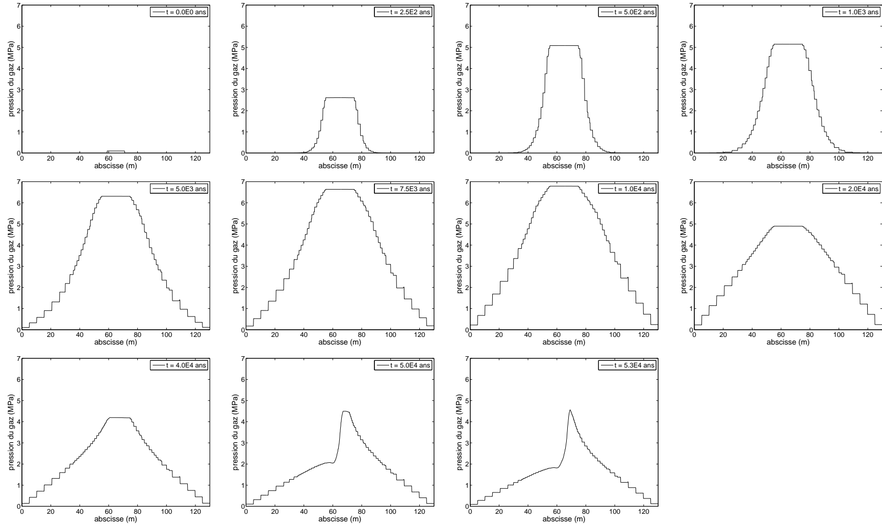
FIGURE 8.6 – Profils de la pression du gaz en x = 103 \text{ m} aux différents temps d’observation. L’abscisse 0 \text{ m} correspond au bas du domaine ( z = 0 \text{ m} ) et l’abscisse 130 \text{ m} correspond au haut du domaine ( z = 130 \text{ m} ).
