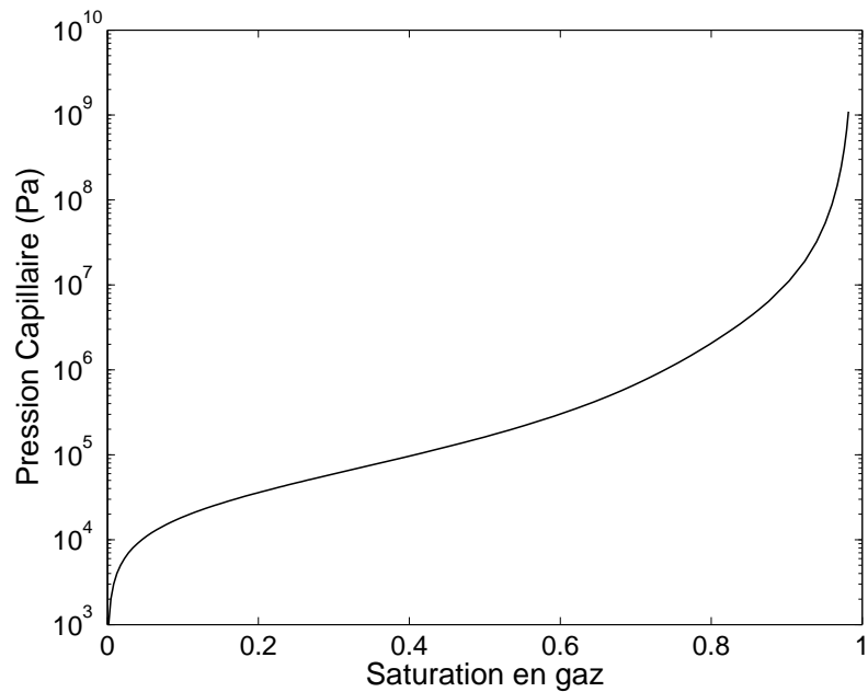
FIGURE 9.2 – Loi de pression capillaire effective de la zone de colis homogénéisée
