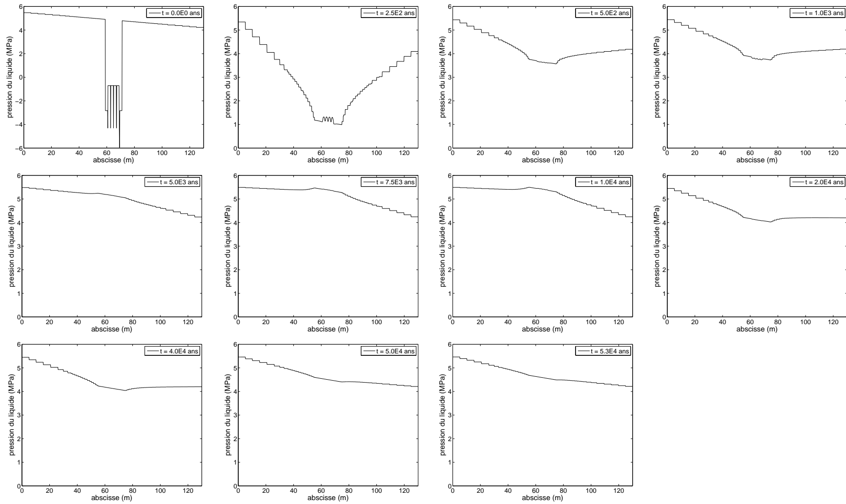
FIGURE 8.5 – Profils de la pression du liquide en x = 103 \text{ m} aux différents temps d'observation. L'abscisse 0 \text{ m} correspond au bas du domaine ( z = 0 \text{ m} ) et l'abscisse 130 \text{ m} correspond au haut du domaine ( z = 130 \text{ m} ).
