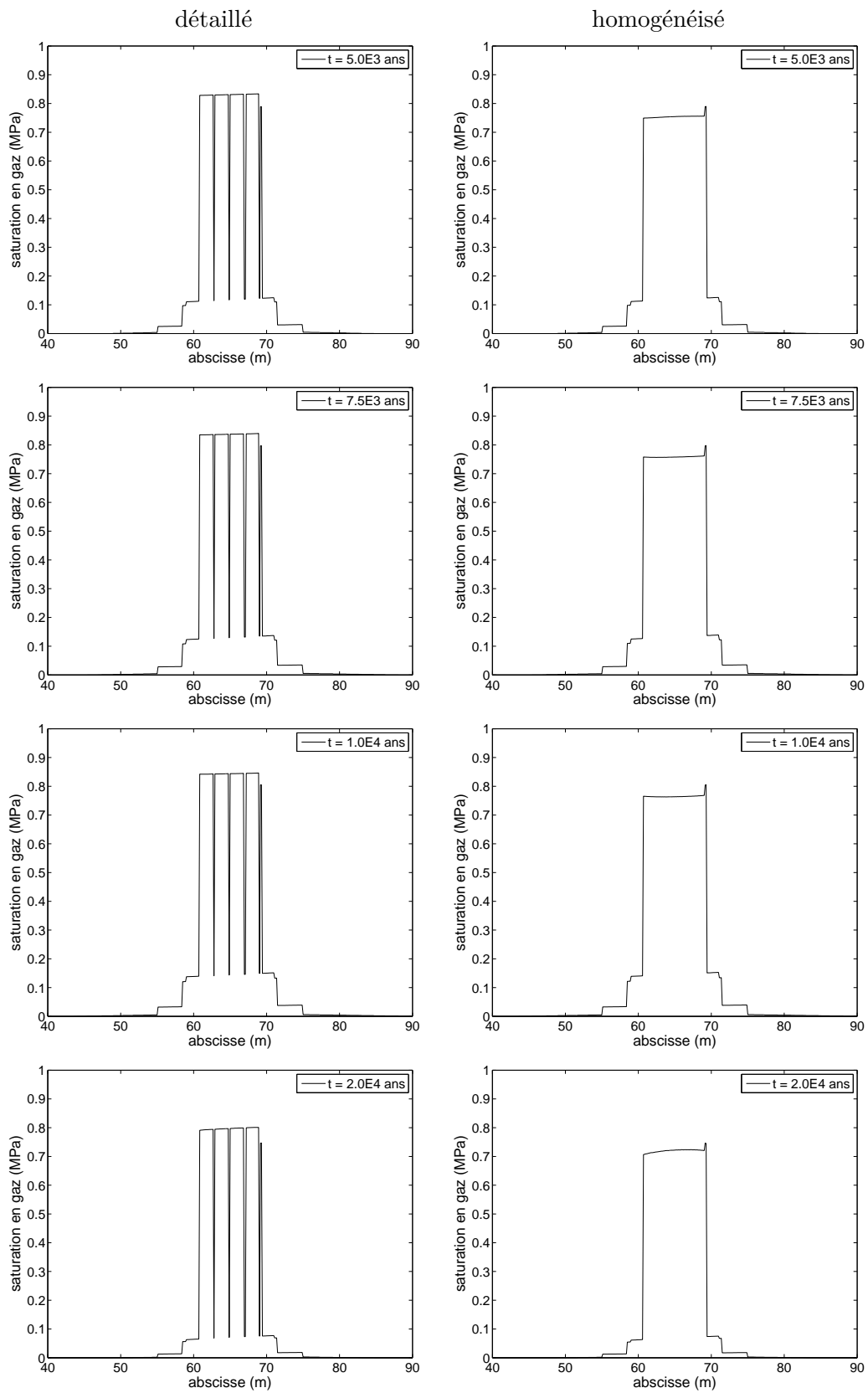
FIGURE 9.14 – Profils selon z de la saturation en gaz en x = 130 m aux différents temps d'observation de 5000 ans à 20000 ans. Comparaison entre le problème détaillé (à gauche) et le problème homogénéisé (à droite).
