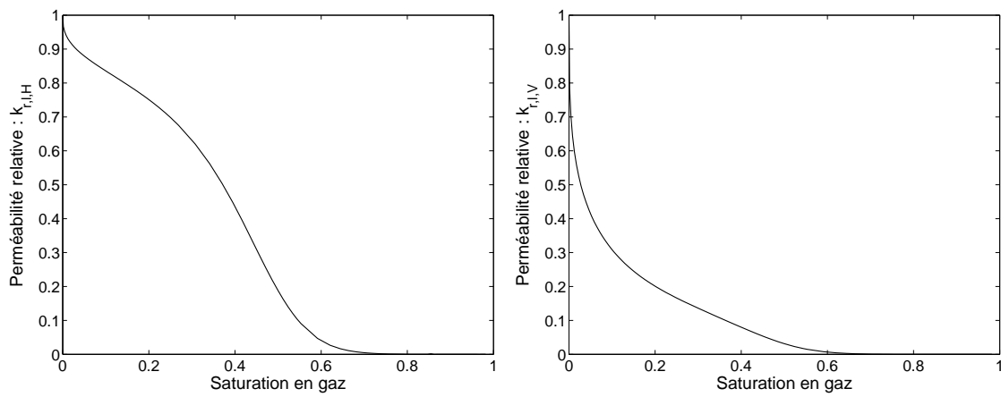
FIGURE 9.3 – Loi de perméabilité relative effective de la phase liquide de la zone de colis homogénéisée
