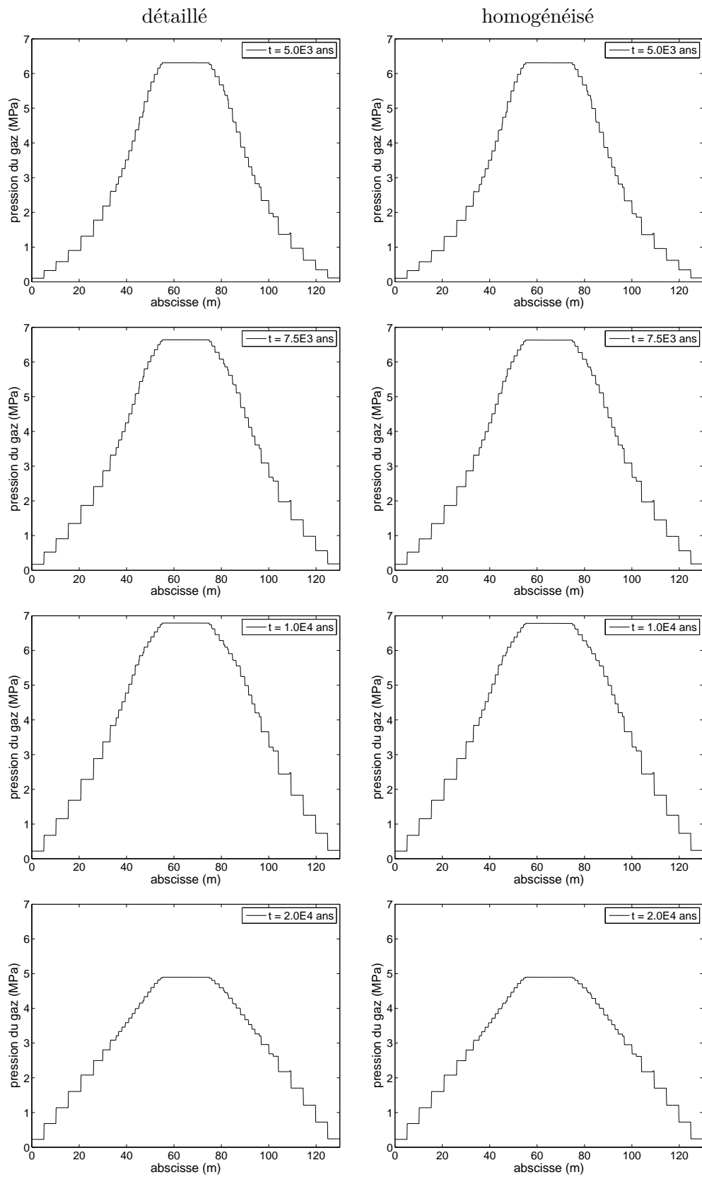
FIGURE 9.12 – Profils selon z de la pression du gaz en x = 130 m aux différents temps d'observation de 5000 ans à 20000 ans. Comparaison entre le problème détaillé (à gauche) et le problème homogénéisé (à droite).
