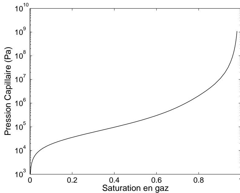
FIGURE 9.2 – Loi de pression capillaire effective de la zone de colis homogénéisée
