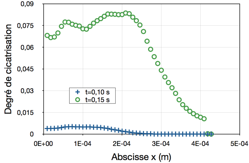
FIG. IV.14: Degré de cicatrisation de l'interface.
