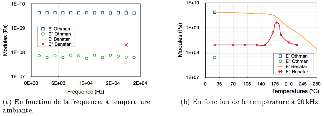
FIG. F-7: Modules viscoélastiques à haute fréquence.
