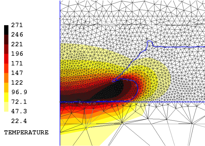
FIG. IV.6: Champ de température à l'instant t = 0,1 s.
