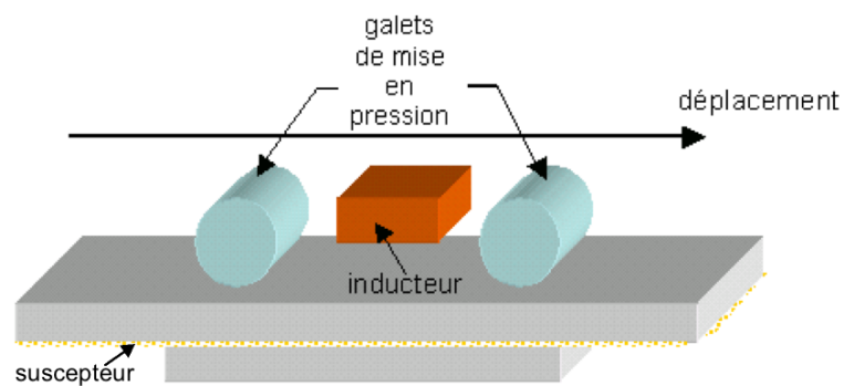
FIG. I.8: Principe du soudage par induction
