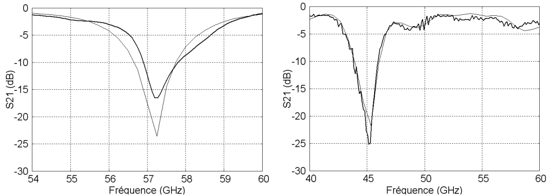
FIG. 1.7 – Module de S21 pour le substrat TPX à 60 GHz (gauche), Module de S21 pour le substrat Duroid 6006 à 45 GHz (droite).
