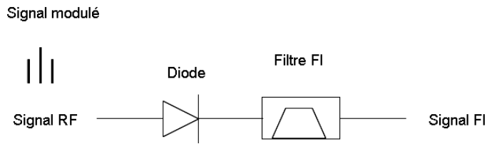
FIG. 2.14 – Démodulation par détecteur simple diode
