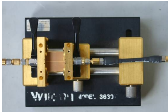
FIG. 1.6 – Technique de mesure avec Cellule Wiltron.
