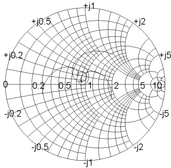
FIG. 1.33 – Impédance d'entrée de la pastille à polarisation circulaire à 60 GHz : Mesure (gras) et simulation (fin)
