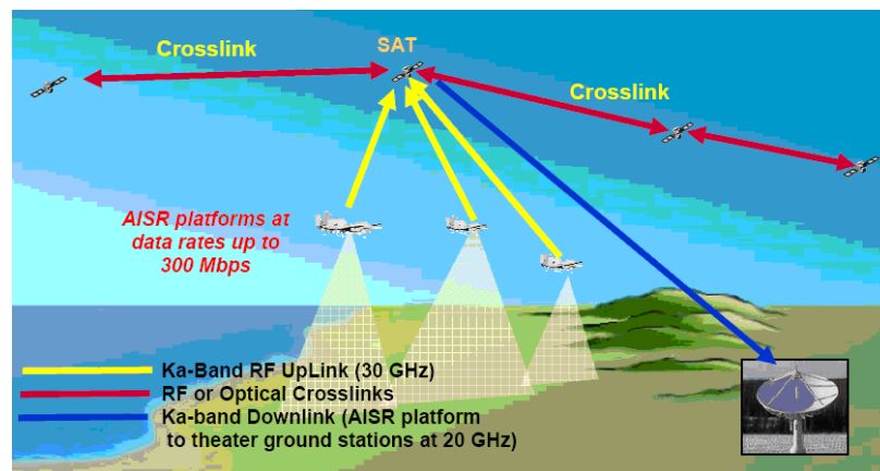
FIG. 5.5 – Application liaison de données haut débit entre un drone et un satellite géostationnaire en bande Ka.
