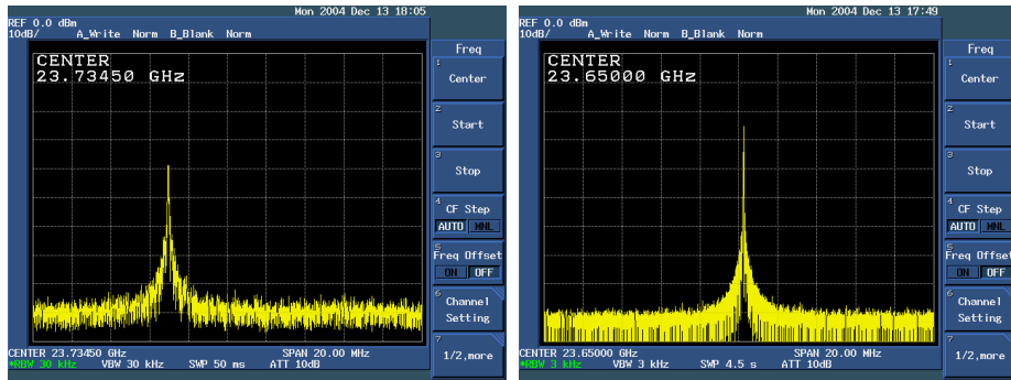
FIG. 2.11 – Spectres des antennes dites oscillatrices : Pastille élémentaire (gauche), réseau de 16 pastilles (droite).
