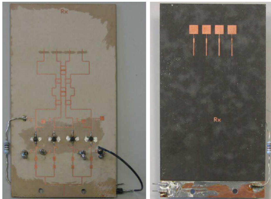
FIG. 4.13 – Maquette active de l'antenne multifaisceaux à 24 GHz.
