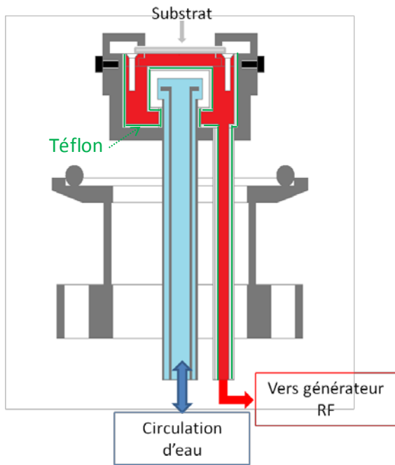
Figure 2-5 : Schéma et photographie de l'électrode porte-échantillon refroidie par un circuit d'eau
