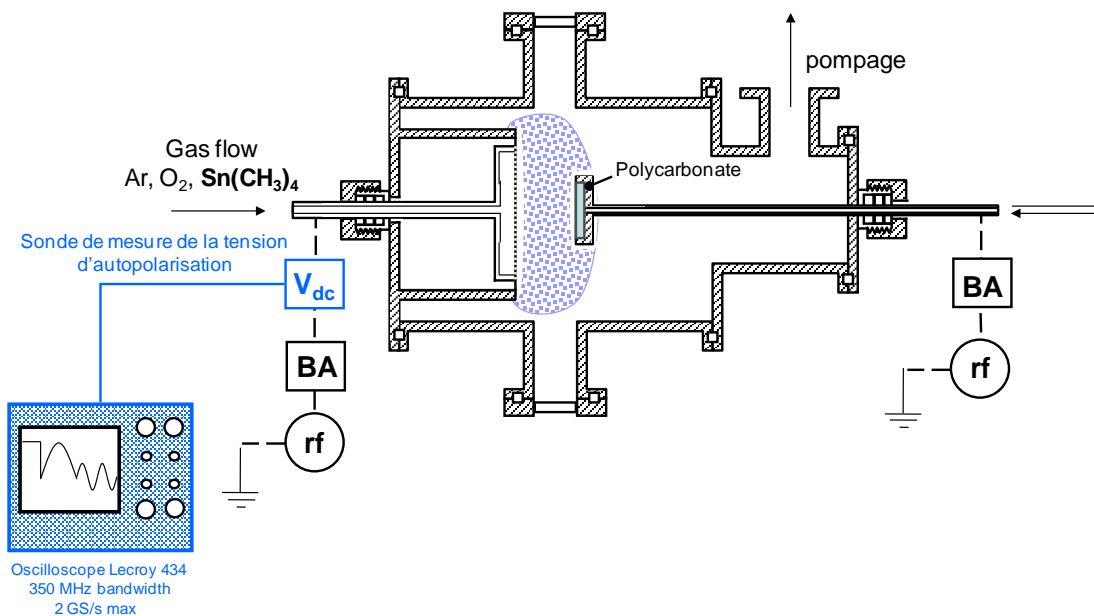
Figure 2-8: Schéma du montage de la sonde de tension pour le suivi de la V_{DC} de l'électrode douche
