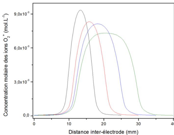
Figure 3-9: Variation de la concentration molaire d'ion \text{O}_2^+ en fonction de la distance inter-électrode, dans un plasma Ar/ \text{O}_2
