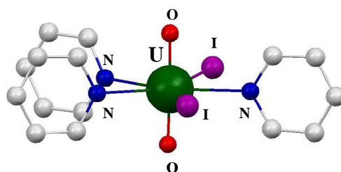
Figure I.21 : Structure du complexe [\text{UO}_2\text{I}_2\text{py}_3] . 152 Les atomes d'hydrogènes ont été omis pour des raisons de clarté.
