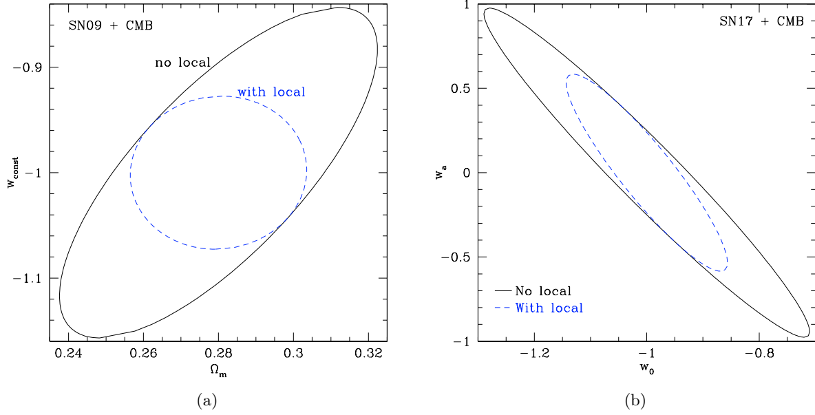
FIG. 1.8: Contours de confiance pour (a) (w, \Omega_m) à partir d'un échantillon de 500 SNe Ia grand z uniformément distribuées entre 0.2 < z < 0.9 et (b) (w_a, w_0) pour un échantillon de 2000 SNe Ia distribuées entre 0.2 < z < 1.7 , avec, et sans un échantillon de 300 SNe Ia à faible z centré sur z = 0.05 .
