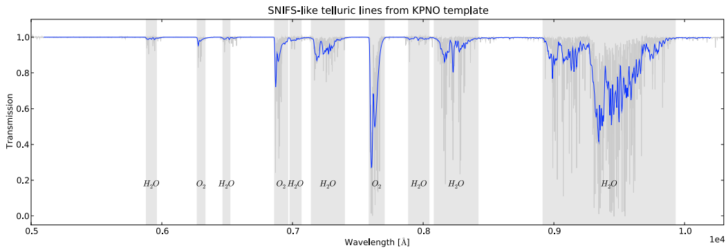
FIG. 9.7: Principales raies telluriques (voir table 9.1) à la résolution SNIFS (en bleu) obtenues à partir du spectre haute résolution (en gris) observé au Keat Peak National Observatory (AZ) (Wallace and Livingston 2003).
