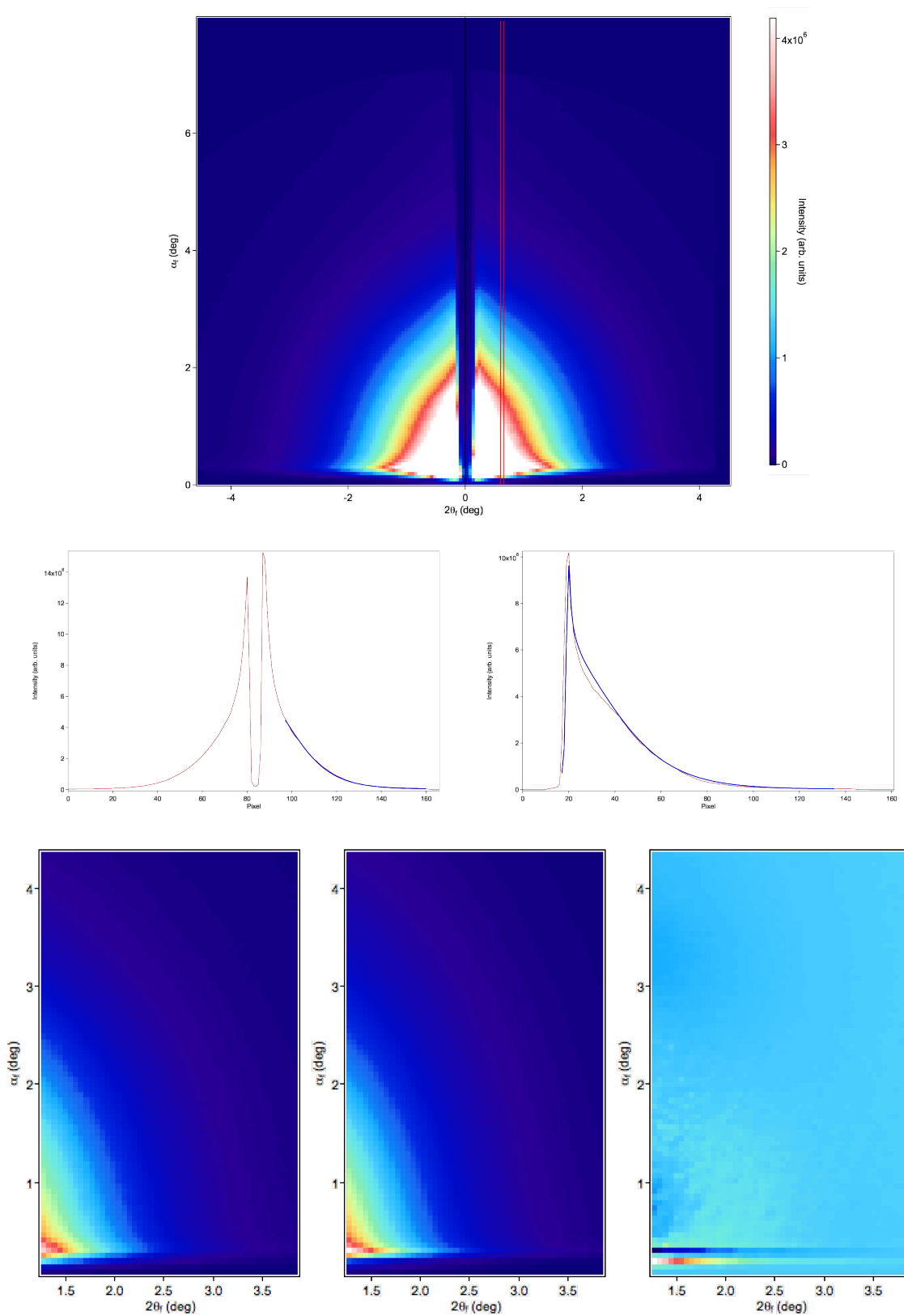
FIGURE 7.10: En haut : spectre de GISAXS d'un échantillon \text{NTCoPt}_{\text{CT}}^{\text{NT}} . Au milieu, ajustement des profils q_{\perp} et q_{\parallel} . En bas ajustement à deux dimensions (de gauche à droite : image expérimentale, ajustement et résidu).
