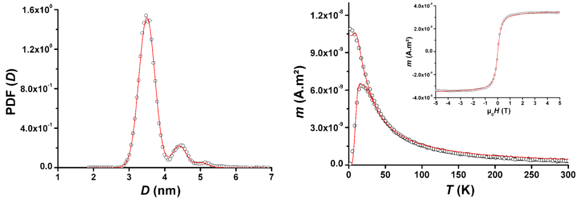
FIGURE 10.5: À gauche distribution des tailles au sein de l'échantillon ^{\text{TM}}\text{Co}_{\text{Cr}}^{\text{CrPt}} . À droite courbes ZFC FC et cycle à 300 K d'un échantillon de cobalt trié en taille avec une taille moyenne de 3,5 nm et une dispersion de 0,22 nm ^{\text{TM}}\text{Co}_{\text{Cr}}^{\text{CrPt}} .
