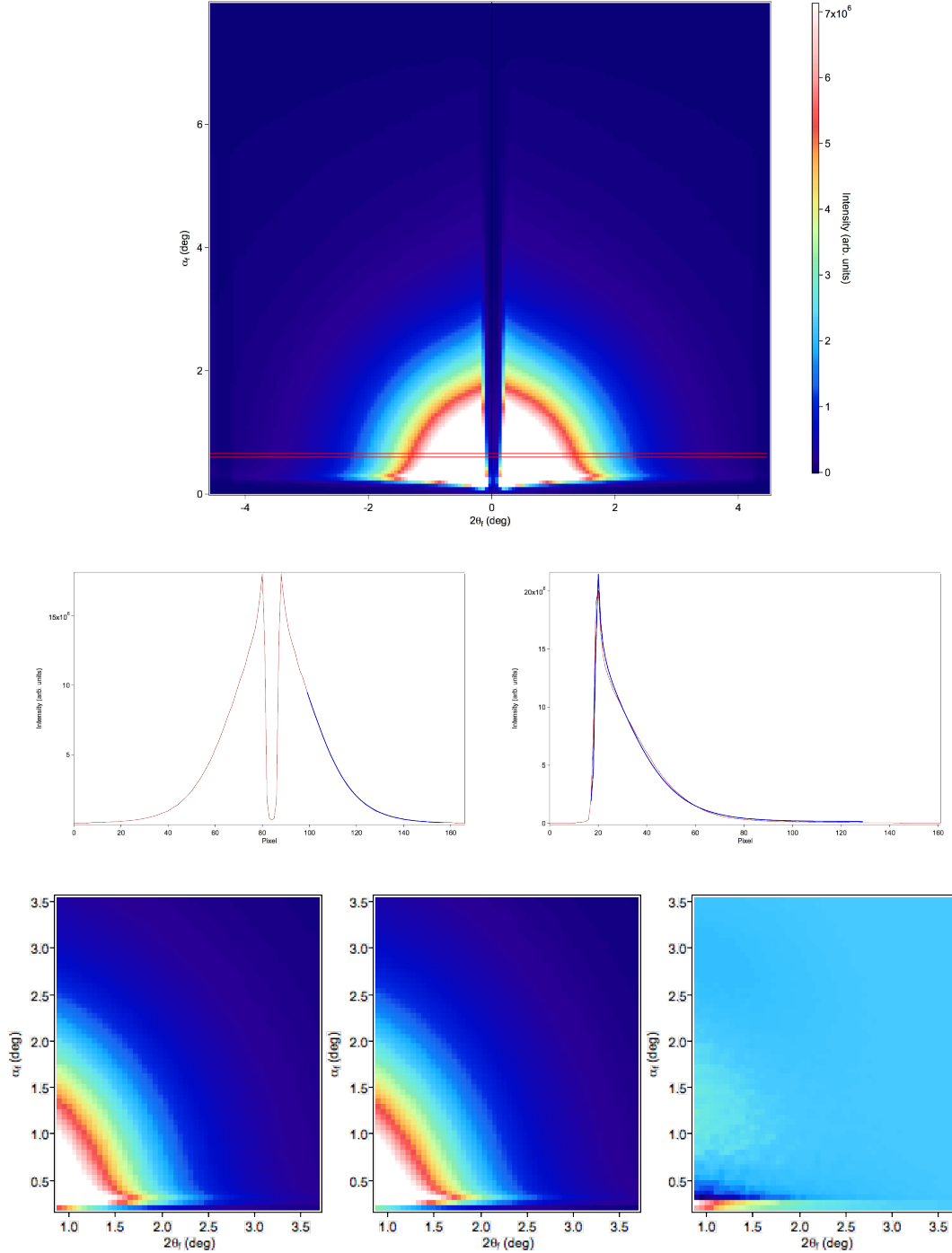
FIGURE 7.11: En haut : spectre de GISAXS d'un échantillon ^{NT}CoPt_{CT}^{cuit} . Au milieu, ajustement des profils q_{\perp} et q_{\parallel} . En bas ajustement à deux dimensions (de gauche à droite : image expérimentale, ajustement et résidu).
