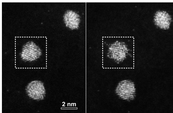
FIGURE 8.2: Image HAADF atomique de nanoparticules CoPt. Le cadre en pointillés repère une zone ayant servi à la mise au point de l'image pendant quelques secondes : on note le dommage important causé par le faisceau intense à la nanoparticule (microscope Titan 300 kV, Minatec-Grenoble).
