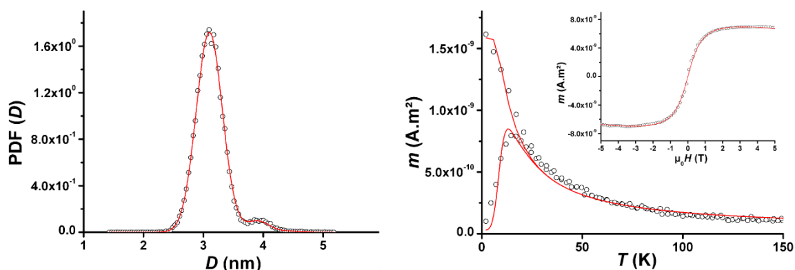
FIGURE 10.7: À gauche distribution des tailles au sein de l'échantillon {}^{\text{TM}}\text{CoPt}_{\text{Ct}}^{\text{cru}} . À droite, « triple fit » sur un échantillon de CoPt {}^{\text{TM}}\text{CoPt}_{\text{Ct}}^{\text{cru}} avec la prise en compte d'une anisotropie de surface.
