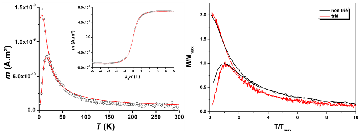
FIGURE 10.4: Á gauche échantillon ^{TM}CoPt_{Ct}^{cru} , avec courbes ZFC - FC - cycle haute température ; Á droite comparaison des ZFC - FC normalisées entre échantillon non trié : ^{NT}CoPt_{Ct}^{cru} et échantillon triés en taille avec une taille moyenne de 3 nm et une dispersion de 0,2 nm : ^{TM}CoPt_{Ct}^{cru} .
