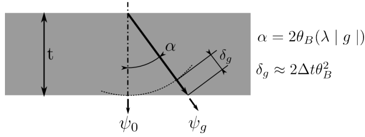
FIGURE 3.7: Description du déphasage de propagation entre deux couches dans la méthode multislice.
