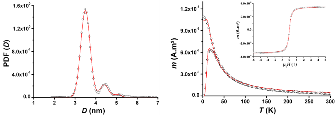
FIGURE 10.5: À gauche distribution des tailles au sein de l'échantillon ^{\text{TM}}\text{Co}_{\text{Ct}}^{\text{cru}} . À droite courbes ZFC FC et cycle à 300 K d'un échantillon de cobalt trié en taille avec une taille moyenne de 3,5 nm et une dispersion de 0,22 nm ^{\text{TM}}\text{Co}_{\text{Ct}}^{\text{cru}} .
