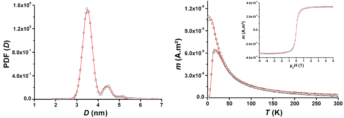
FIGURE 10.5: À gauche distribution des tailles au sein de l'échantillon ^{\text{TM}}\text{Co}_{\text{CrPt}}^{\text{cru}} . À droite courbes ZFC FC et cycle à 300 K d'un échantillon de cobalt trié en taille avec une taille moyenne de 3,5 nm et une dispersion de 0,22 nm ^{\text{TM}}\text{Co}_{\text{CrPt}}^{\text{cru}} .
