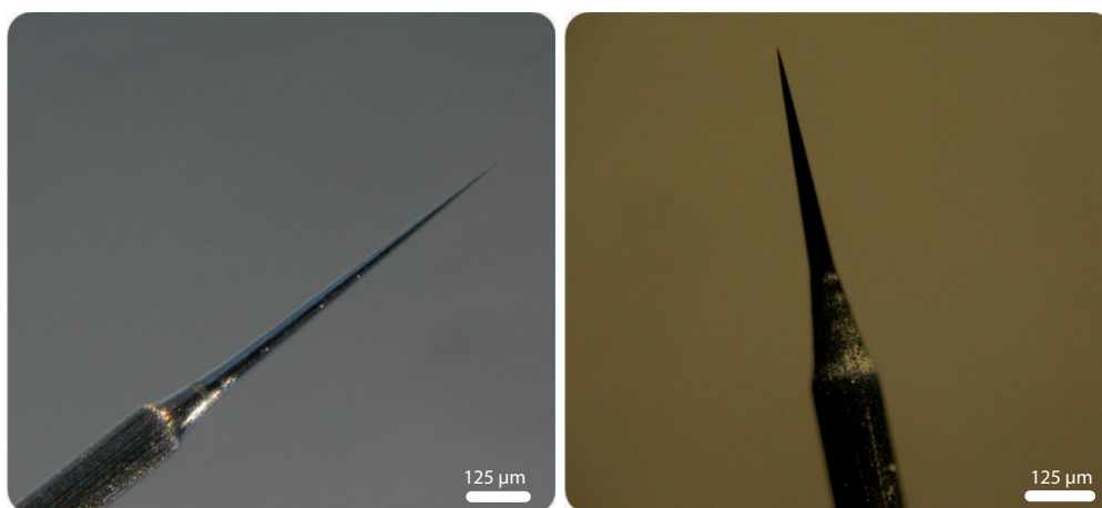
Figure 3.8 – Images de deux pointes métalliques de Tungstène obtenues par polissage électrolytique. En faisant varier la longueur immergée du filament de W dans la solution électrolytique de NaOH, la nature et la valeur de la tension appliquée pendant l'électrolyse, on arrive à contrôler l'affinage de la pointe ainsi créée.
