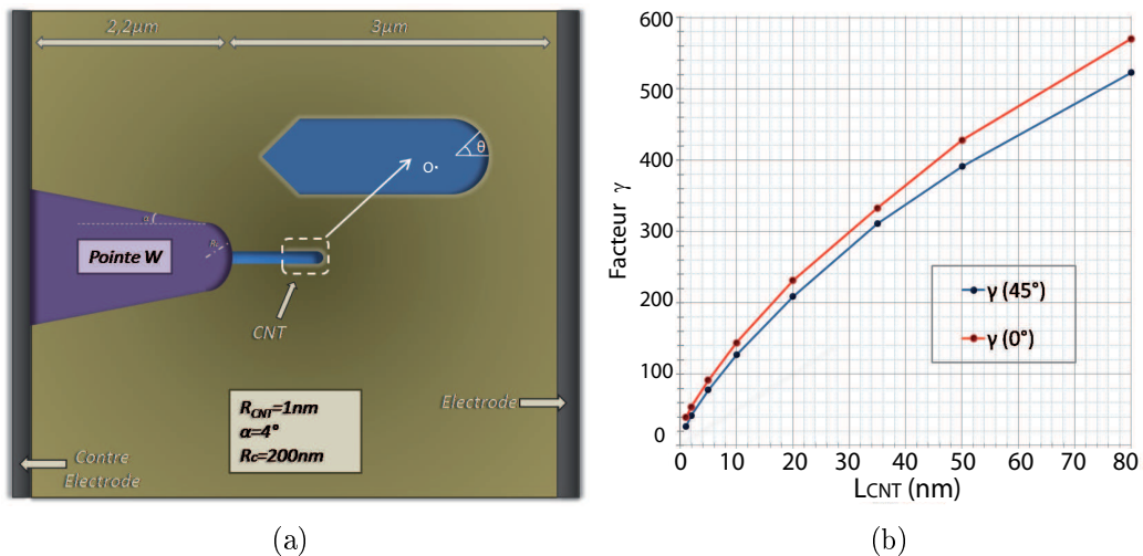
Figure 2.13 – a) Schéma représentatif d'un nanotube situé dans l'axe d'une pointe de W affînée. L'angle \theta représenté sur la figure est défini comme étant l'angle entre l'axe principal du nanotube et la droite qui coupe un point de la surface hémisphérique du nanotube. Une contre électrode a été placée au niveau de la base du substrat ainsi qu'une autre électrode à 3 \mu\text{m} de l'extrémité de la pointe de W . b) Evolution du facteur \gamma à \theta = 0^\circ et à \theta = 45^\circ en fonction de la longueur du nanotube.
