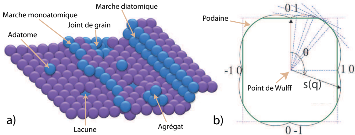
Figure 4.2 – a) Schéma montrant quelques défauts (adatomes, lacunes, joints de grain, etc) pouvant apparaître sur une surface à l'échelle atomique. b) Schéma de construction classique de "Wulff" déterminant la forme d'un cristal à l'équilibre.
