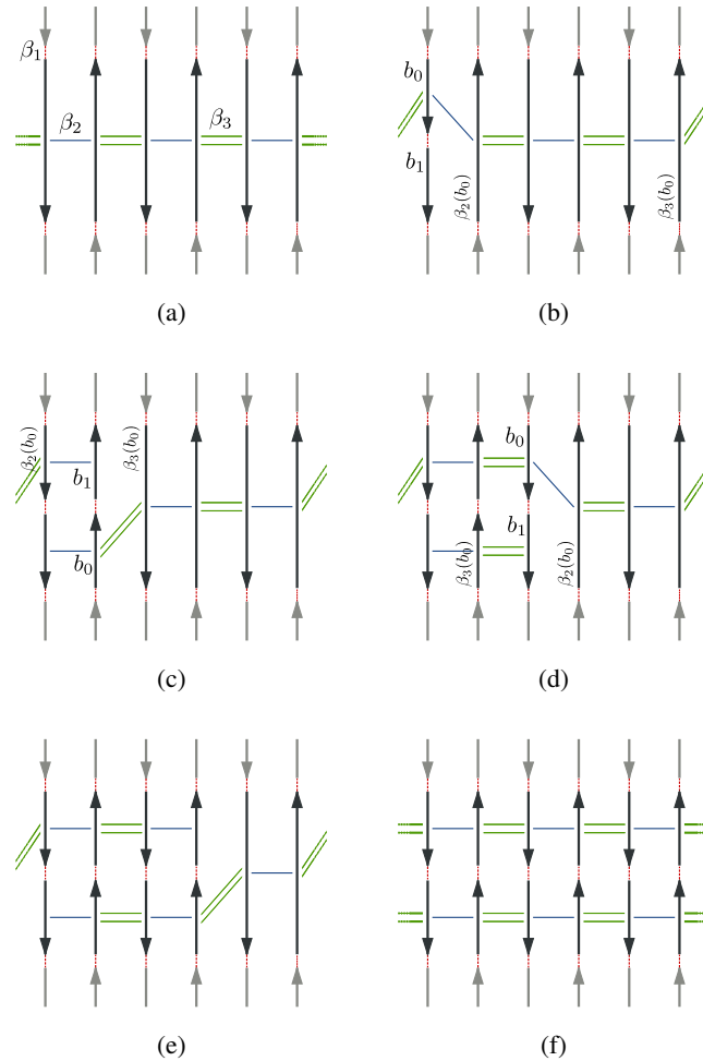
FIG. 5.1: Illustration de l'insertion d'un sommet sur une arête composée de six brins. (a) Configuration initiale avec six brins représentant l'arête incidente à b . La légende des relations entre les brins est donnée sur la figure. Les brins en gris clair sont les brins des arêtes incidentes. (b) Insertion de b_1 entre b_0 et \beta_1(b_0) . Les brins \beta_2(b_0) et \beta_3(b_0) n'ont pas encore été traités : nous ne modifions pas les relations \beta_2 ou \beta_3 . (c) Lors du traitement du brin suivant, le brin \beta_2(b_0) a été traité. Nous modifions donc les relations \beta_2 pour rendre conforme l'orbite des deux arêtes en cours de création. (d) Lors du traitement du brin suivant, le brin \beta_3(b_0) a été traité. Nous modifions alors les relations \beta_3 pour être conforme aux orbites des deux nouvelles arêtes. (e) Traitement du brin suivant. (f) Résultat une fois que tous les brins ont été traités.
