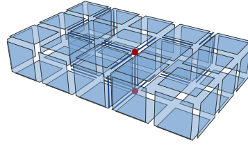
FIG. 2.11: Matrice intervoxel représentant le plongement de la carte de niveau 3 (Figure 2.7) avec des éléments unitaires.
