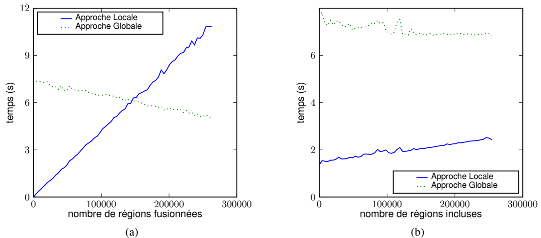
FIG. 4.2: Comparaison de l'approche locale et globale de la fusion en fonction (a) du nombre de régions à fusionner dans une seule région résultante. (b) du nombre de régions imbriquées dans la région résultante.
