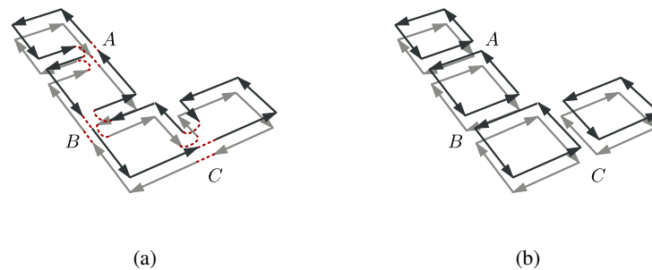
FIG. 5.10: Exemple de fermeture des faces élémentaires lors de l'éclatement d'une face. (a) Configuration initiale, les sommets étiquetés par A , B et C sont modifiés par l'Algorithme 19 afin de fermer les faces élémentaires. (b) Résultat de l'opération de fermeture des faces élémentaires. La face initiale est remplacée par quatre faces élémentaires.
