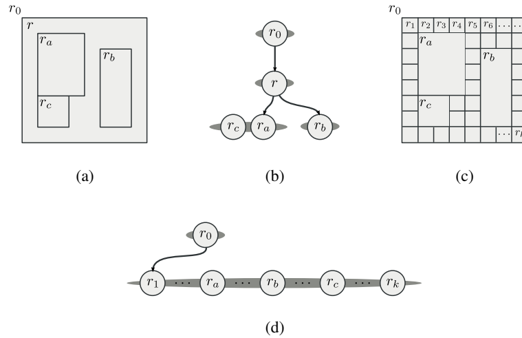
FIG. 5.17: Mise à jour de l'arbre d'imbrication des régions dans le cas de l'éclatement d'une région. (a) Partition initiale de l'image. (b) Arbre d'imbrication initial. (c) Résultat de l'éclatement de la région r dans la partition. (d) Résultat de l'éclatement de la région r dans l'arbre d'imbrication.
