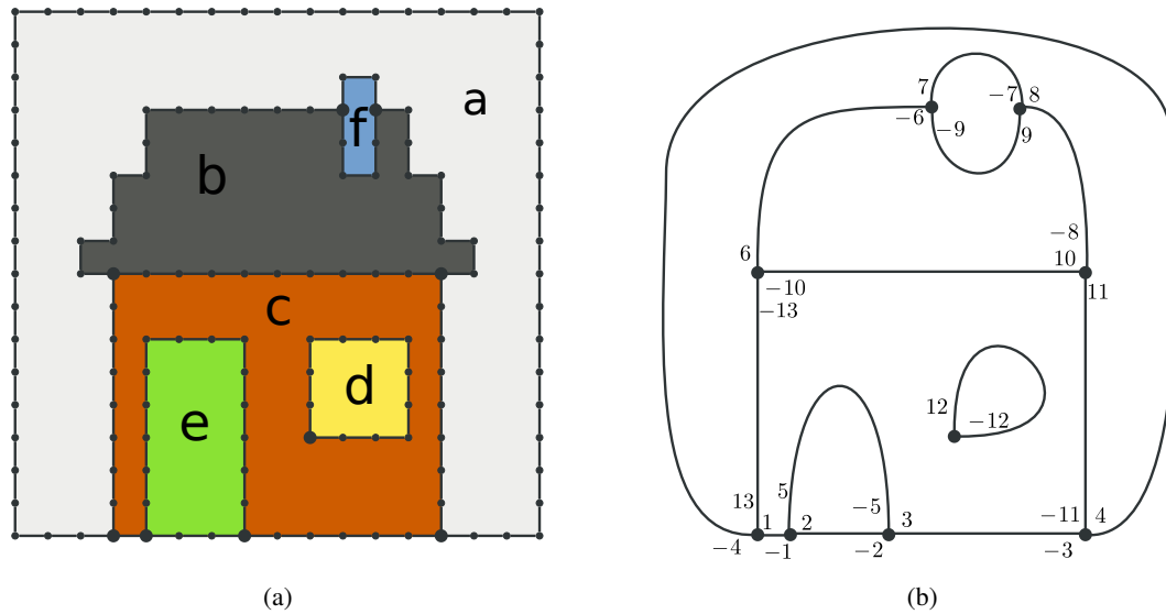
FIG. 1.23: Exemple d'une carte discrète représentant une image : (a) frontières en interpixel de la partition de l'image ; (b) carte planaire représentant la carte des frontières de la partition.
