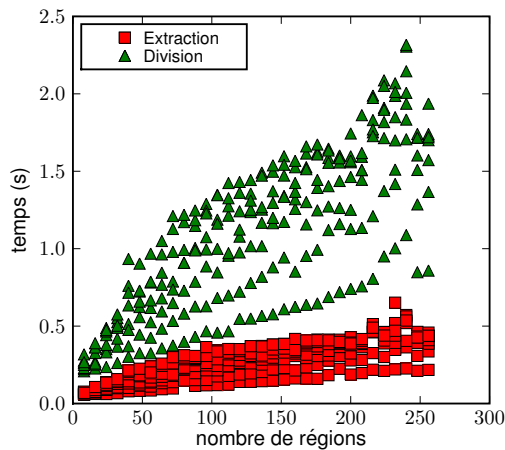
FIG. 5.22: Comparaison de l'extraction avec l'opération de division dans le cas d'images aléatoires simples.
