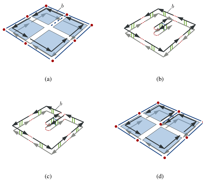
FIG. 5.6: Insertion d'une arête pendante dans une face. (a) Situation initiale de la face. (b) Quatre nouveaux brins sont ajoutés et cousus entre eux pour former une arête pendante. (c) Les brins sont reliés au sommet incident à b . (d) Le lignel et le pointel qui correspondent à l'arête et le sommet pendant sont allumés.
