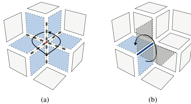
FIG. 5.7: Ombrelles dans la matrice intervoxel. Les éléments intervoxels représentés en pointillés sont les éléments de l'ombrelle. Les flèches signifient la permutation. (a) Les six lignels et les six surfels appartenant à l'ombrelle du pointel dessiné. (b) Les quatre surfels appartenant à l'ombrelle du lignel dessiné.
