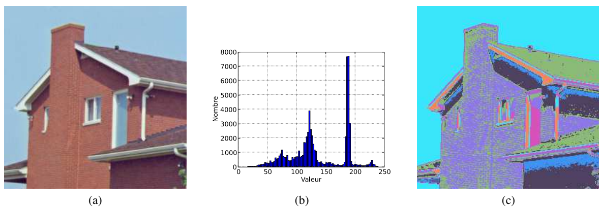
FIG. 3.2: Exemple de regroupement des valeurs des pixels d'une image 2D : (a) image originale en 256 niveaux de gris ; (b) histogramme de l'image ; (c) image étiquetée correspondant au regroupement des pixels d'après l'histogramme en 8 classes.
