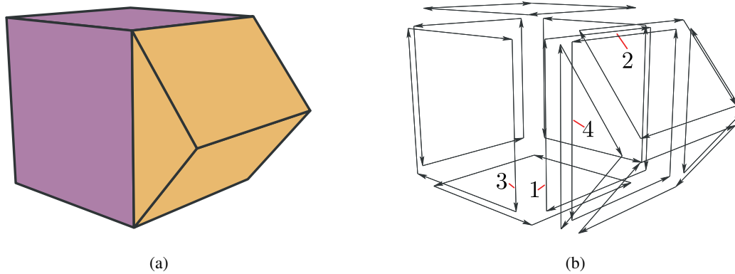
FIG. 1.18: Exemple de carte combinatoire en dimension 3 : (a) un objet composé de deux volumes, un cube et un prisme ; (b) carte combinatoire représentant l'objet. Les brins sont représentés par des flèches indiquant la relation \beta_1 . Les involutions \beta_2 et \beta_3 sont implicitement données par la géométrie utilisée dans la représentation. Deux brins proches incidents à la même face mais dans des volumes différents sont reliés par \beta_3 (par exemple \beta_3(1) = 4 ). Deux brins proches incidents au même volume mais situés dans des faces différentes sont liés par \beta_2 (par exemple \beta_2(1) = 3 ). Deux brins qui se suivent dans la même face et le même volume sont liés par \beta_1 , la flèche donnant le sens de la permutation (par exemple \beta_1(1) = 2 et \beta_0(2) = 1 ).
