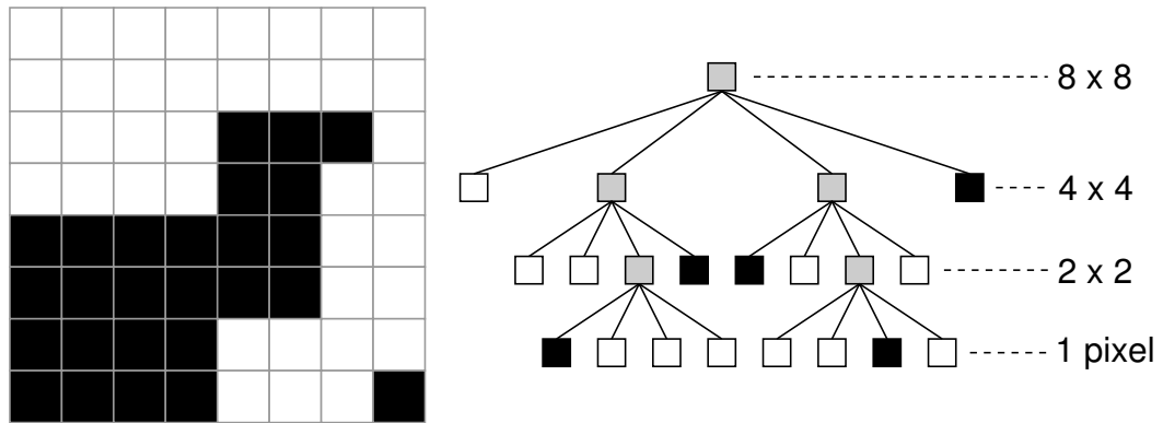
FIG. 1.13: Exemple de quadtree représentant une image binaire 8 \times 8 pixels. Les nœuds gris dans l'arbre représentent les régions non homogènes qui sont alors subdivisées en quatre sous-régions. Les feuilles de l'arbre représentent les régions homogènes de l'image.
