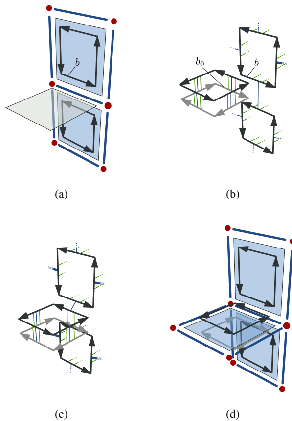
FIG. 5.13: Insertion d'une face élémentaire pendante dans un volume. (a) Configuration initiale avec un brin b incident à une arête élémentaire et un surfel s incident appartenant au même volume que b et qui n'est pas allumé. (b) Ajout des huit brins représentant la face élémentaire pendante. Le brin b_0 est plongé avec le même lignel et le même pointel que le brin b . (c) Couture des brins b , b_0 et de leurs images par \beta_2 de manière à connecter la face insérée avec l'arête incidente à b . (d) Allumage du plongement des cellules insérées.
