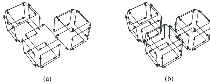
FIG. 5.16: Exemple d'éclatement d'un volume en volumes élémentaires. (a) Le bord du volume est éclaté en faces élémentaires. (b) Résultat de l'algorithme d'éclatement de volume, deux faces ont été insérées à l'intérieur du volume et reliées au bord du volume initial pour obtenir les trois volumes élémentaires issus de l'éclatement.
