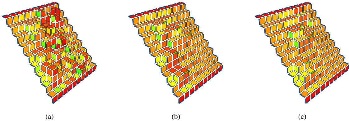
FIG. 6.8: Exemple de lissage d'une surface bruitée. (a) Surface bruitée originale. (b) Surface lissée en minimisant le nombre de surfels. (c) Surface lissée en minimisant l'estimateur d'aire.
