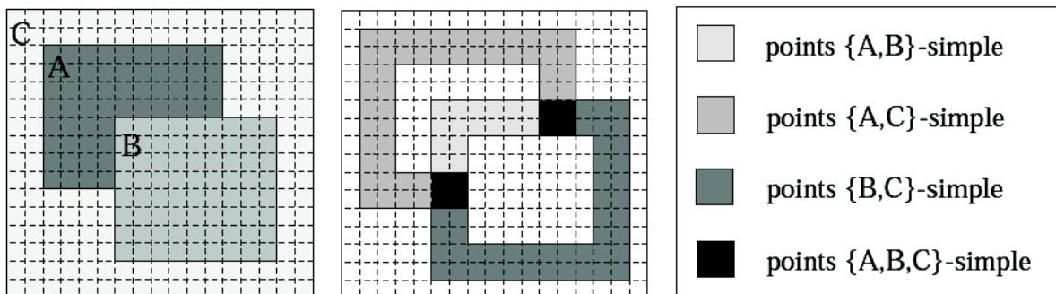
FIG. 3.11: Classification des points selon le fait qu'ils soient simples pour différentes régions dans une image 2D comportant trois régions. Les régions A et B sont considérées en 4-connexité et la région C est considérée en 8-connexité.
