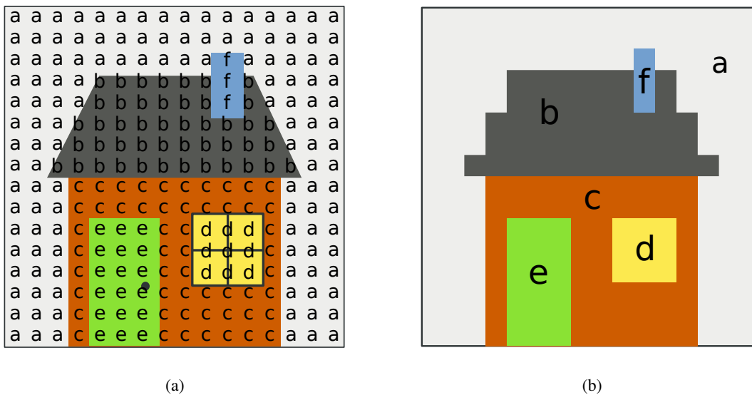
FIG. 1.6: Image 2D étiquetée : (a) image 2D où chaque pixel est associé à l'un des 6 étiquettes ; (b) image de couleurs représentant la partition de l'image 2D. Une couleur est choisie pour chaque étiquette et chaque pixel est dessiné avec la couleur de son étiquette.
