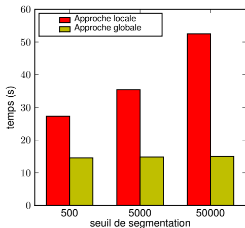
FIG. 4.6: Comparaison de l'approche locale et de l'approche globale lors d'un traitement automatisé impliquant un grand nombre de fusions de régions. Plus le seuil de segmentation est grand, plus le nombre de régions fusionnées est important.
