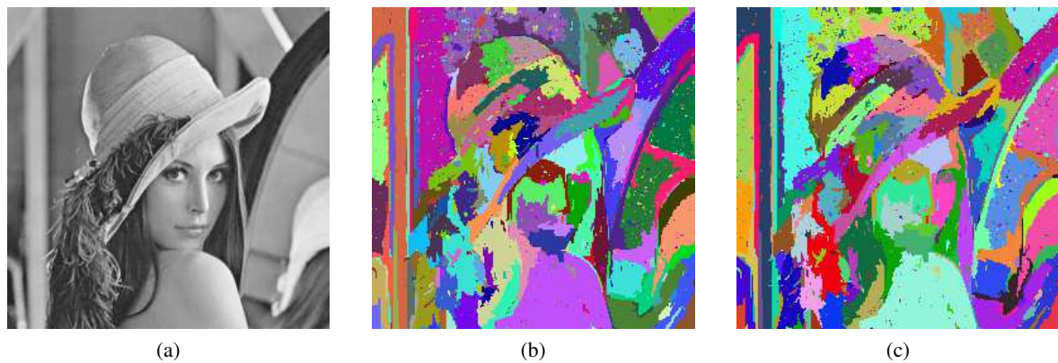
FIG. 7.1: Exemple de segmentation d'une image 2D (Lena) à l'aide d'un critère de contraste. Le seuil de segmentation k est fixé à 500 dans les deux applications. (a) Image originale ( 256 \times 256 ). (b) Segmentation à l'aide de l'algorithme original sur les graphes (4-connectivité). (c) Segmentation à l'aide de l'algorithme adapté sur les cartes topologiques. Les deux partitions obtenues sont identiques.
