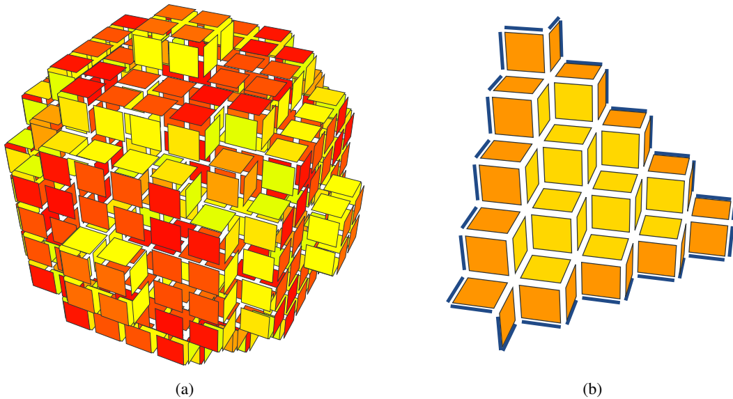
FIG. 6.7: Exemples d'estimation d'aire pour deux surfaces discrètes. L'échelle des couleurs indique la valeur de l'aire estimée pour chaque surfel. Elle va de vert (aire nulle : 0) à rouge (aire maximale : 1). (a) Pour une sphère de rayon 5, la mesure estimée est de 281,29 alors que la mesure théorique est de 314,15. (b) Pour un plan R2 dans un cube de 5 \times 5 \times 5 voxels, la mesure estimée est de 25,50 alors que la mesure théorique est de 21,65.
