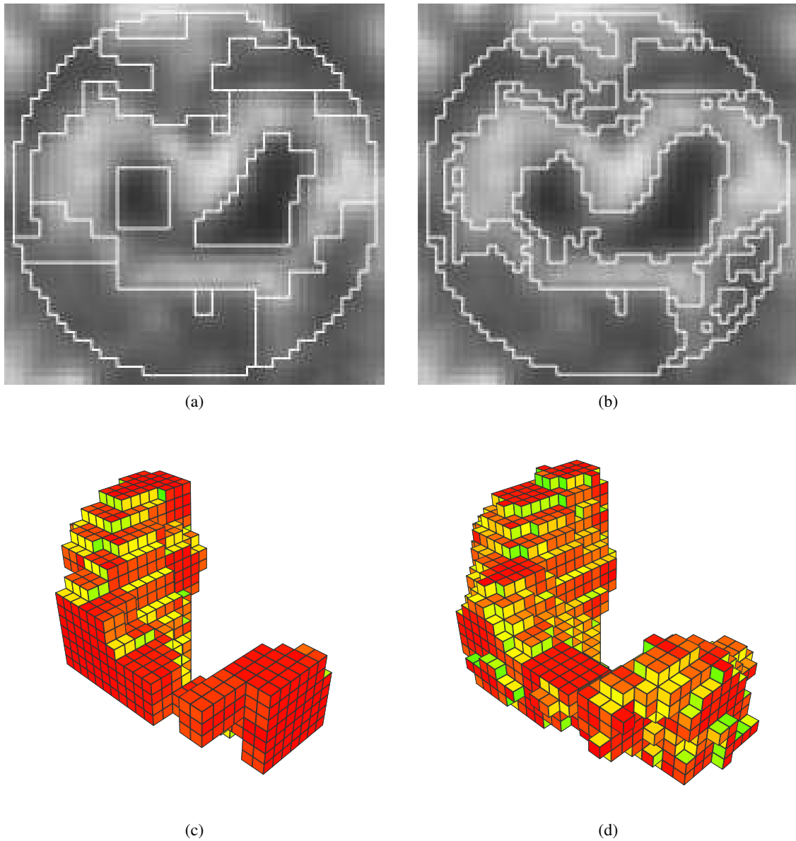
FIG. 6.13: Raffinement d'une partition sur une image médicale. (a) Coupe de l'image représentant la partition initiale. (b) Partition après déformation : nous observons que les formes sont globalement moins carrées. (c) Surface de la région hachurée avant la déformation : la forme est très cubique. Cette région contient 1293 voxels et sa surface est composée de 1192 surfels. (d) Surface de la région hachurée après la déformation : la forme est plus lisse. La région résultante est plus grosse, elle contient 1970 voxels et sa surface comprend 1716 surfels.
