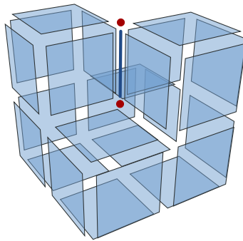
FIG. 2.10: Configuration où les deux pointels sont allumés alors qu'ils ne sont incidents qu'à un seul lignel. Les pointels représentent le plongement des sommets du bord de l'arête.
