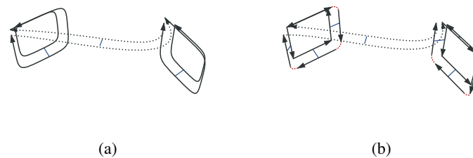
FIG. 5.4: Exemple d'éclatement des arêtes en arêtes élémentaires. (a) Trois arêtes appartenant à la surface d'un volume : il y a deux arêtes réelles et une arête fictive (dont les brins sont dessinés en pointillés). (b) Résultat de l'opération d'éclatement des arêtes : les arêtes réelles sont remplacées par des arêtes élémentaires, l'arête fictive n'est pas modifiée.
