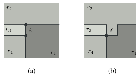
FIG. 3.12: Changement de la topologie de la partition sans changement de la topologie de chaque région. (a) Le basculement du pixel x de la région r_1 dans la région r_2 ne change pas la topologie d'après la définition des points simples de [Coi99]; (b) Un sommet et une arête disparaissent, faisant disparaître une relation d'adjacence entre la région r_1 et la région r_3 : il y a changement dans la topologie de la partition.
