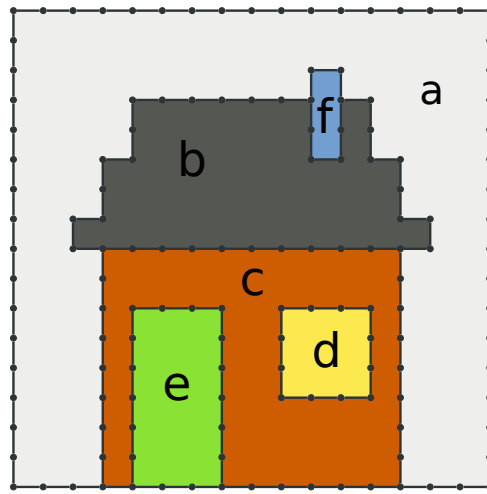
FIG. 1.12: Partition d'une image 2D représentée à l'aide de l'interpixel.
