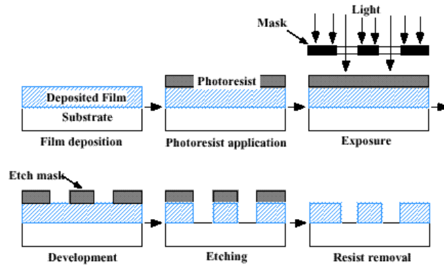
FIG. 3 – Traitement front-end .
