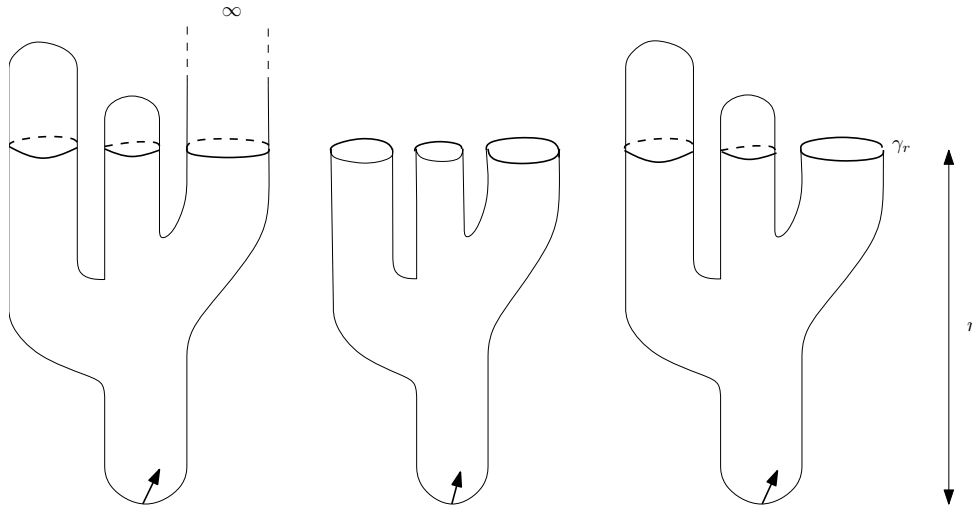
FIG. 1.8 – Une quadrangulation q vue de profil ainsi sa boule B_{\mathbf{Q},r}(q) et son enveloppe \hat{B}_{\mathbf{Q},r}(q) .
