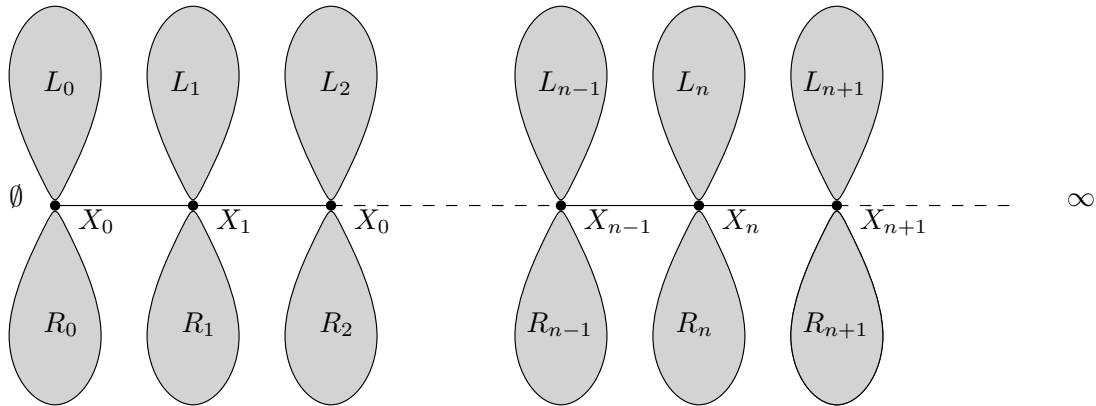
FIG. 1.9 – Exemple d'arbre de loi \mu .
